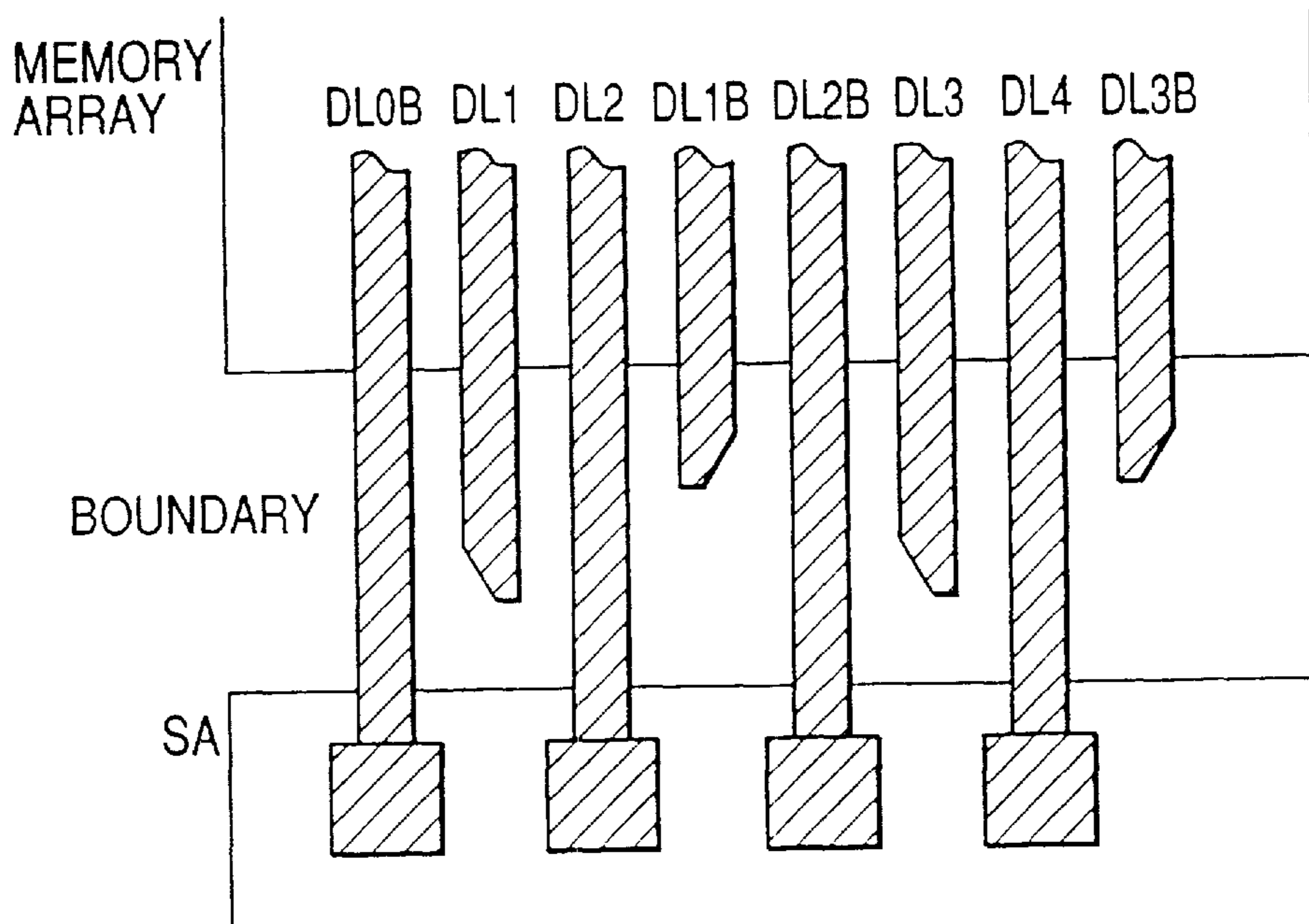
FIG. 12(b)
