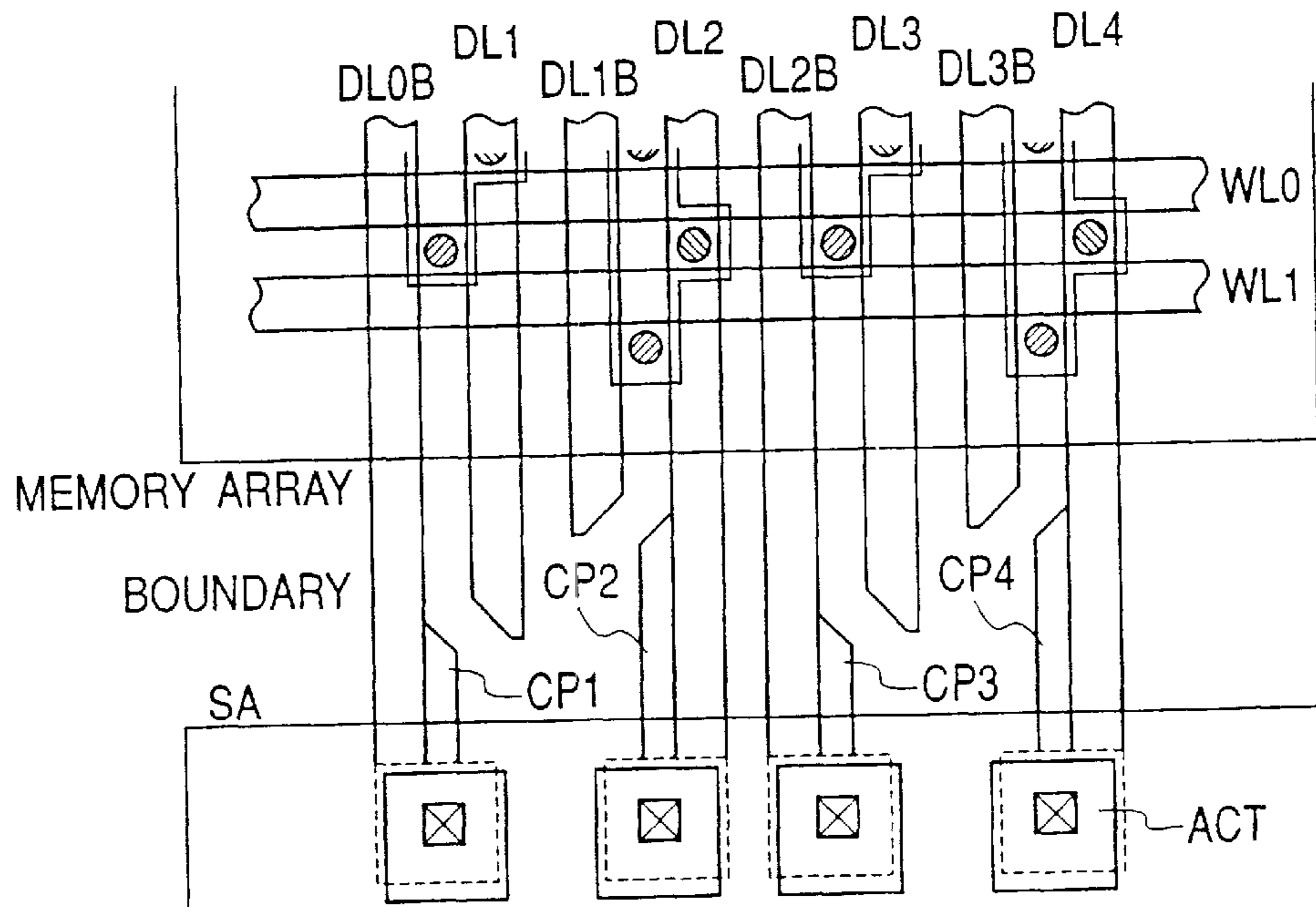
FIG. 6(b)
