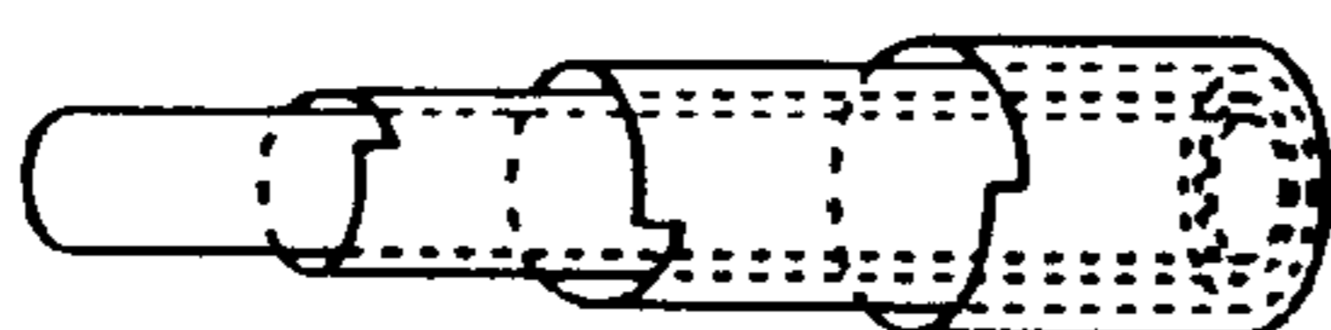
MWCNT (MULTI · WALL CARBON NANO · TUBE)
