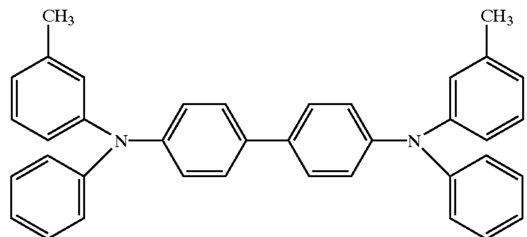
TPD:
