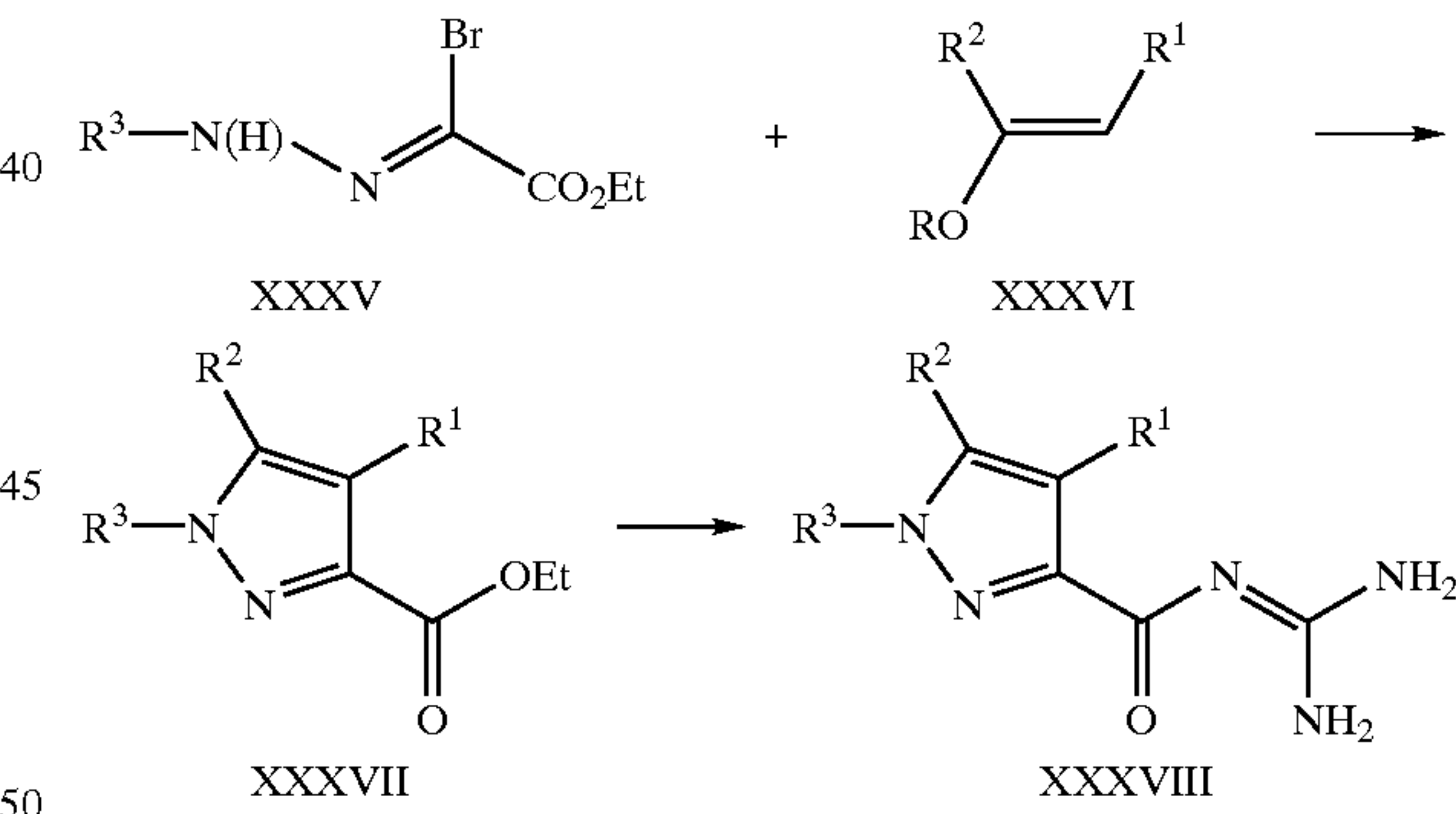
SCHEME VI
