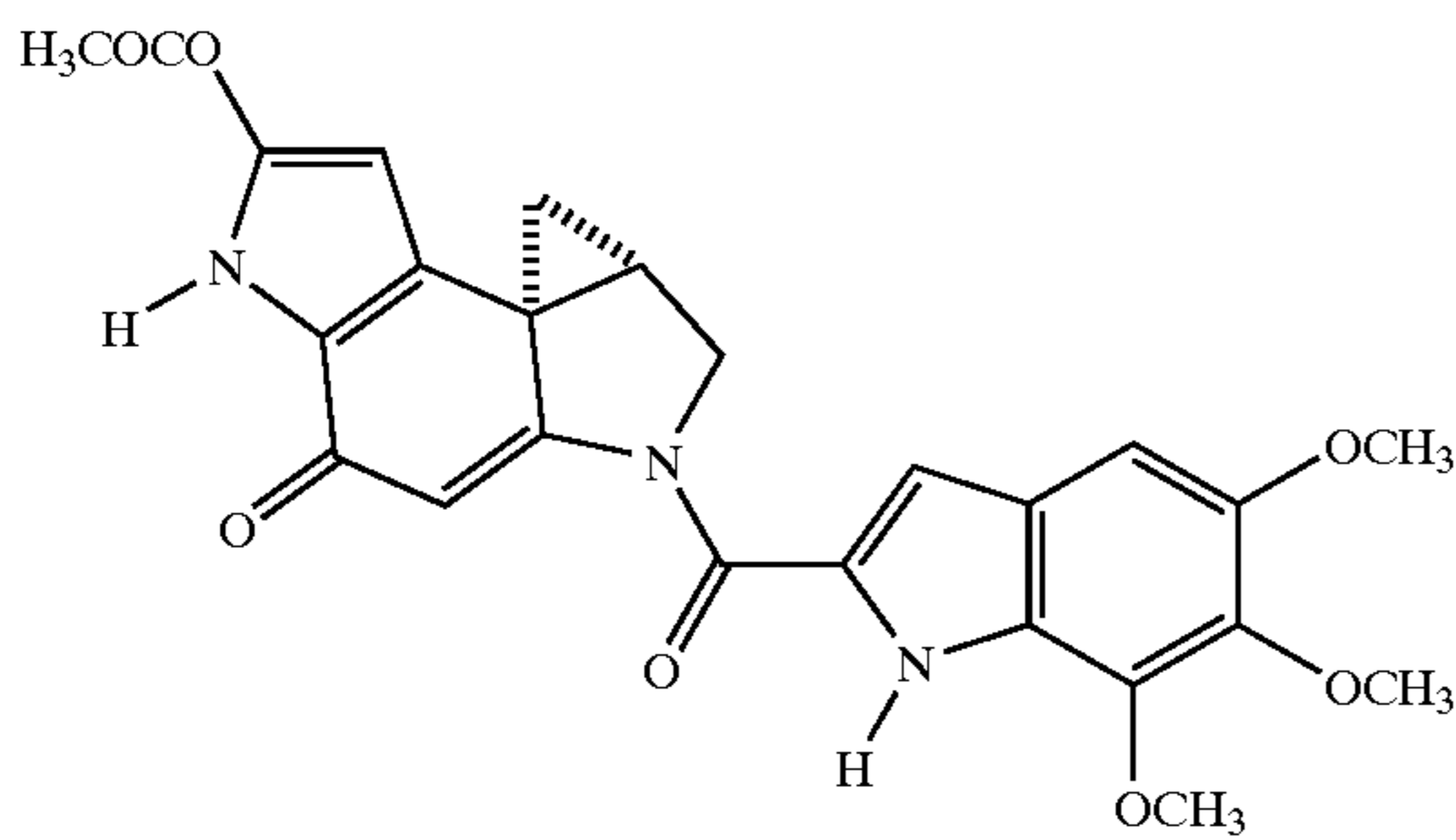
Duocarmycin SA
