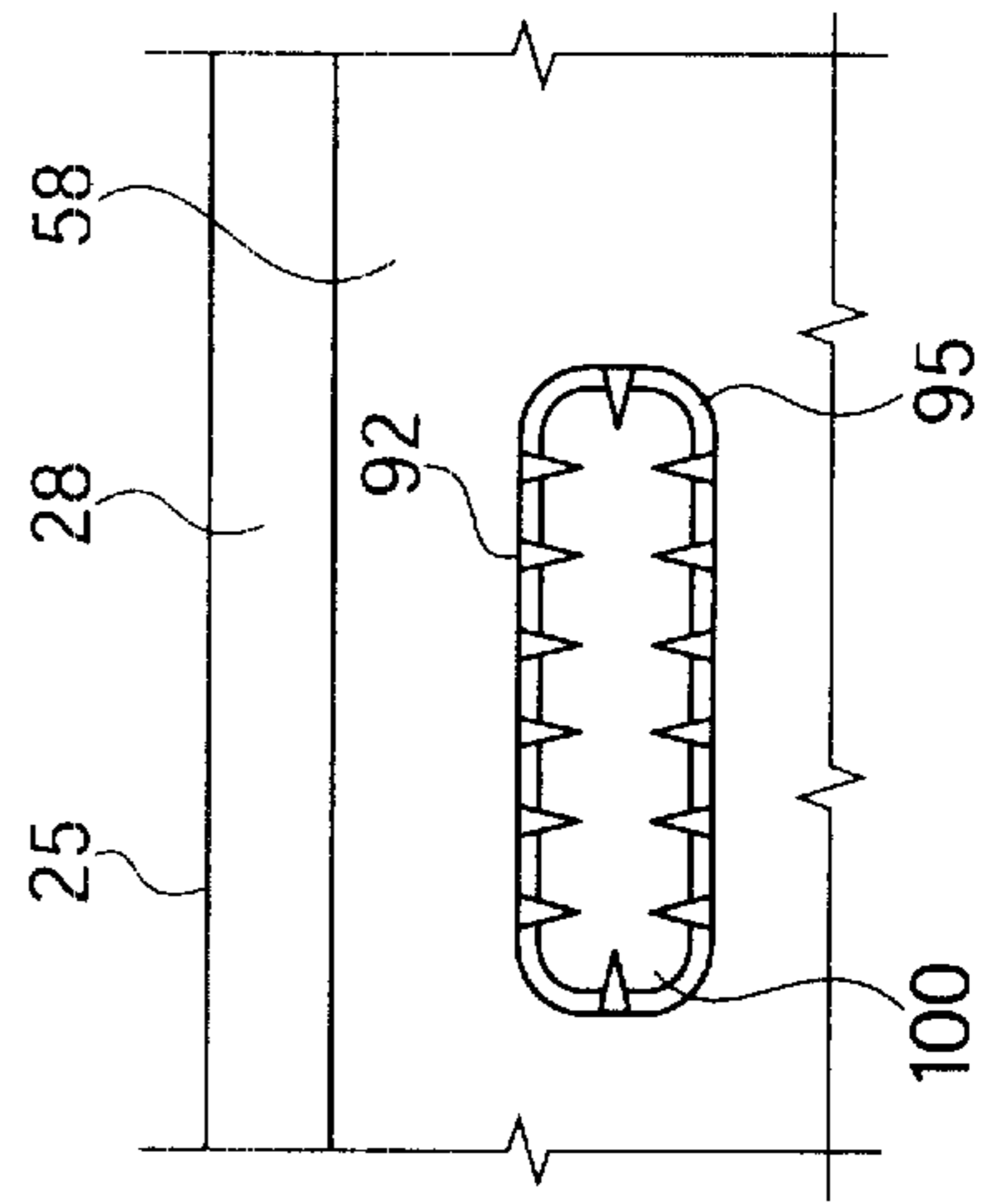
FIG. 7 A-A'
