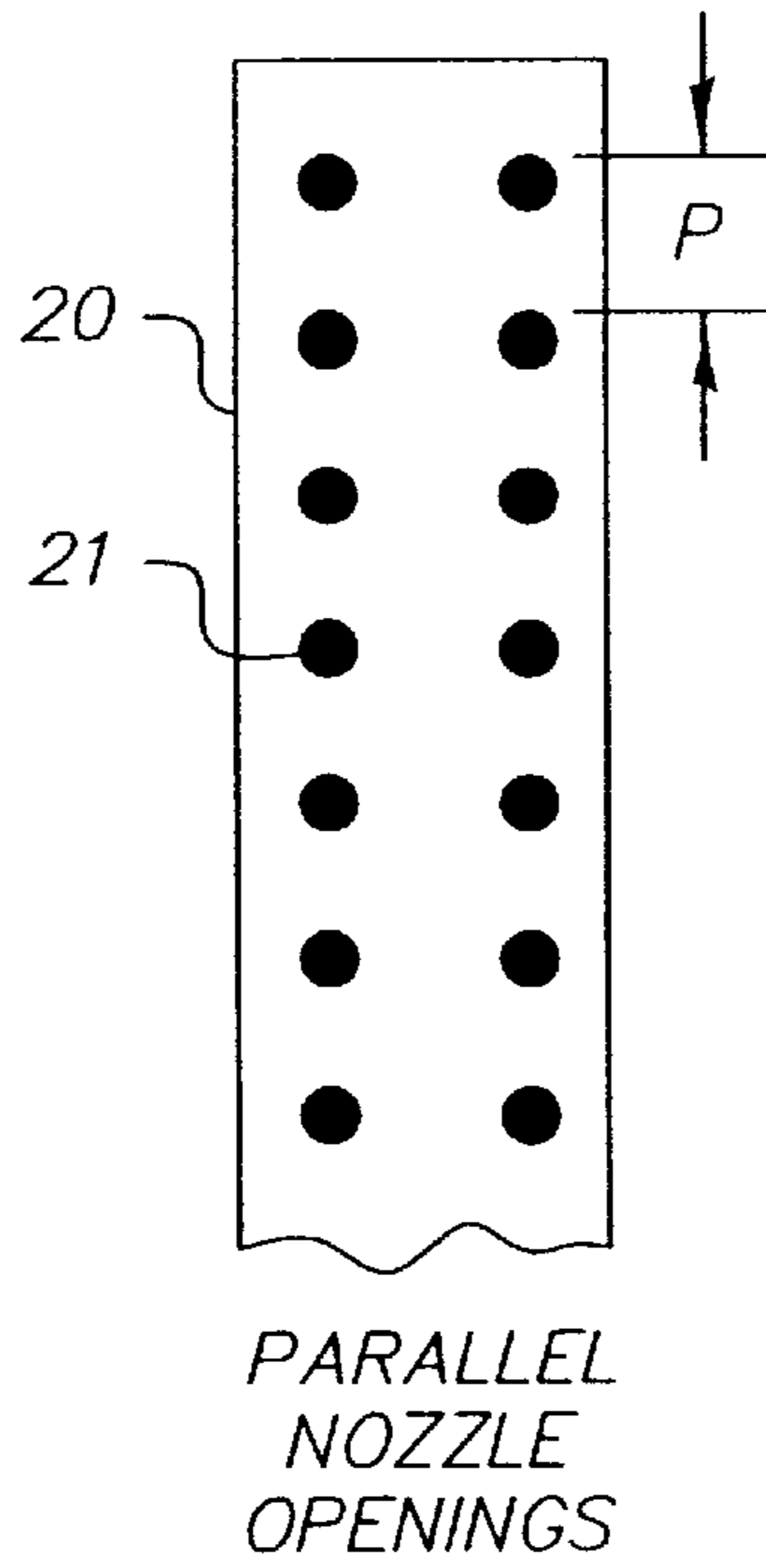
FIG. 5A
