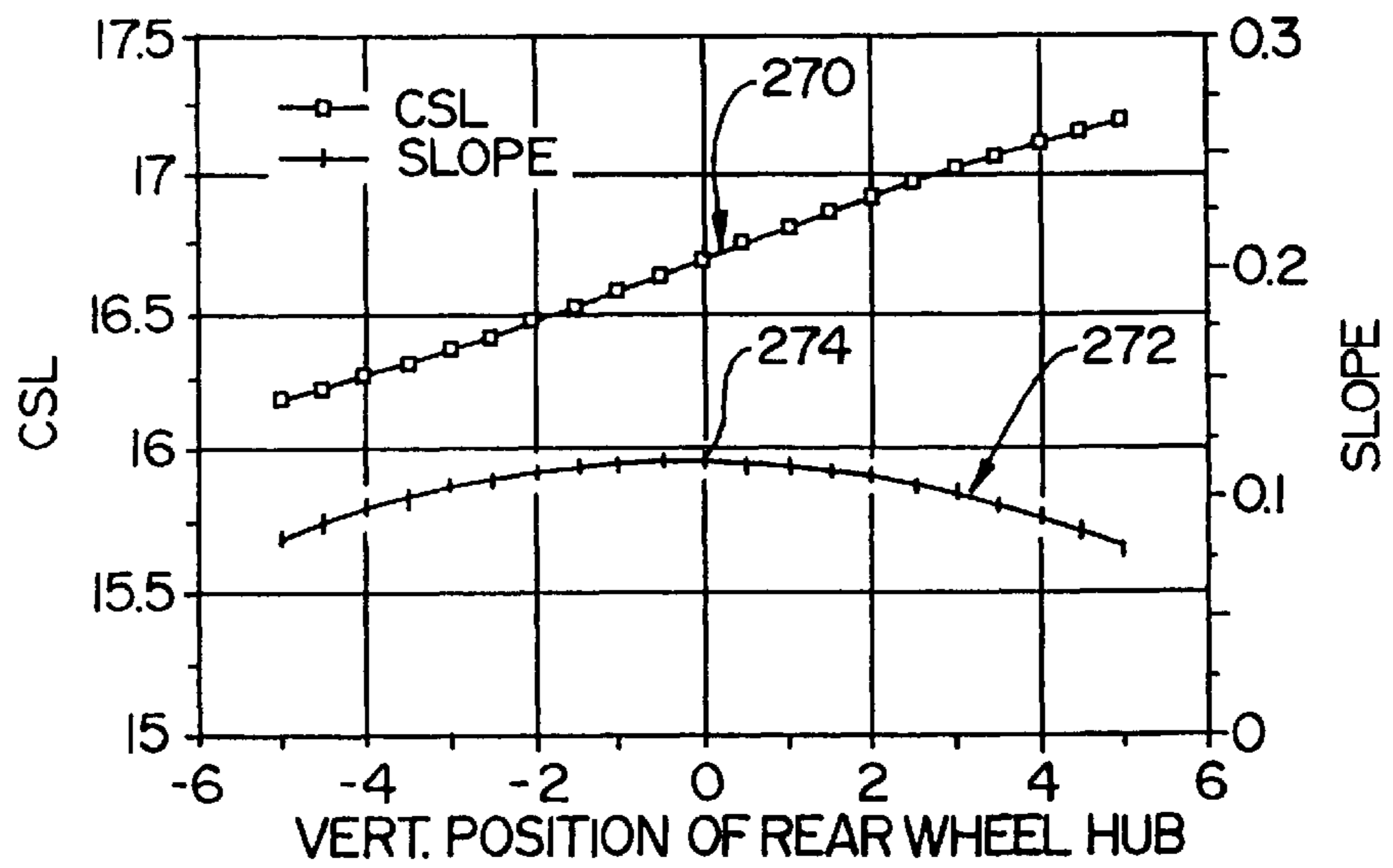
FIG. 16B
