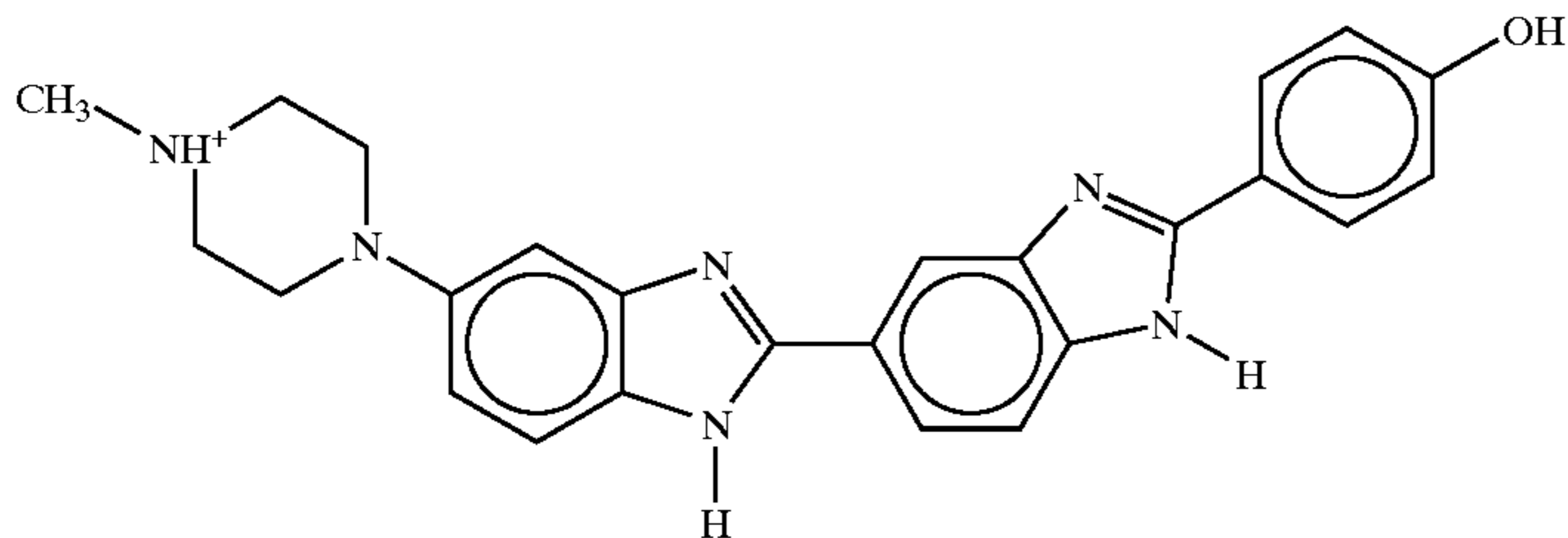
Hoechst 33258
