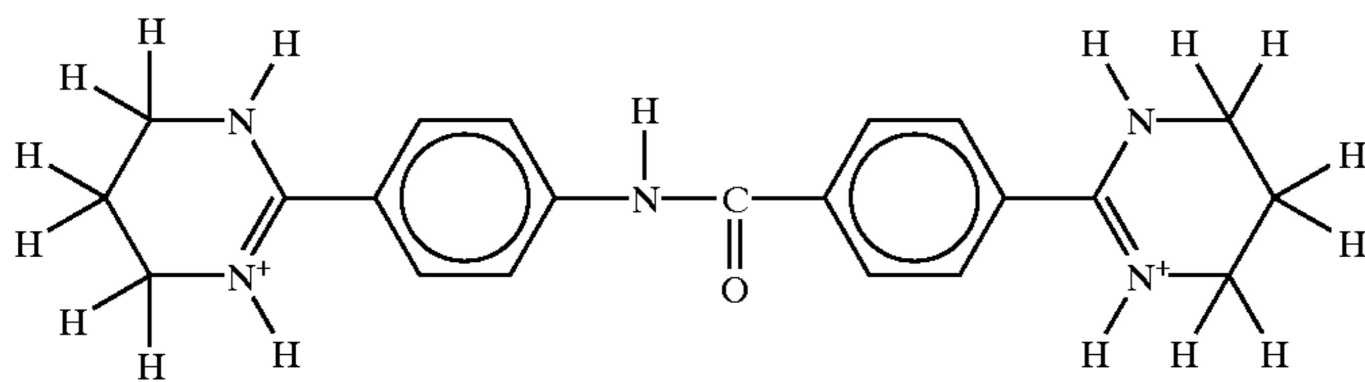
NSC 57153
