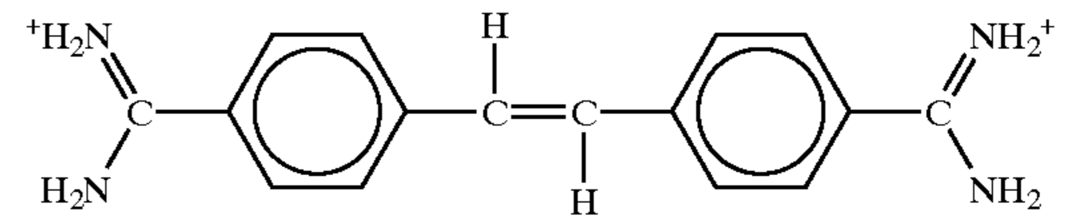
Stilbamidine
