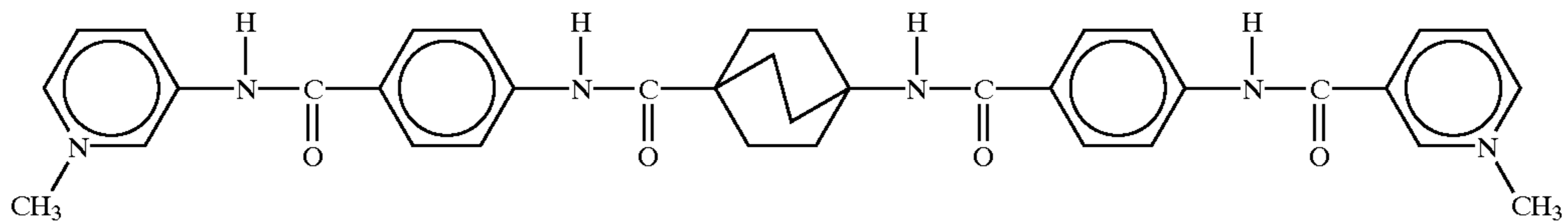
SN 16814
