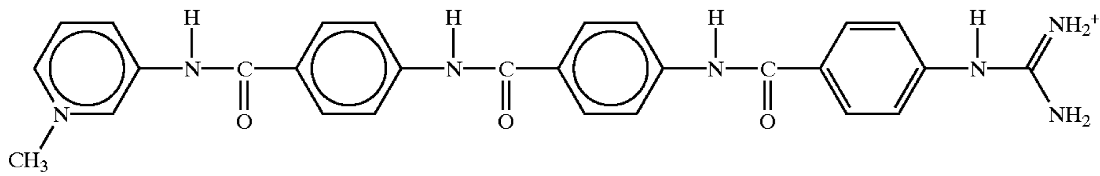
SN 6136
