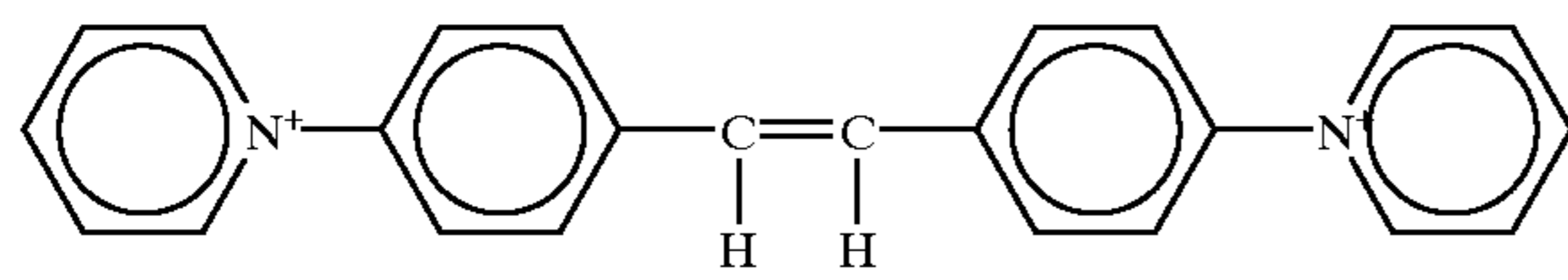
SN 18071
