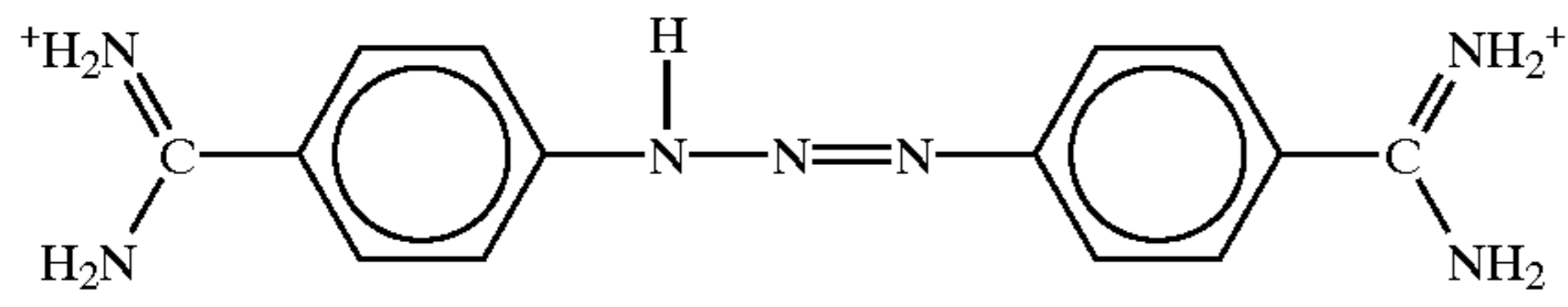
Berenil
