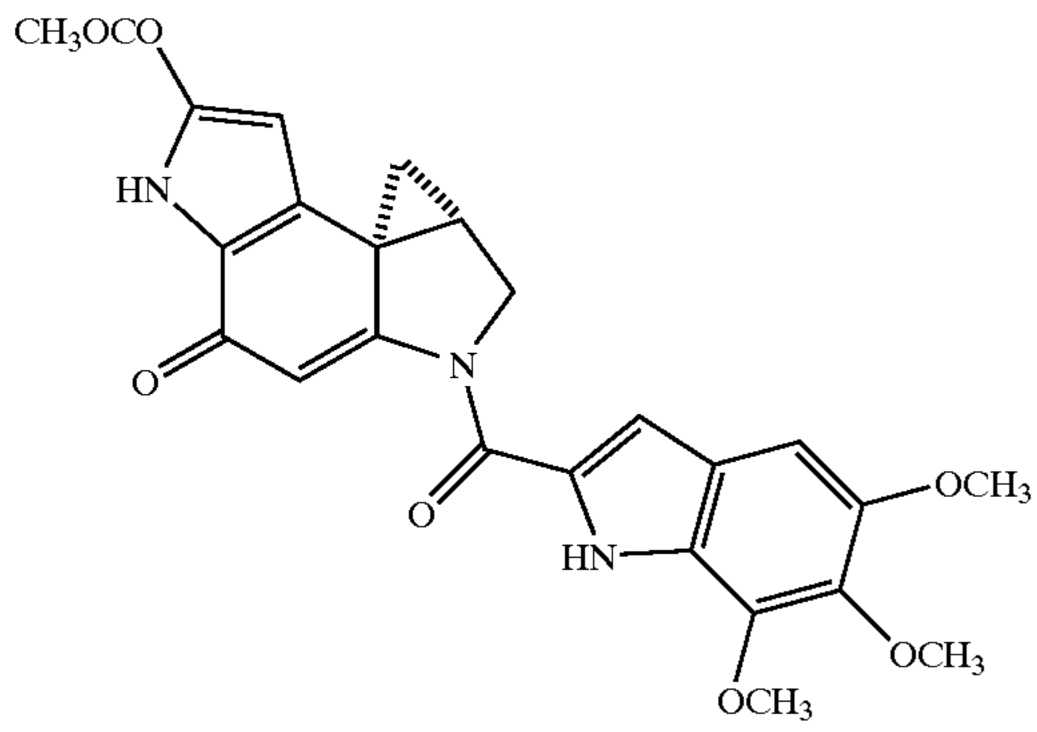
Duocarmycin SA
