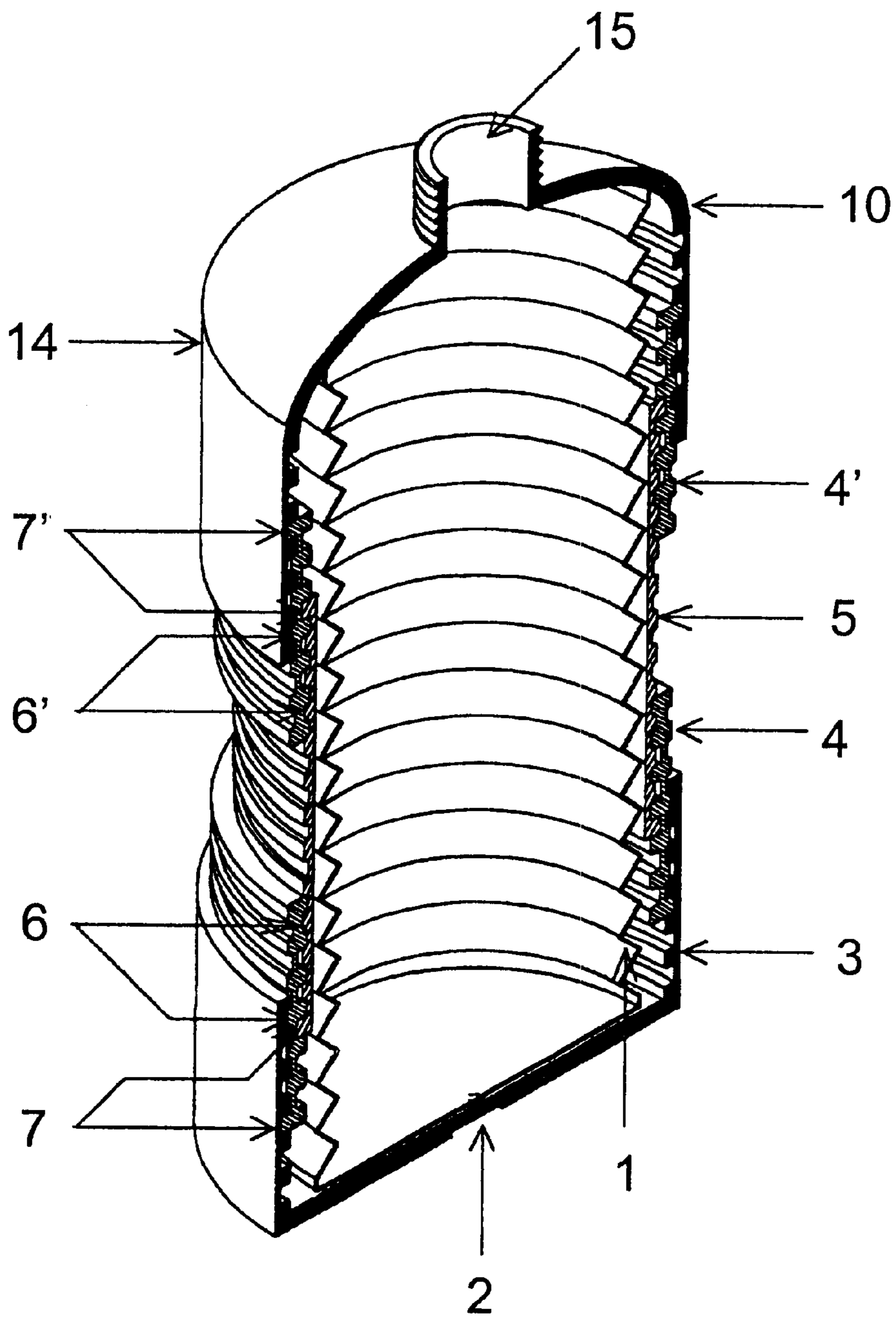
FIG. 1
