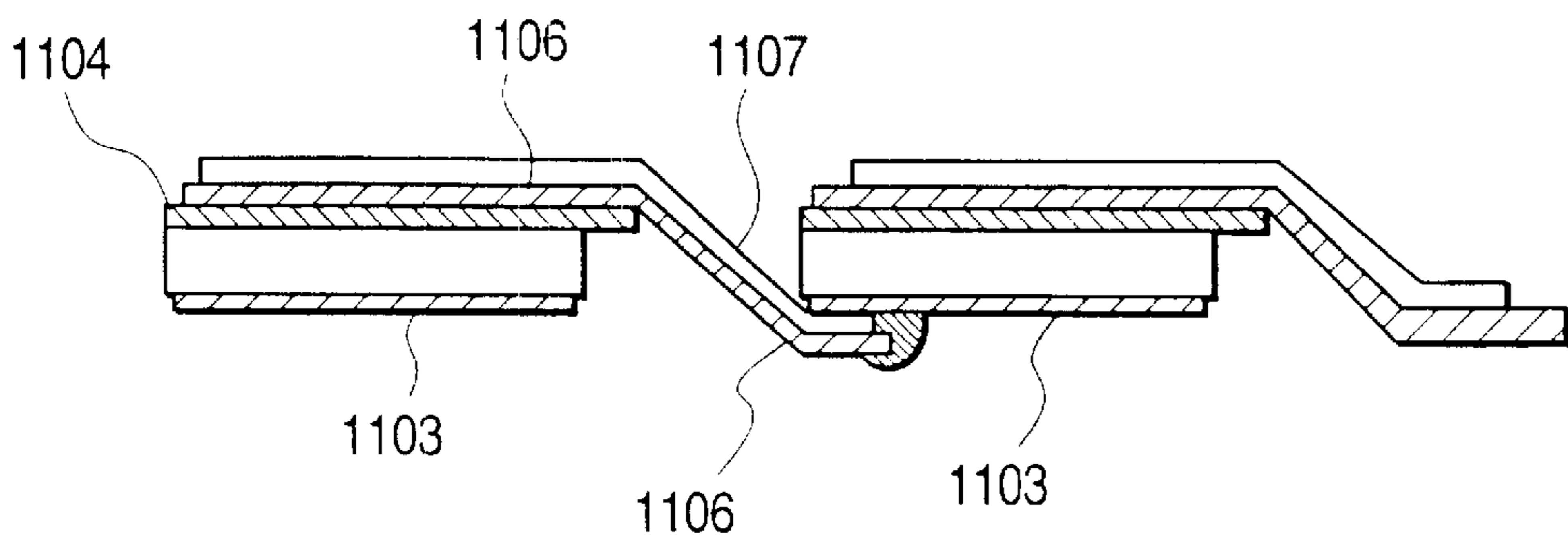
FIG. 11C
