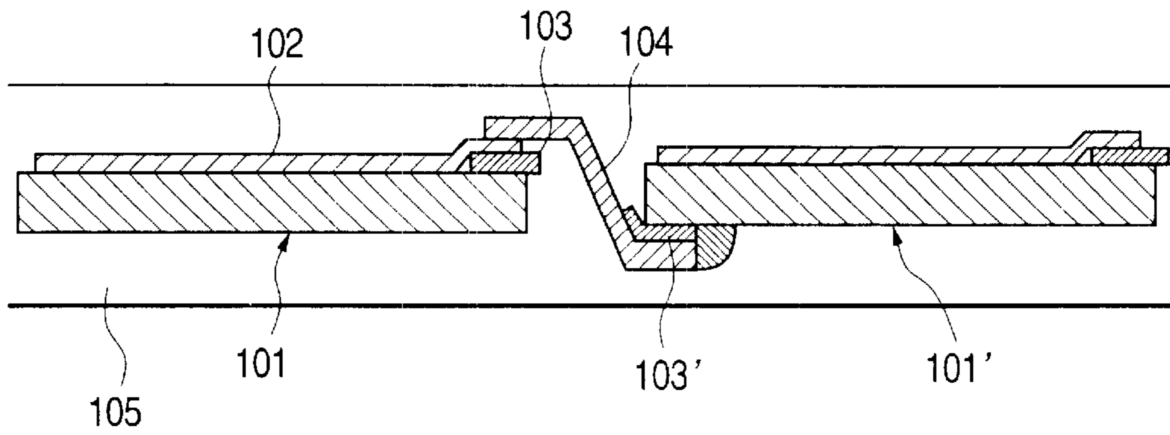
FIG. 5B
