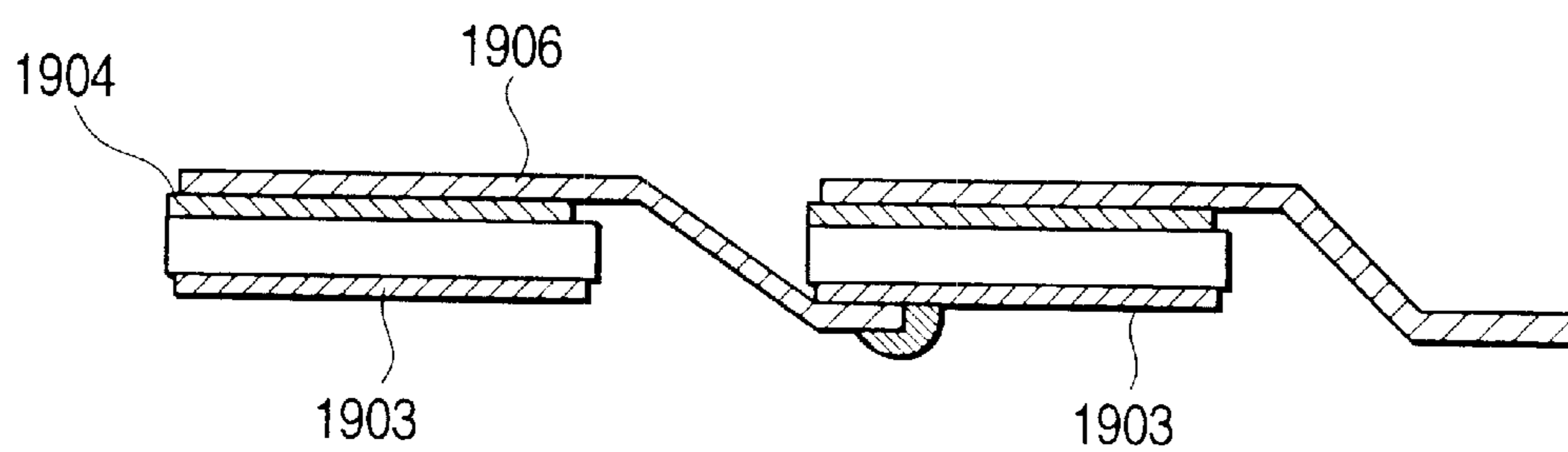
FIG. 19C
