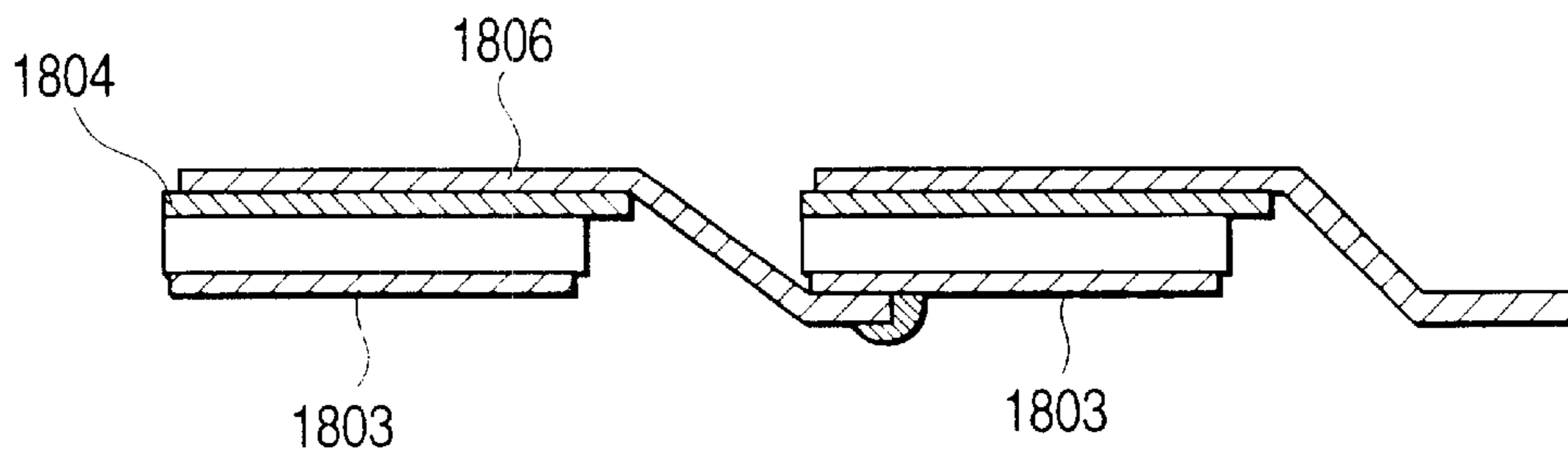
FIG. 18C
