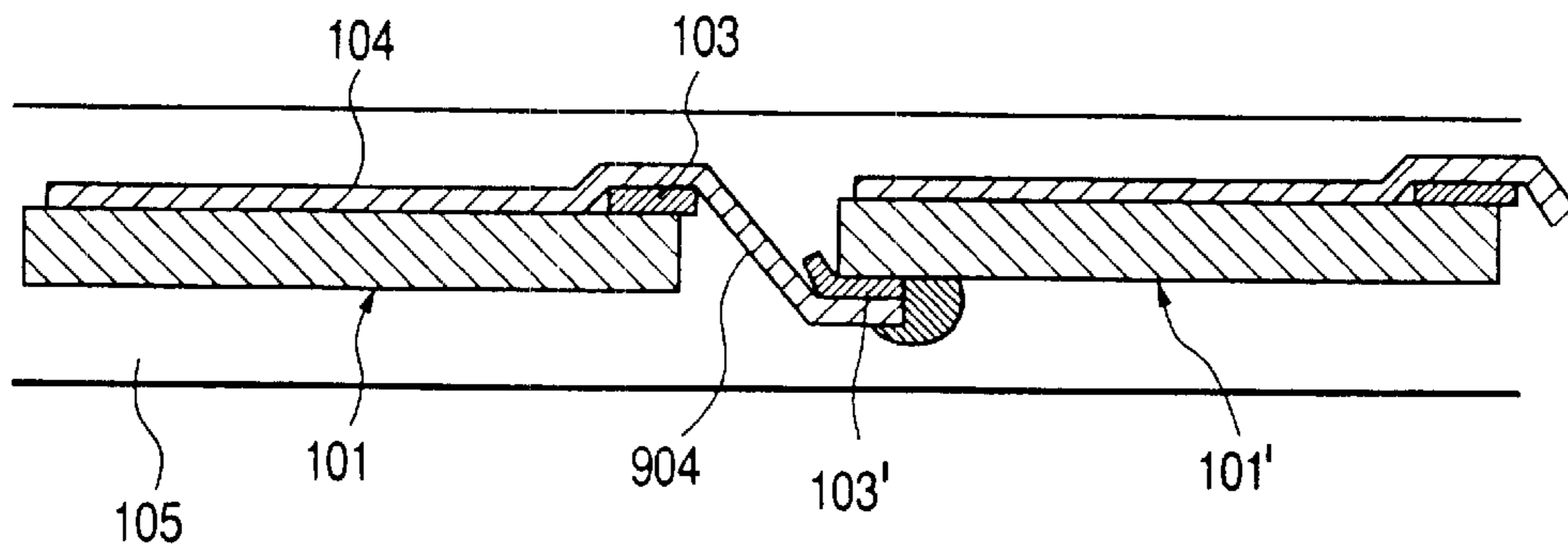
FIG. 7B
