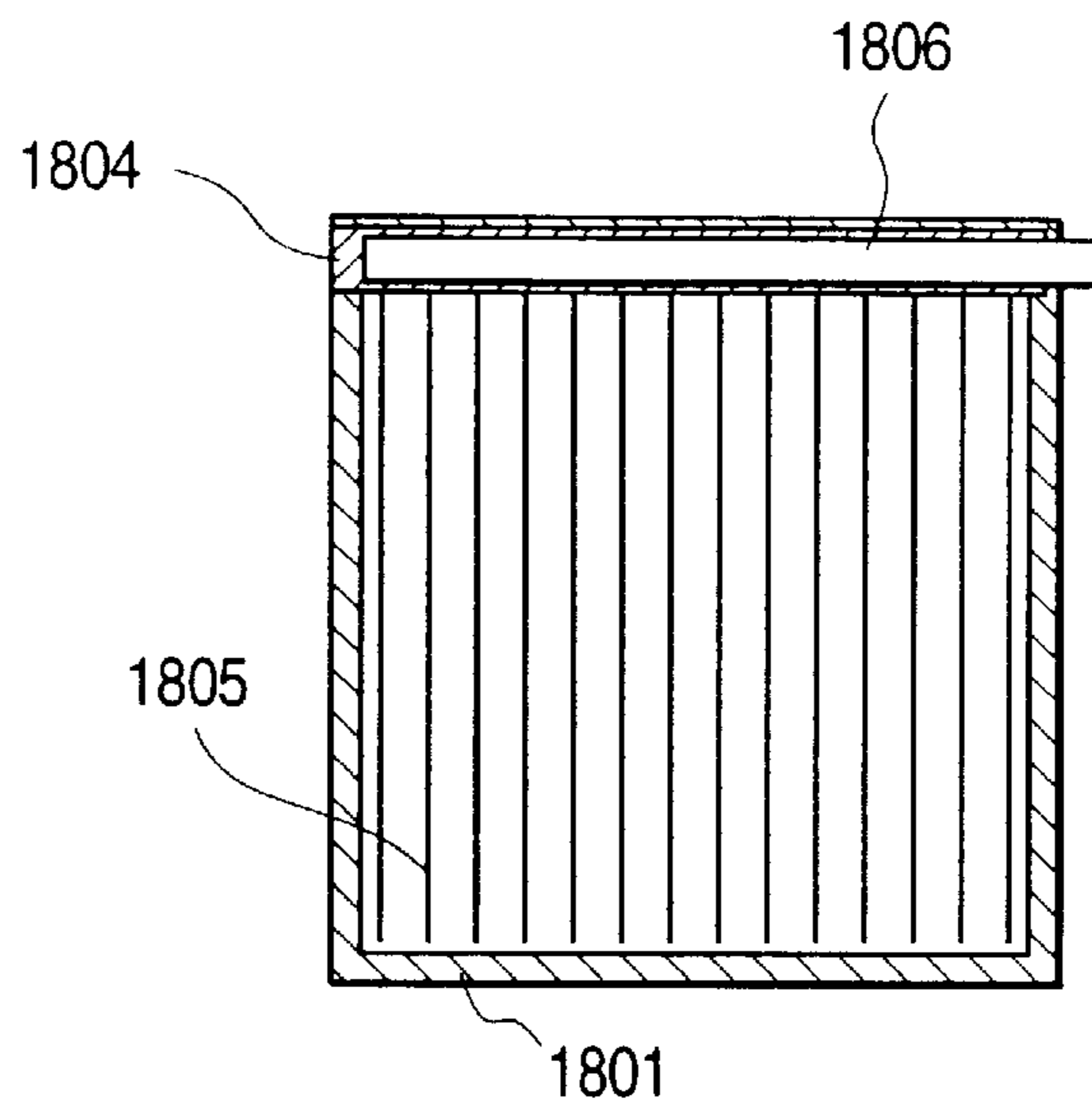
FIG. 18A
