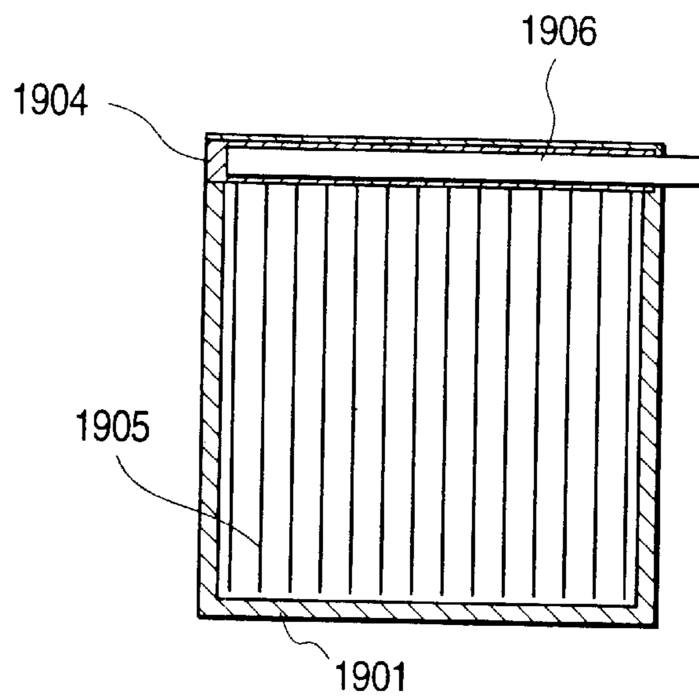
FIG. 19A
