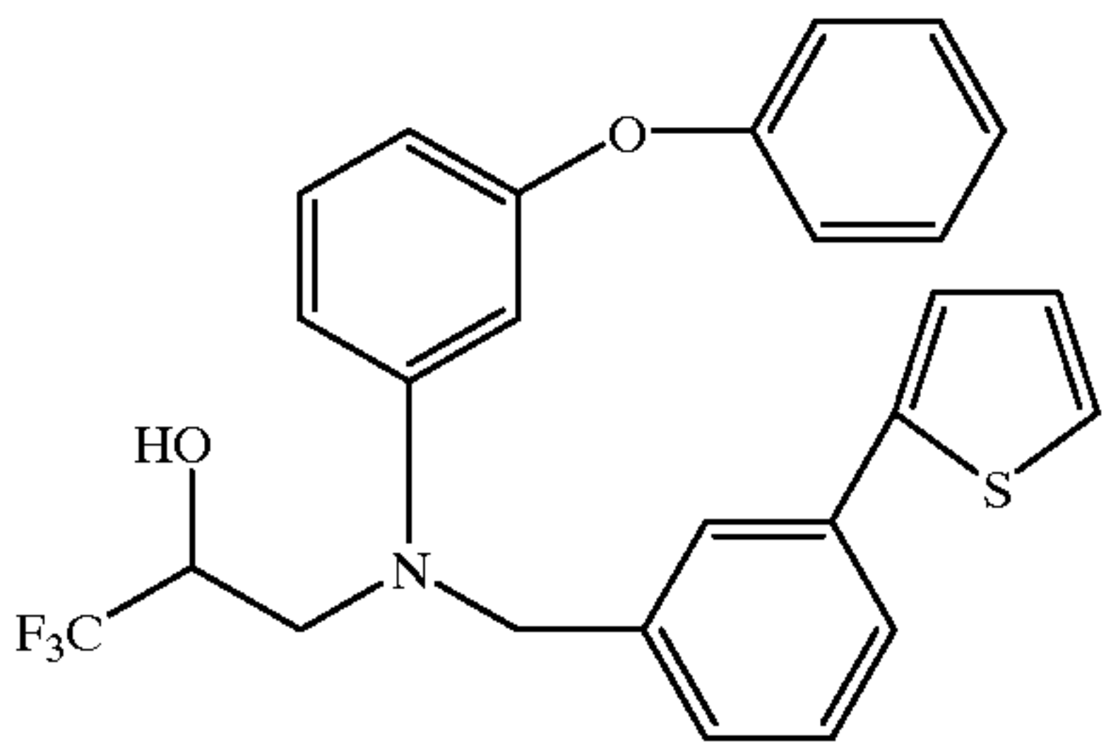
3-[(3-phenoxyphenyl) [[3-(2-thienyl)phenyl]methyl]amino]-1,1,1-trifluoro-2-propanol
