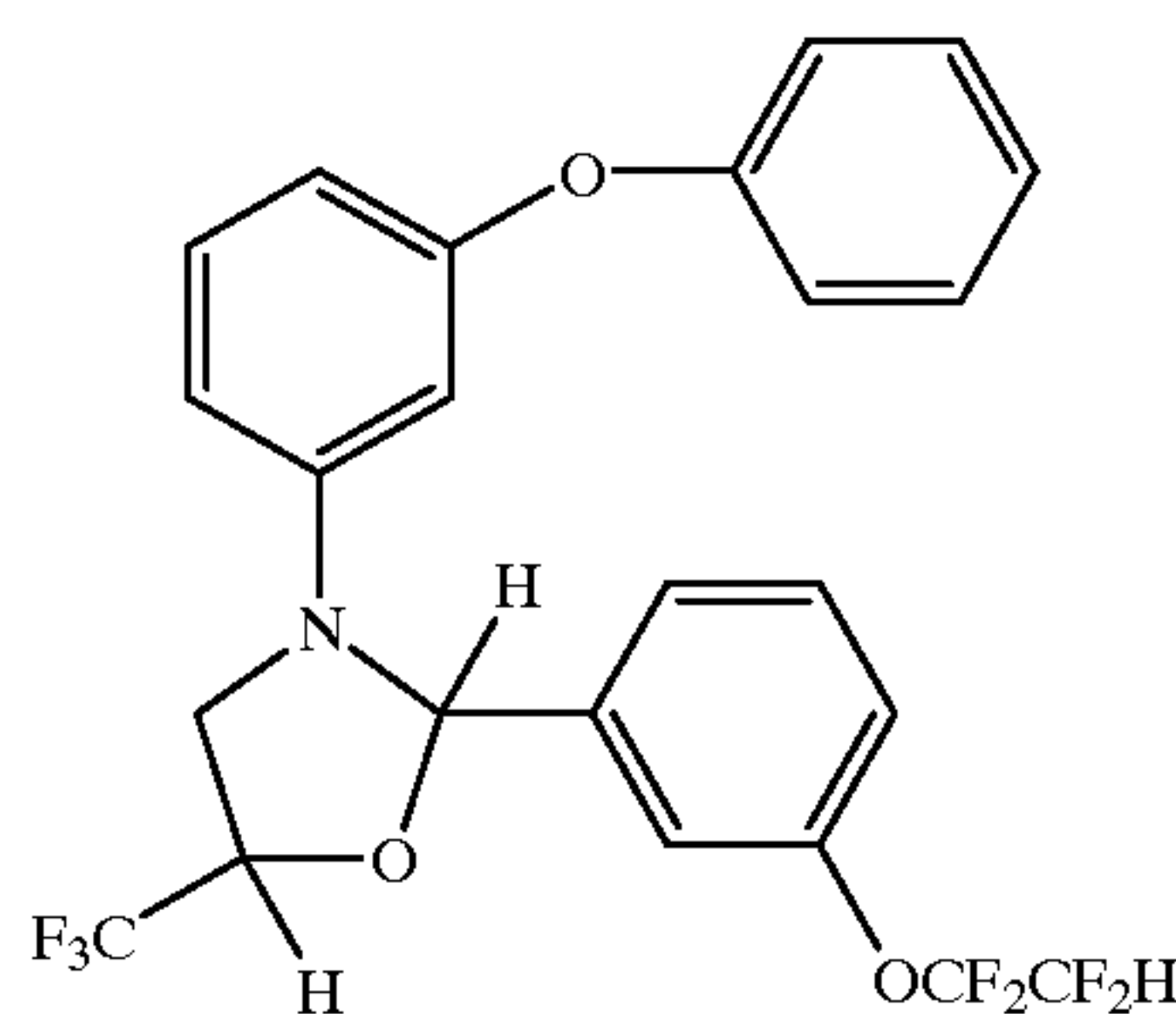
3-(3-phenoxyphenyl)-2-[3-(1,1,2,2-tetrafluoroethoxy)phenyl]-5-(trifluoromethyl)oxazolidine
