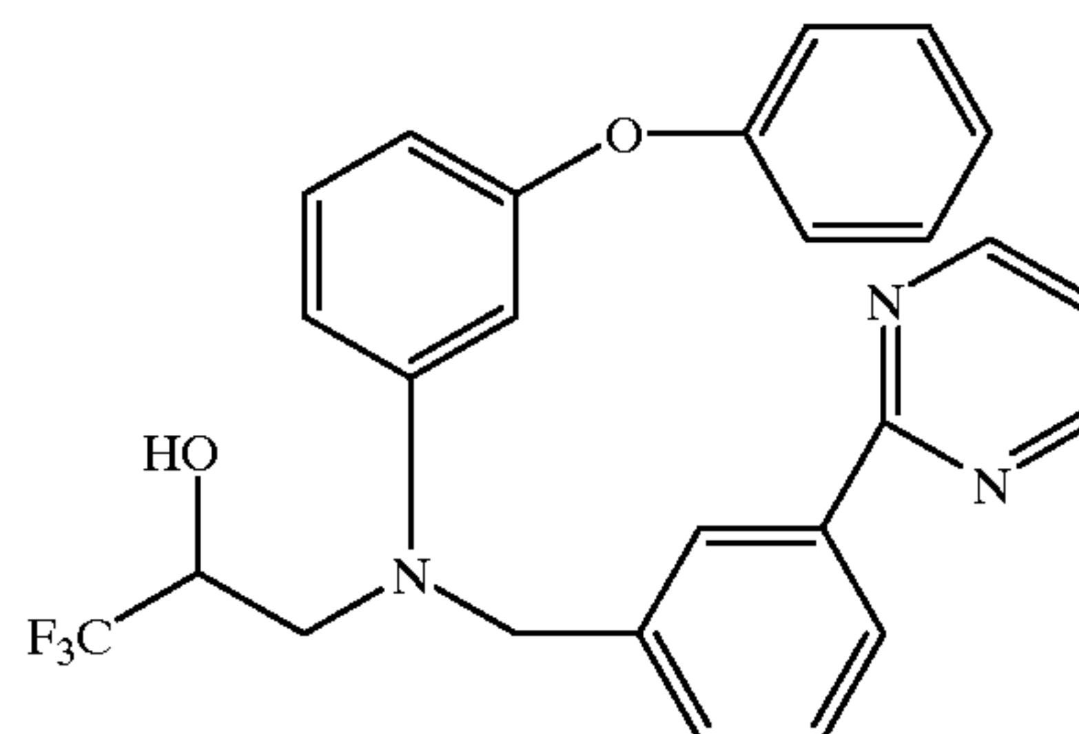
3-[(3-phenoxyphenyl)[[3-(2-pyrimidinyl)phenyl]methyl]amino]-1,1,1-trifluoro-2-propanol
