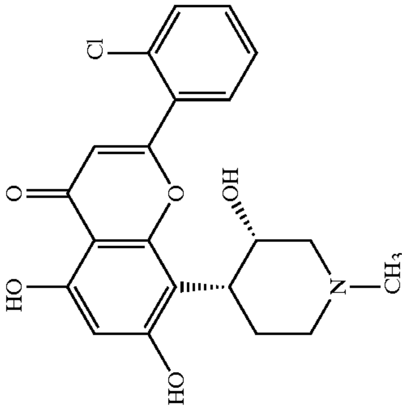
Flavopiridol
