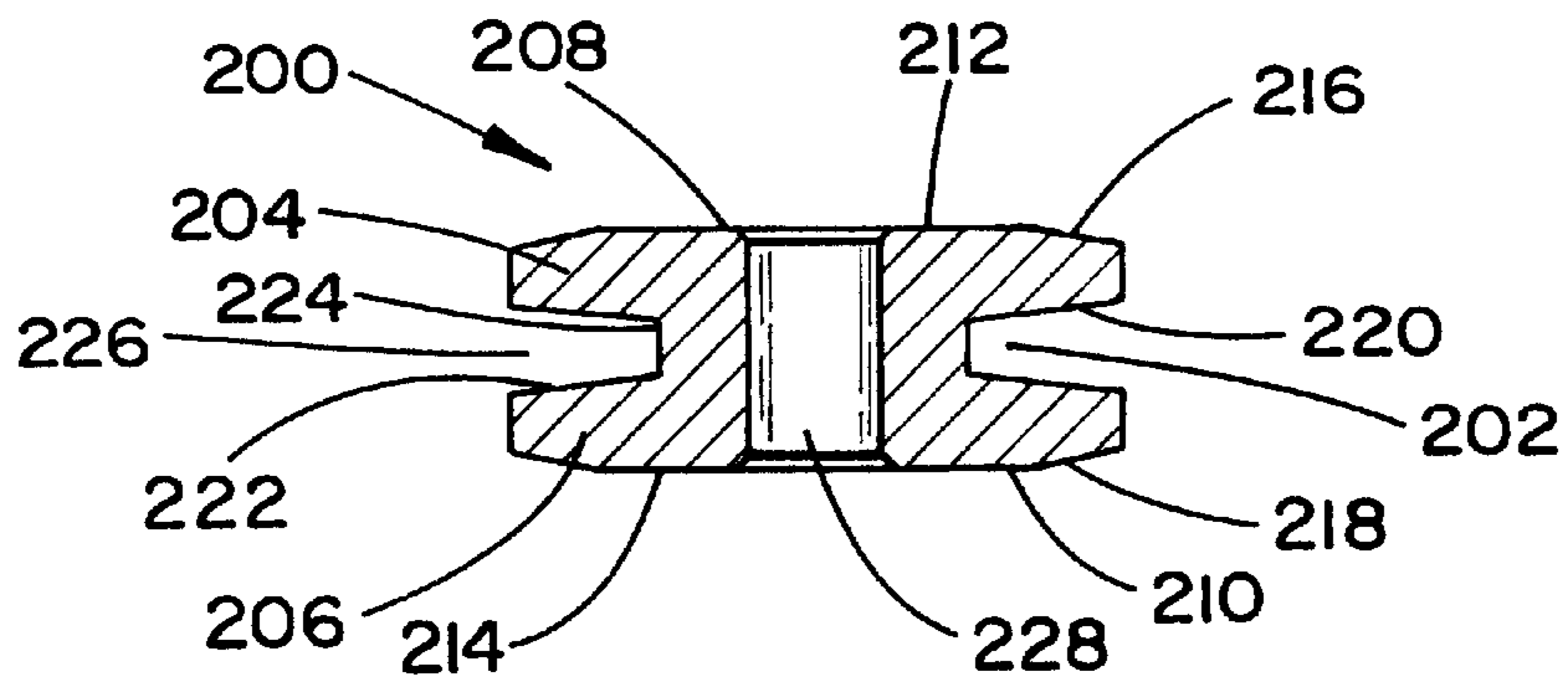
Section A-A
