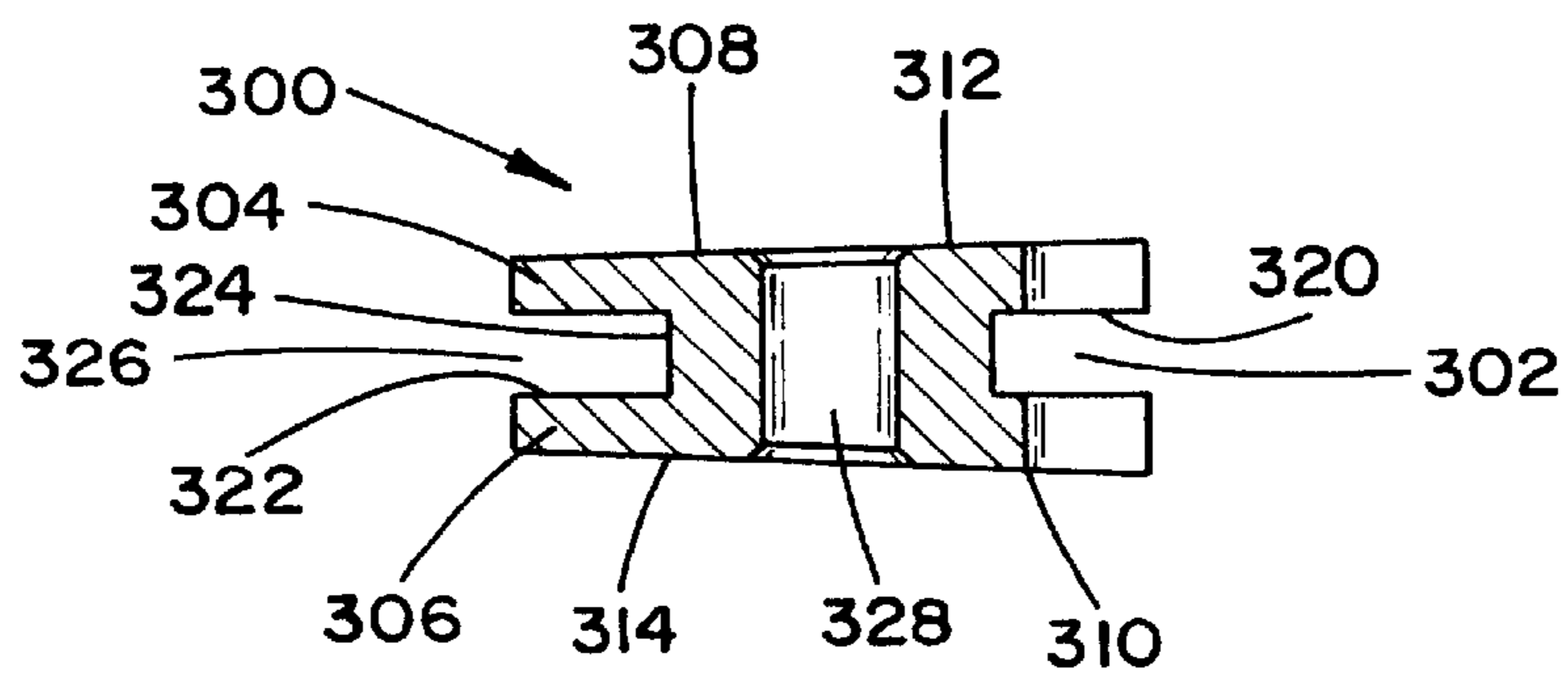
Section A-A
