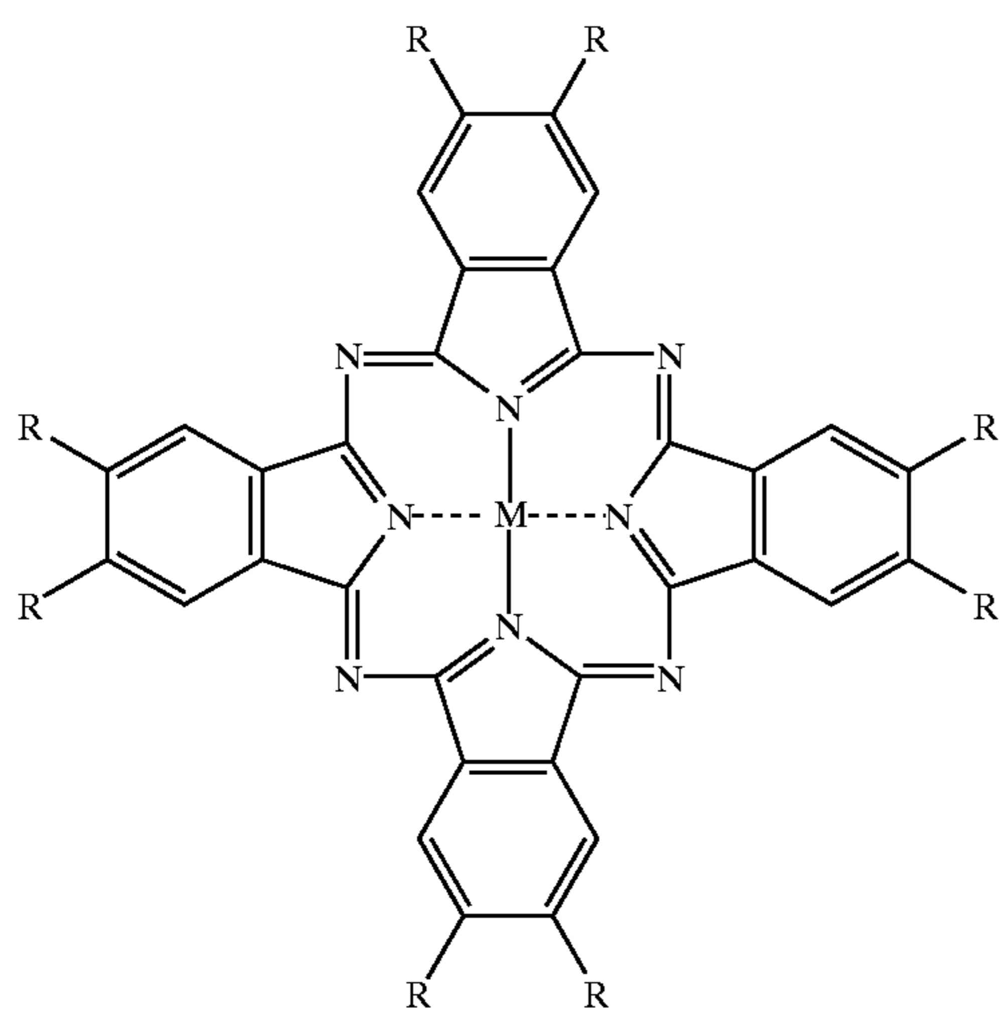
2,3-octasubstituted
