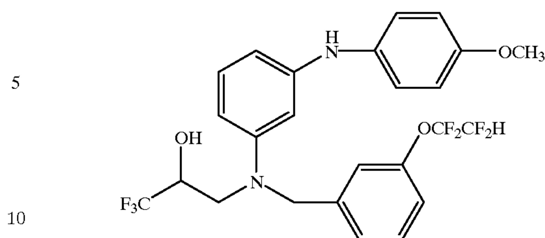
3-[[3-[(4-methoxyphenyl)amino]phenyl]-[3-(1,1,2,2-tetrafluoroethoxy)phenyl]methyl]amino]-1,1,1-trifluoro-2-propanol
