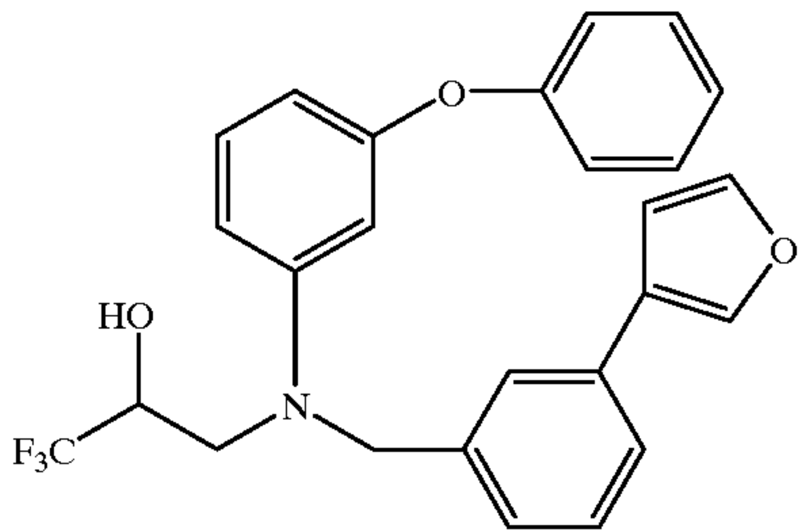
3-[(3-phenoxyphenyl)[[3-(3-furanyl)phenyl]methyl]amino]-1,1,1-trifluoro-2-propanol
