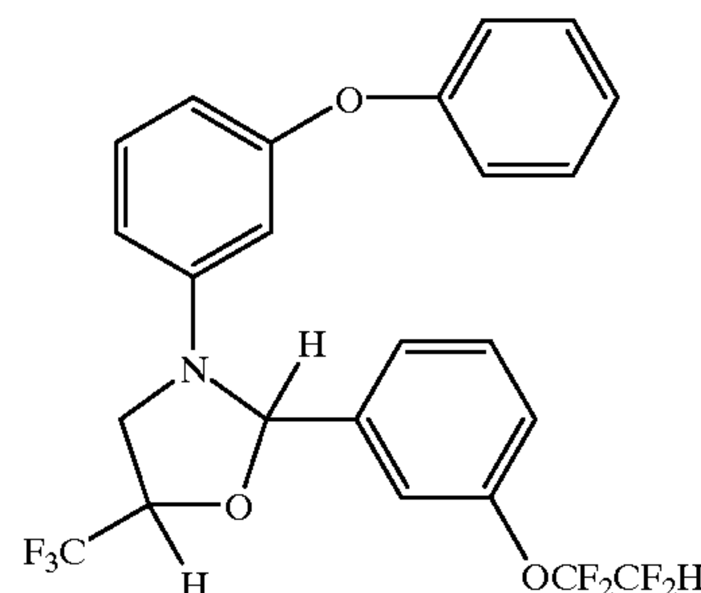
3-(3-phenoxyphenyl)-2-[3-(1,1,2,2-tetrafluoroethoxy)phenyl]-5-(trifluoromethyl)oxazolidine
