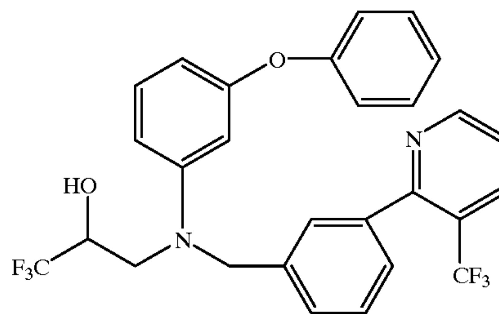
3-[(3-phenoxyphenyl)[[3-(2-pyridinyl)phenyl]methyl]amino]-1,1,1-trifluoro-2-propanol
