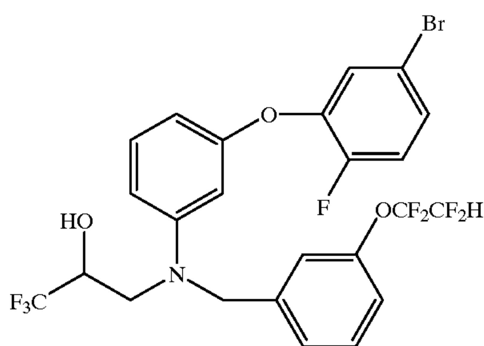
3-[3-(5-bromo-2-fluorophenoxy)phenyl][3-(1,1,2,2-tetrafluoroethoxy)phenyl]methyl]amino]-1,1,1-trifluoro-2-propanol
