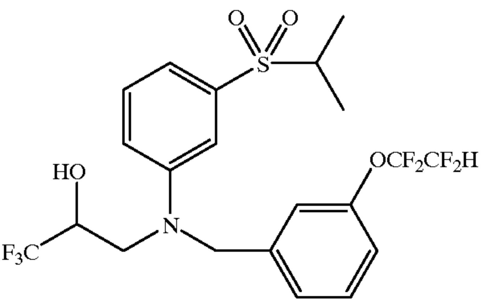
3-[[[3-[(1-methylethyl)sulfonyl]phenyl][[3-(1,1,2,2-tetrafluoroethoxy)-phenyl]methyl]amino]-1,1,1-trifluoro-2-propanol
