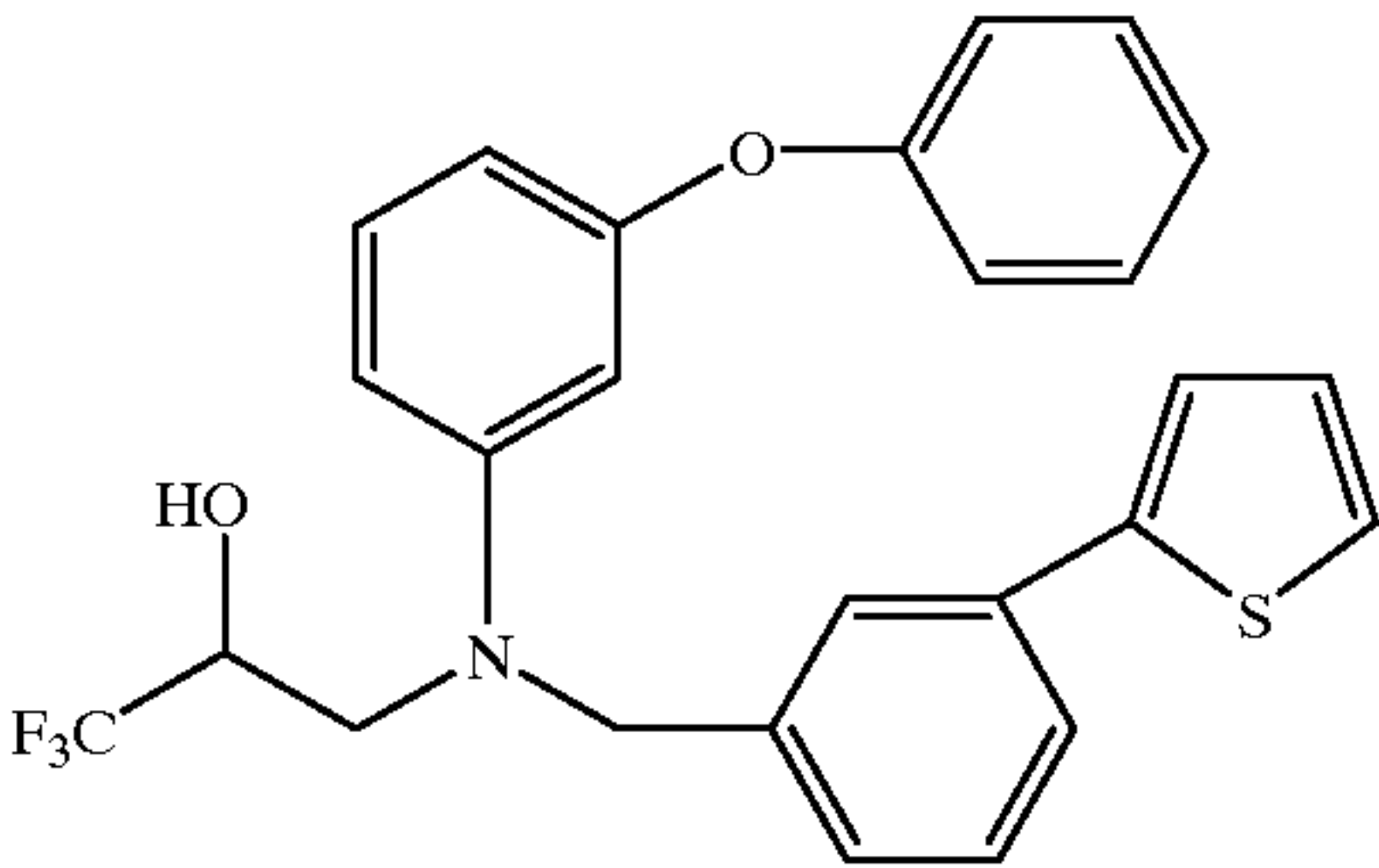
3-[(3-phenoxyphenyl) [[3-(2-thienyl)phenyl]methyl]amino]-1,1,1-trifluoro-2-propanol
