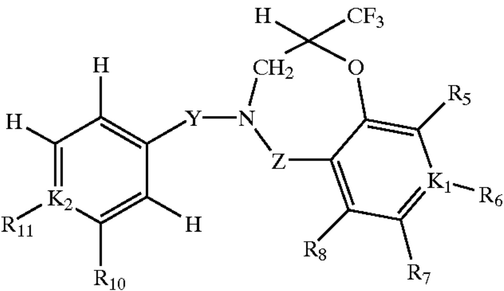
Cyclo-VII
