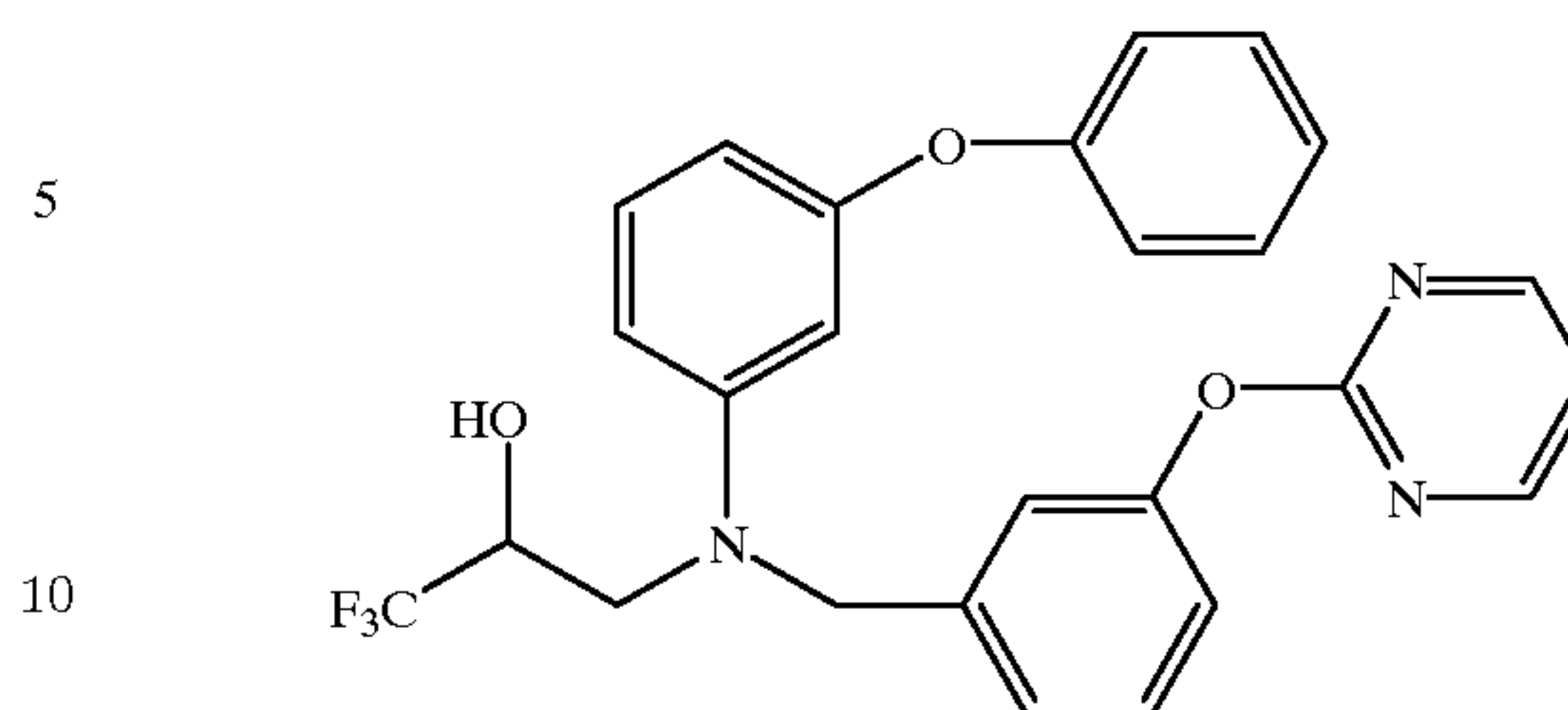
3-[(3-phenoxyphenyl)[[3-(2-pyrimidinyl)oxy]phenyl]methyl]amino]-1,1,1-trifluoro-2-propanol
