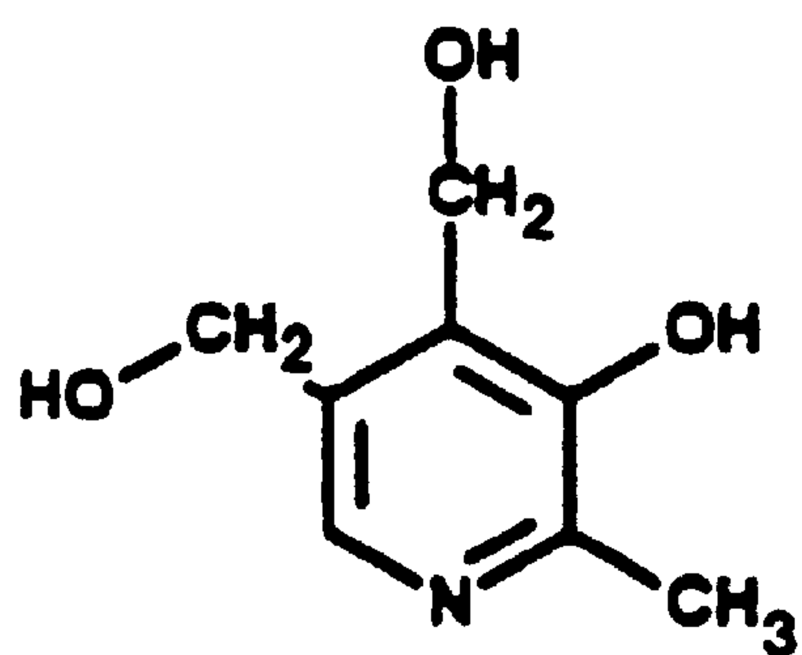
Pyridoxine
