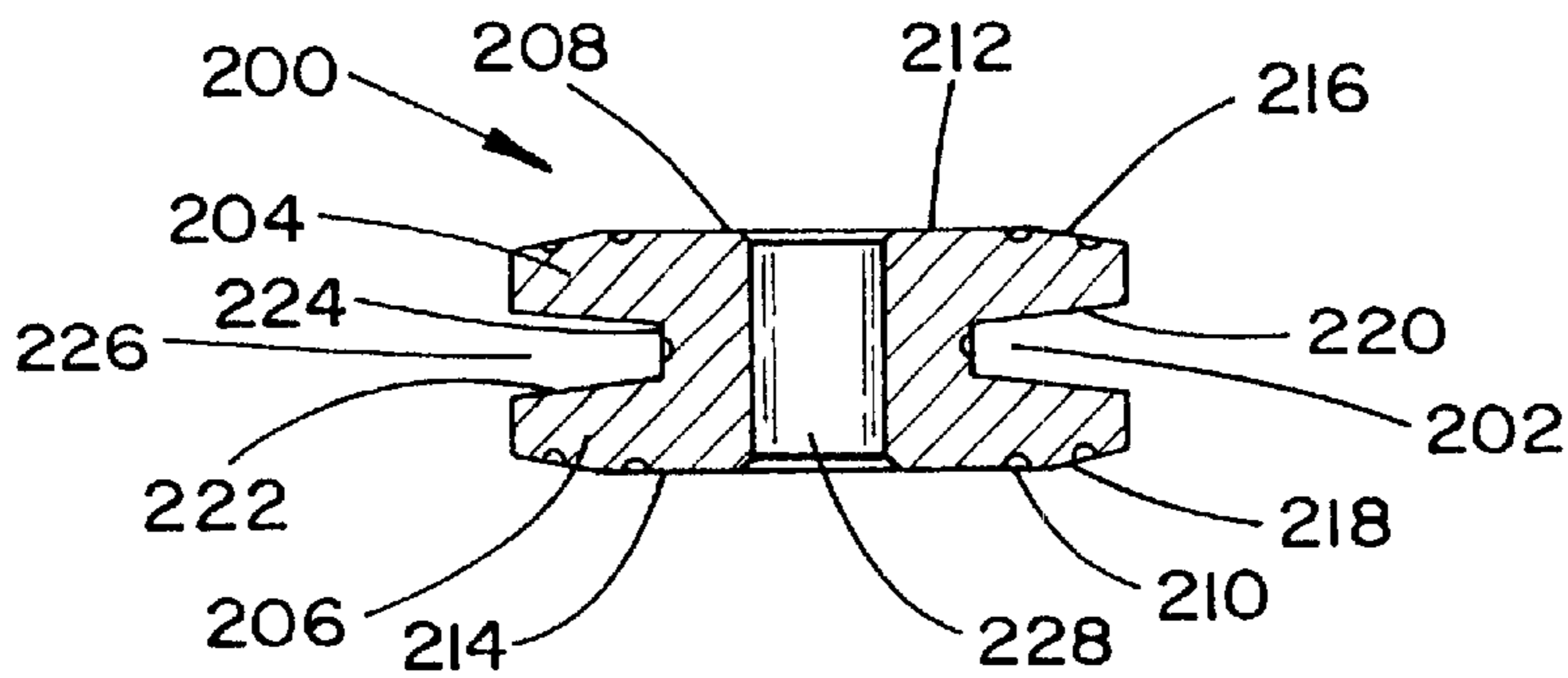
Section A-A
