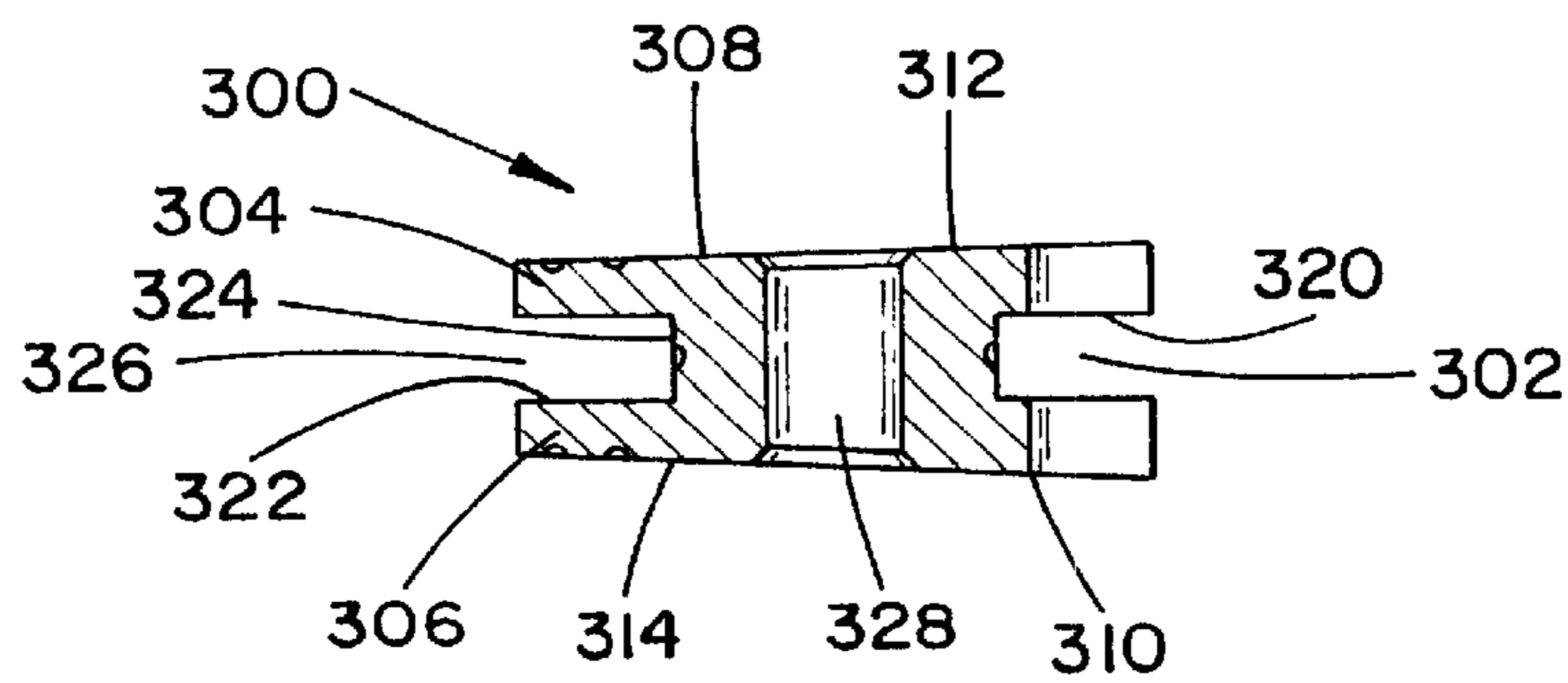
Section A-A
