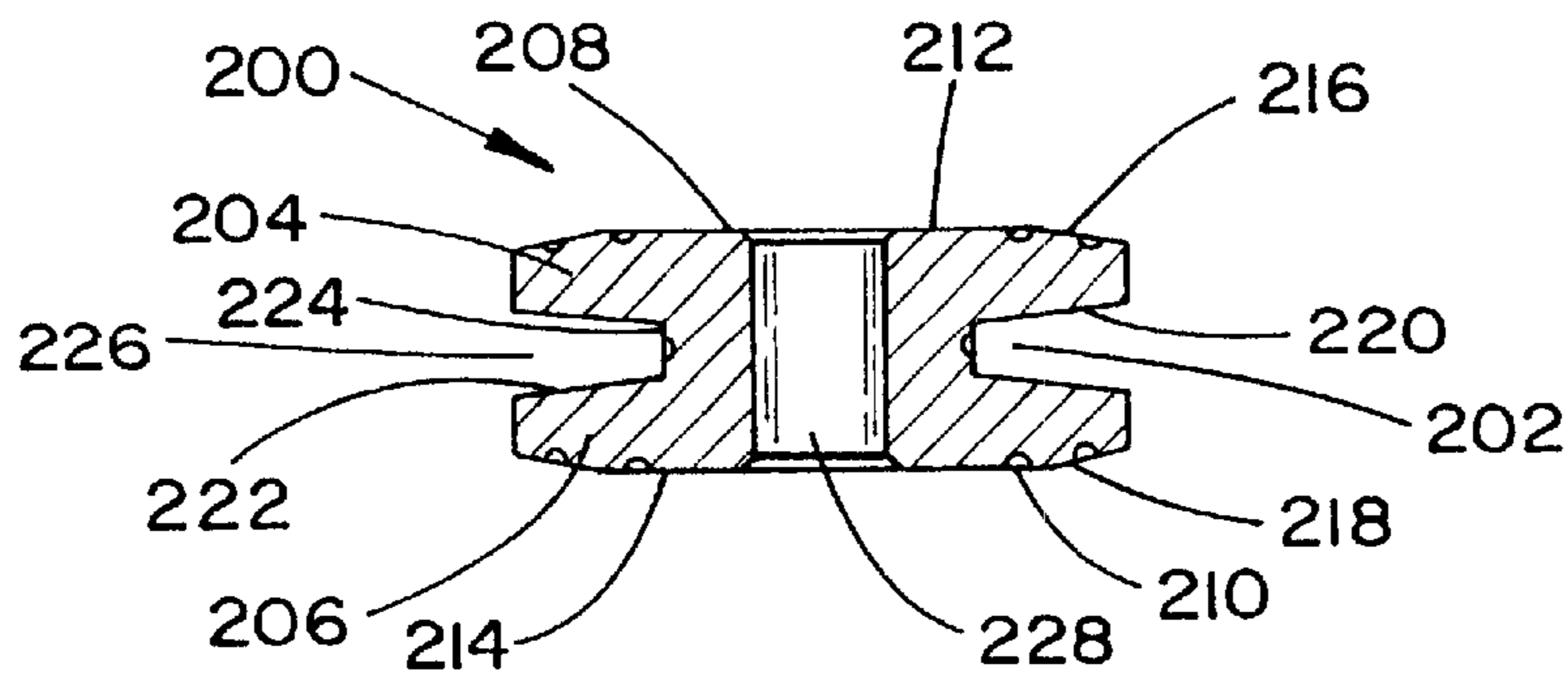
Section A-A
