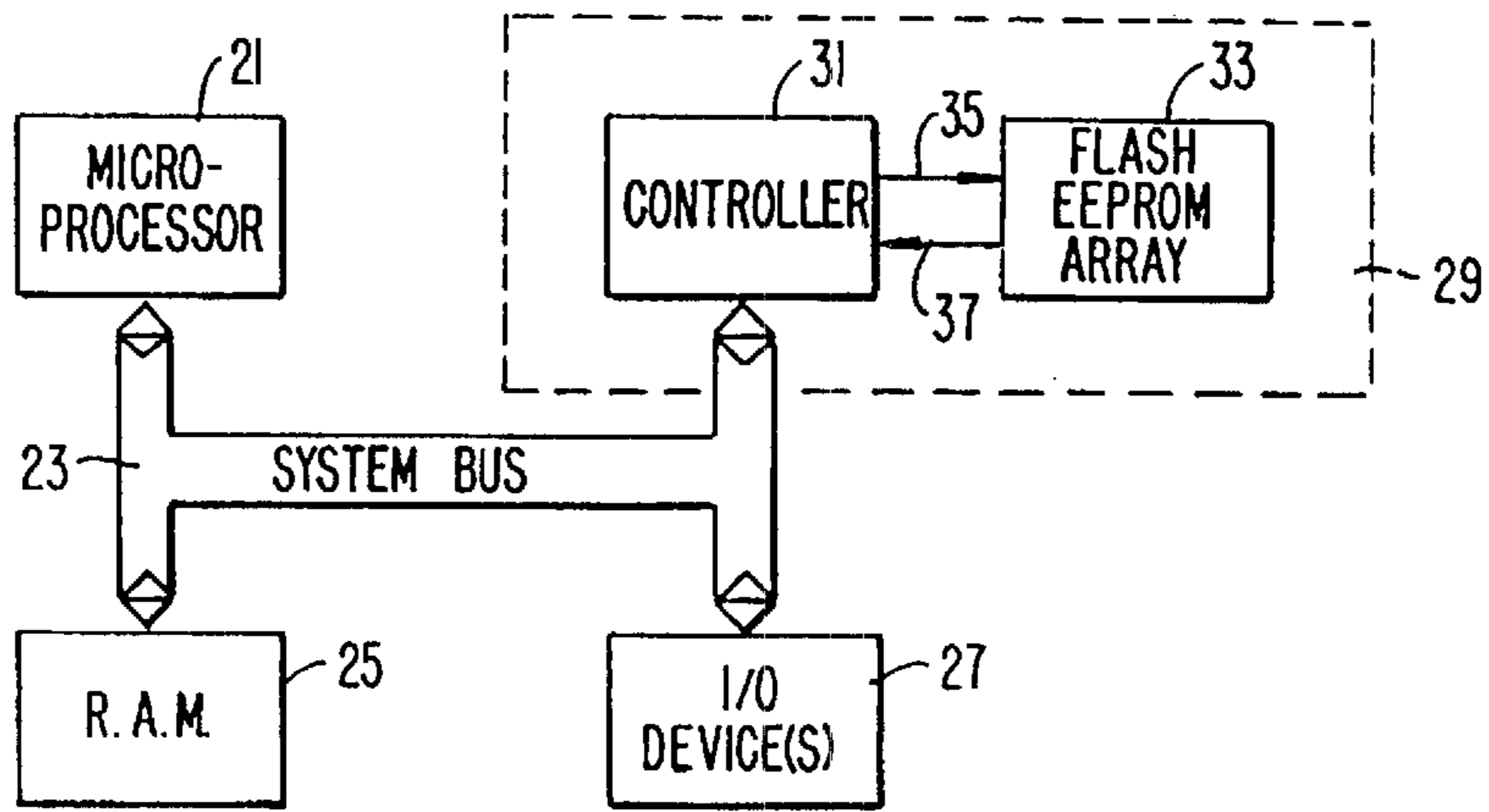
FIG. 1A
