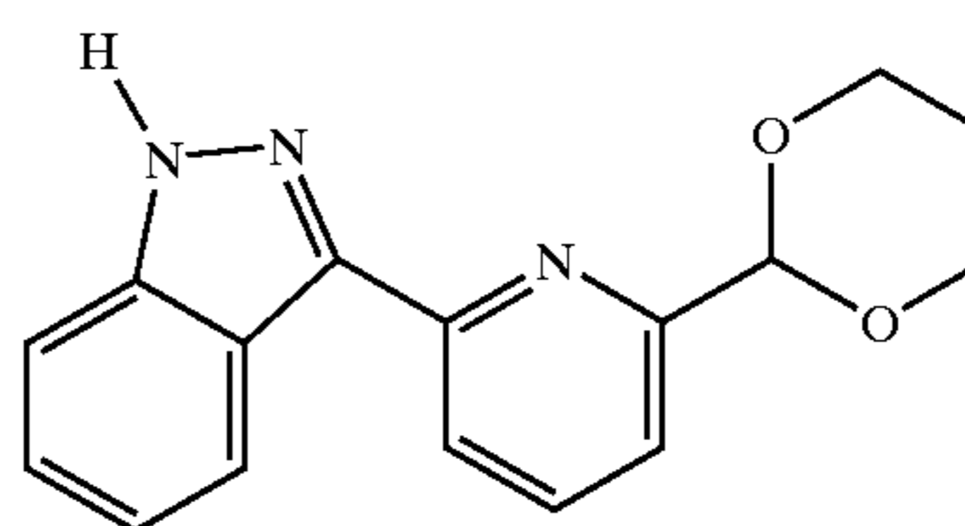
3-(6-(1,3-Dioxan-2-yl)-2-pyridyl)indazole
