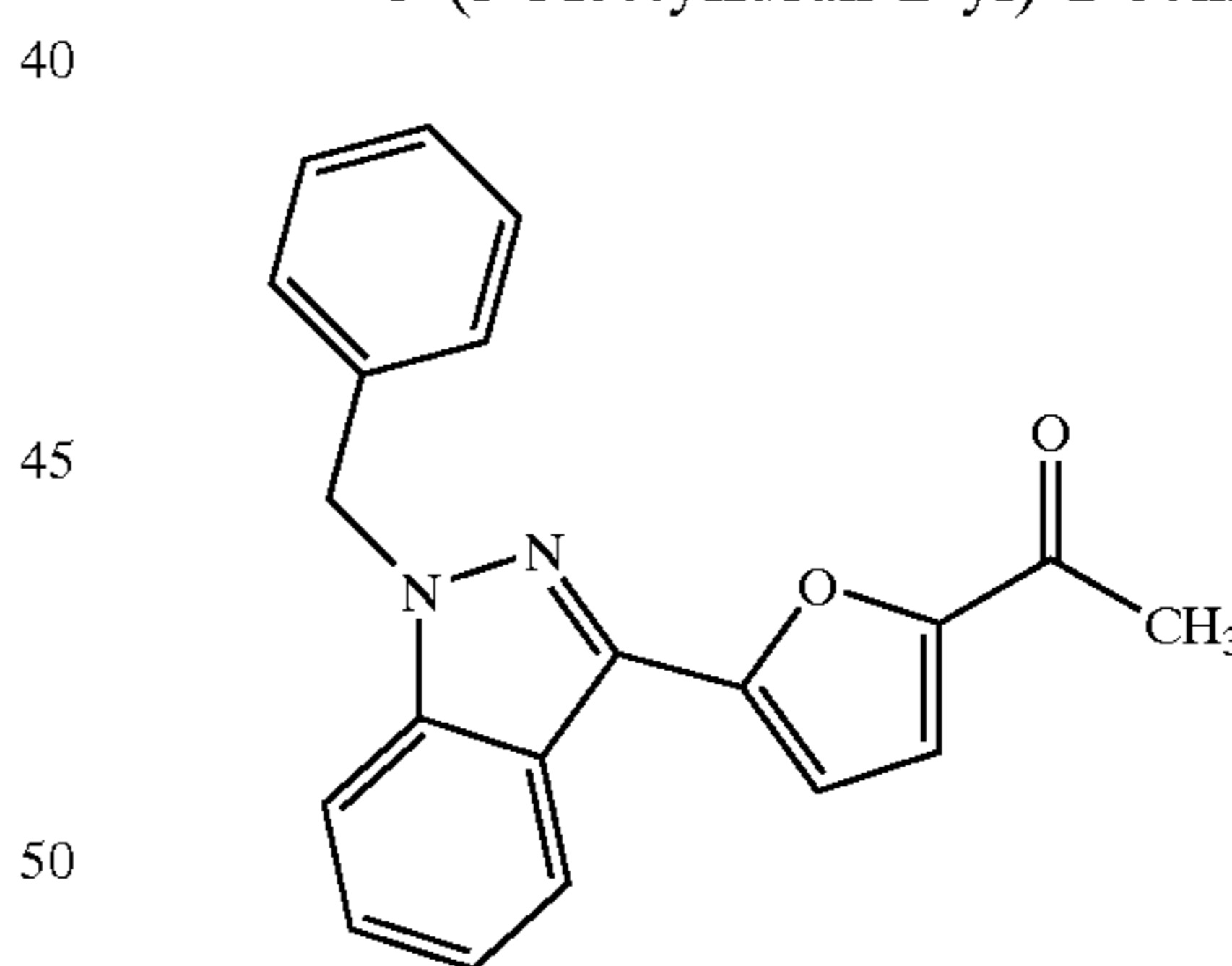
3-(5-Acetylfuran-2-yl)-1-benzyl-indazole
