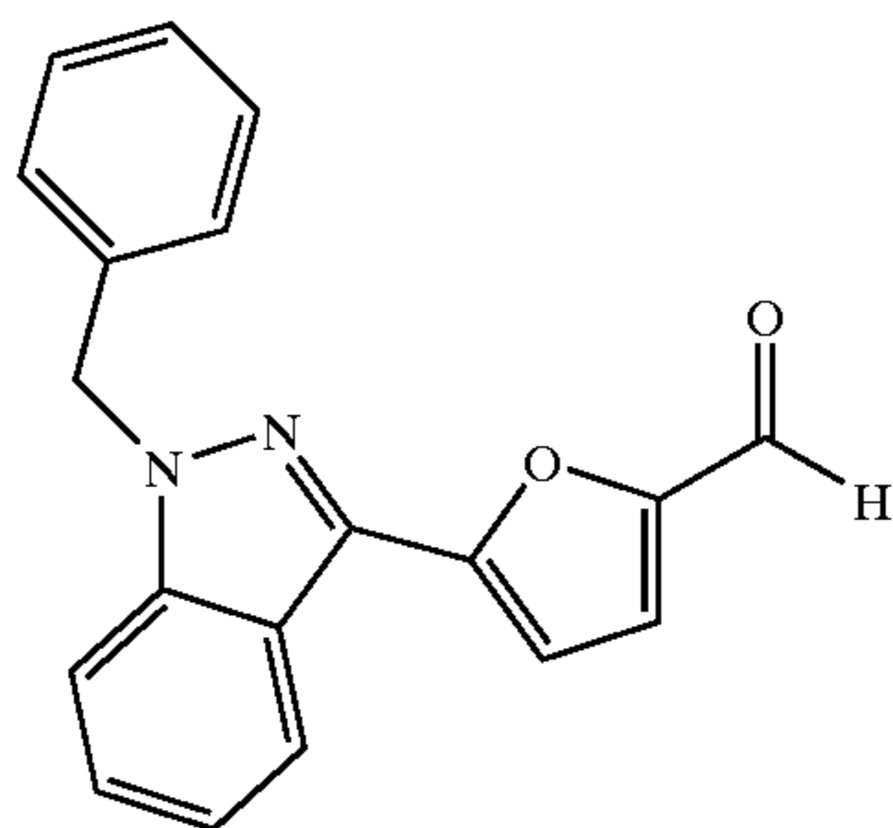
1-Benzyl-3-(5-formylfuran-2-yl)-indazole
