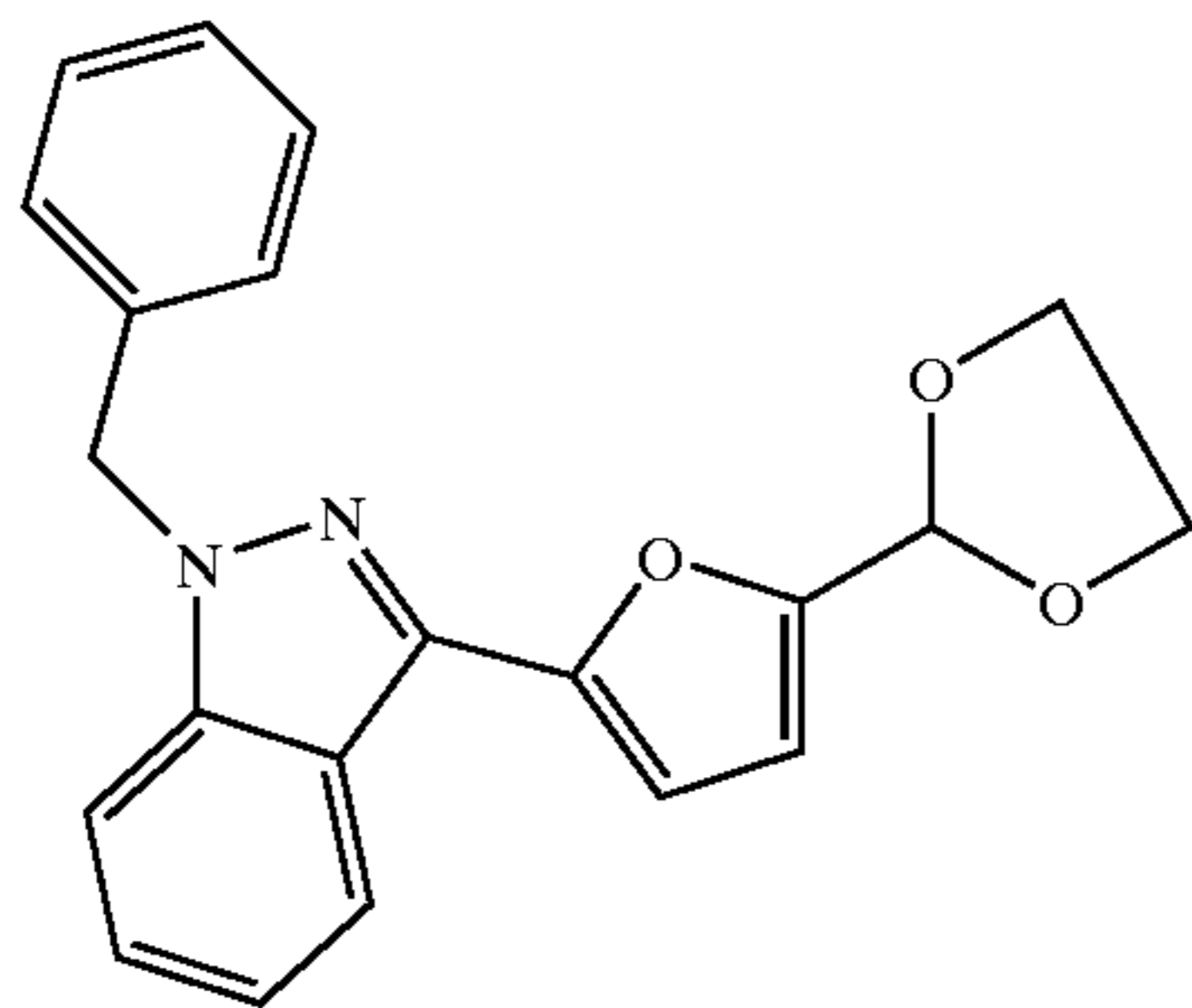
1-Benzyl-3-[5-(1,3-dioxolan-2-yl)-furan-2-yl]-indazole
