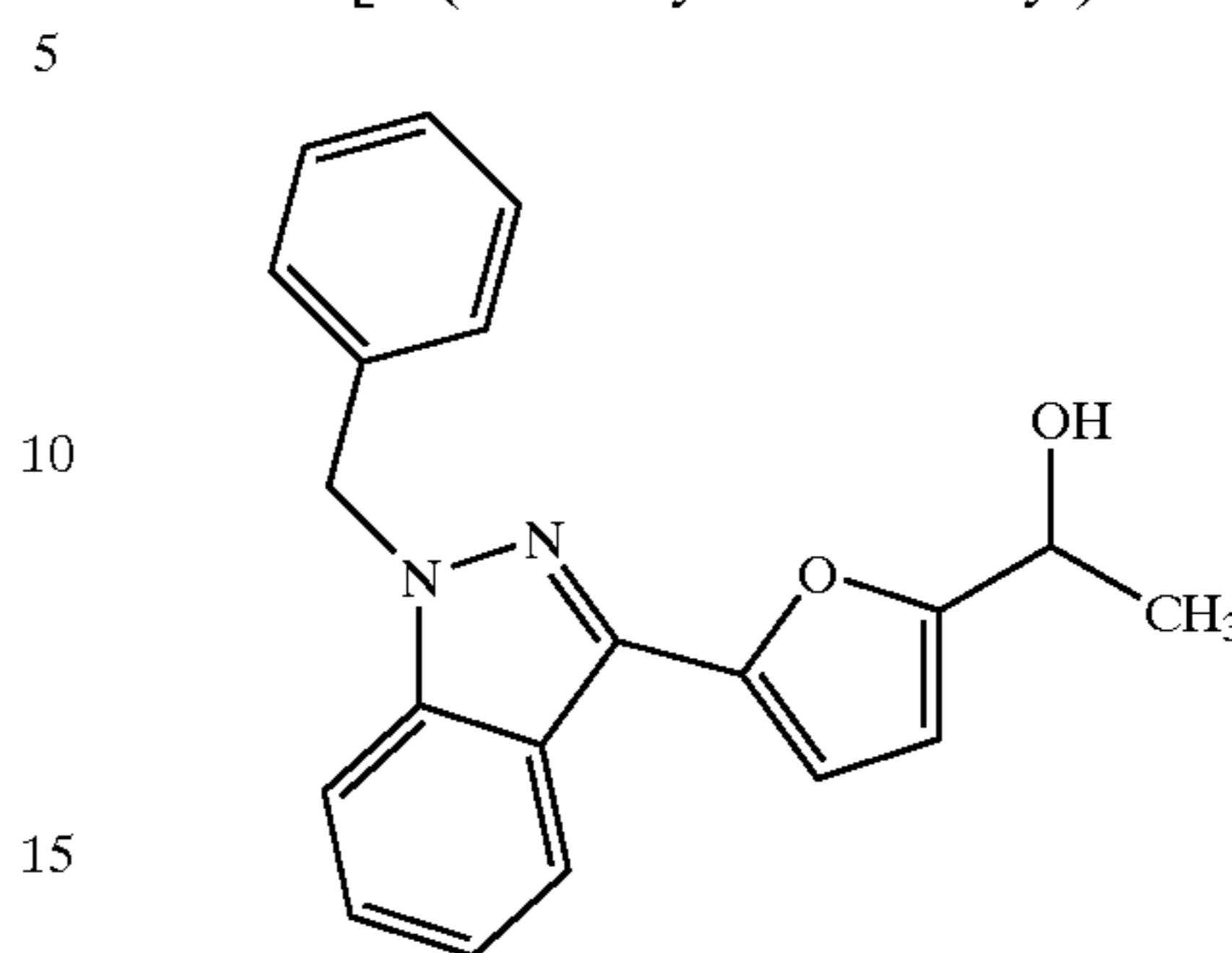
1-[5-(1-Benzylindazol-3-yl)-furan-2-yl]-ethanol
