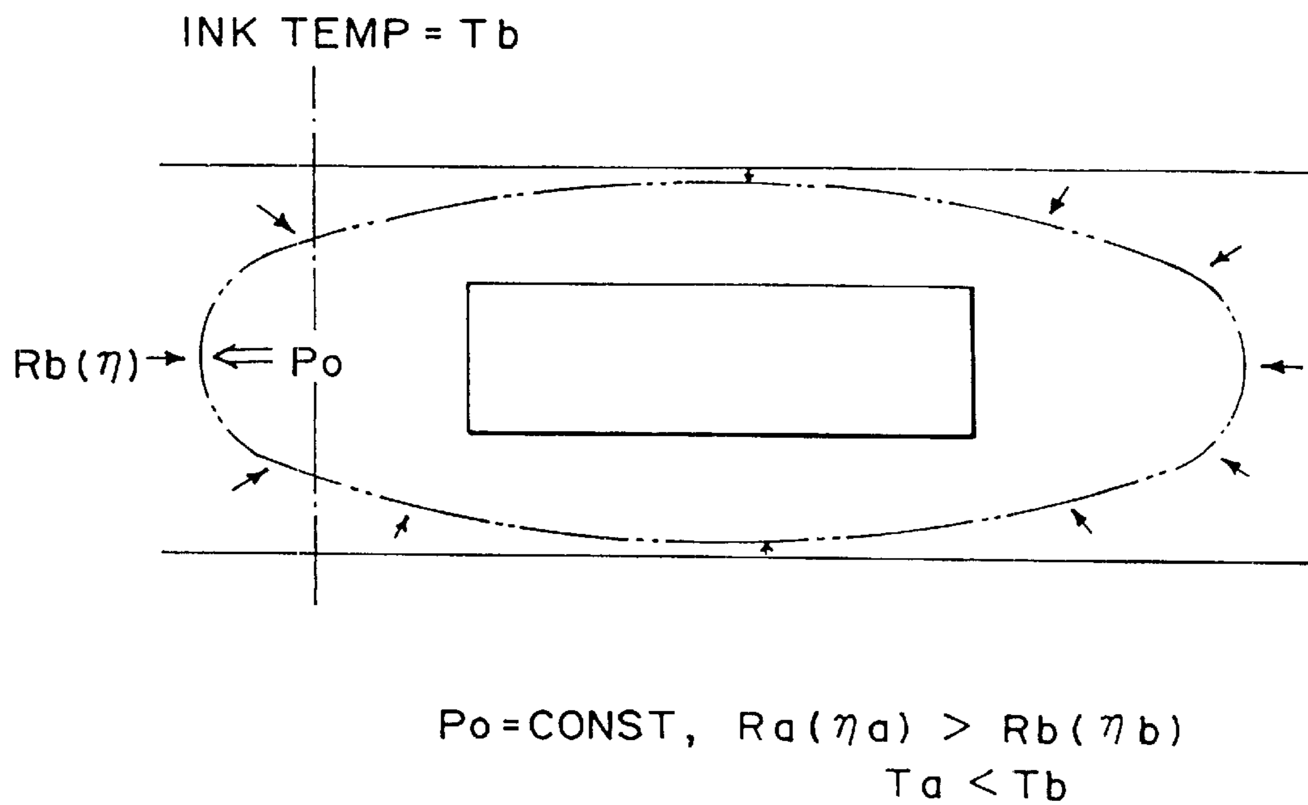
FIG. 6(B)
