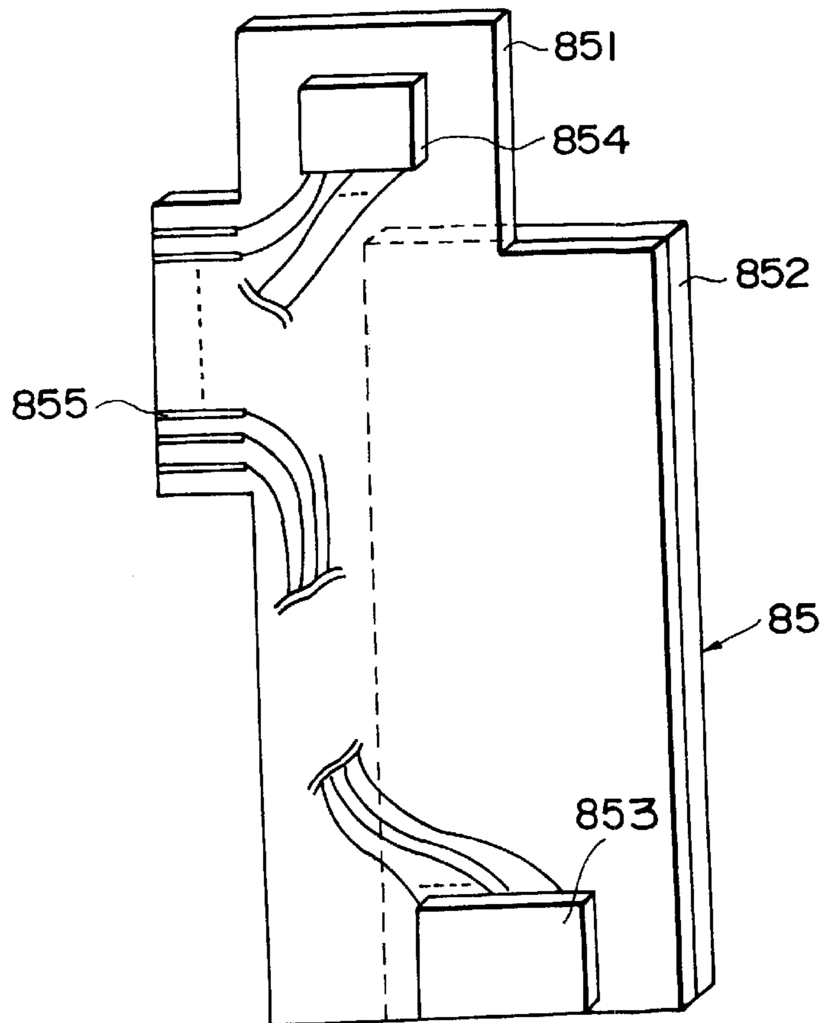
FIG. 32A
