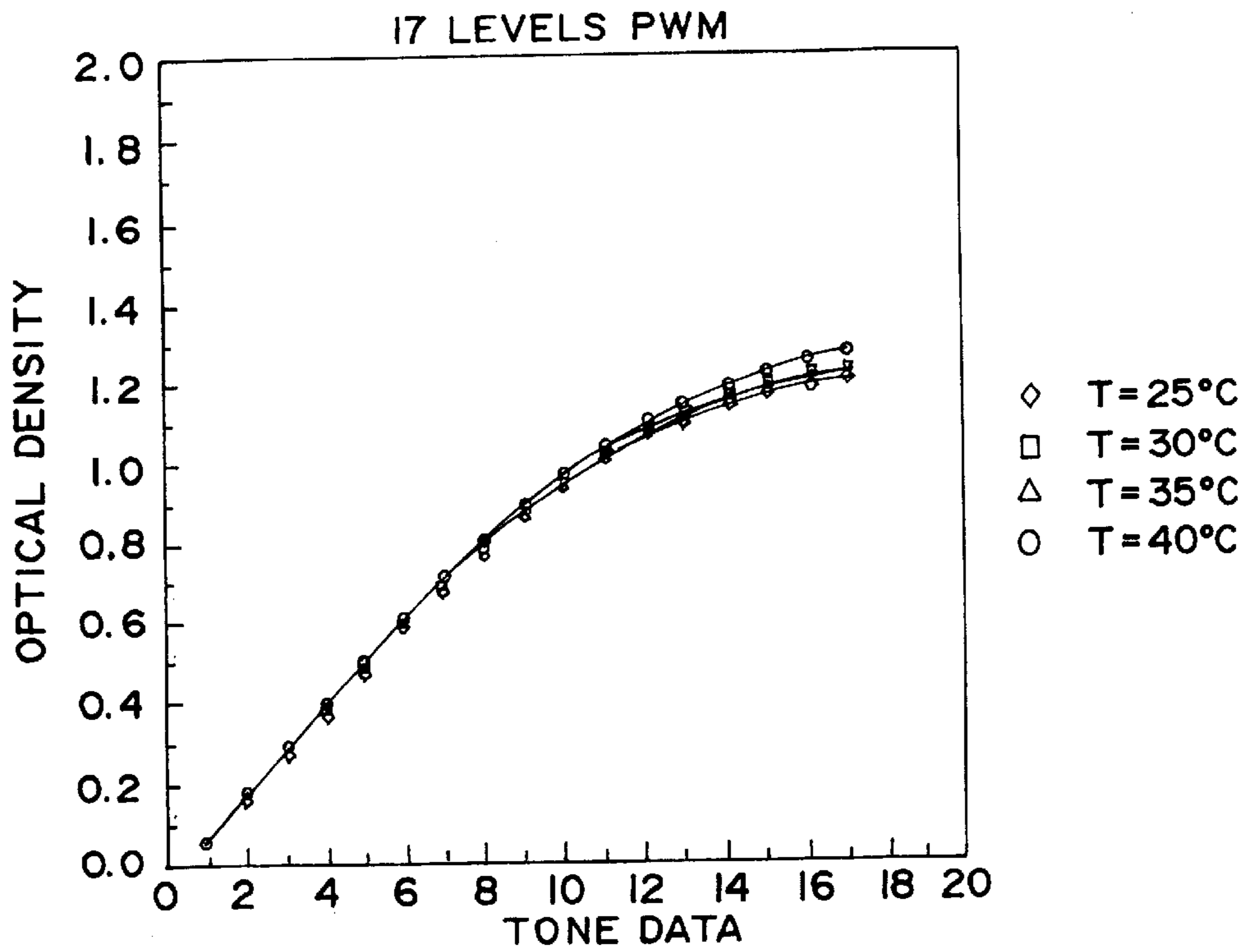
FIG. 17A
