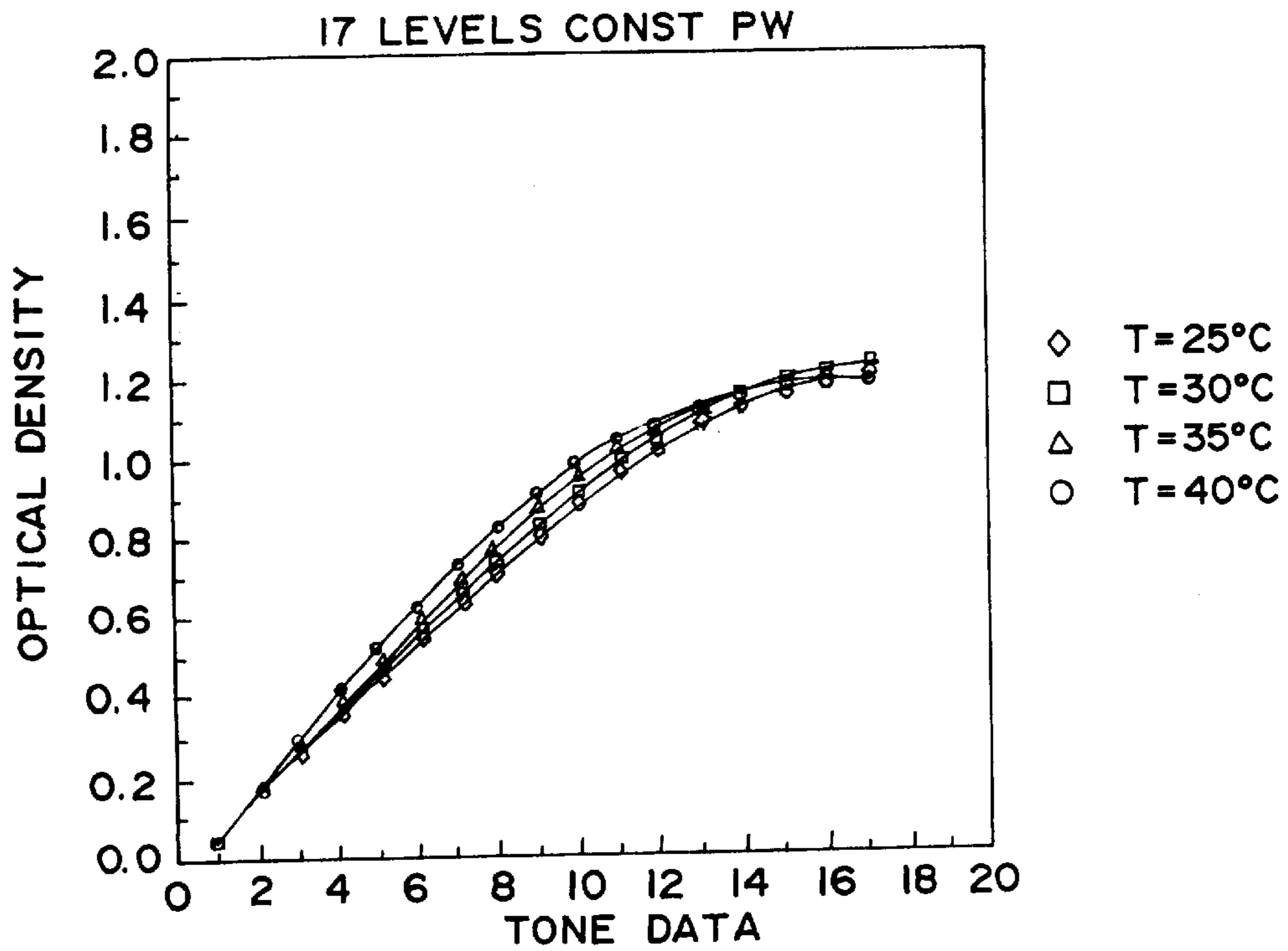
FIG. 17B
