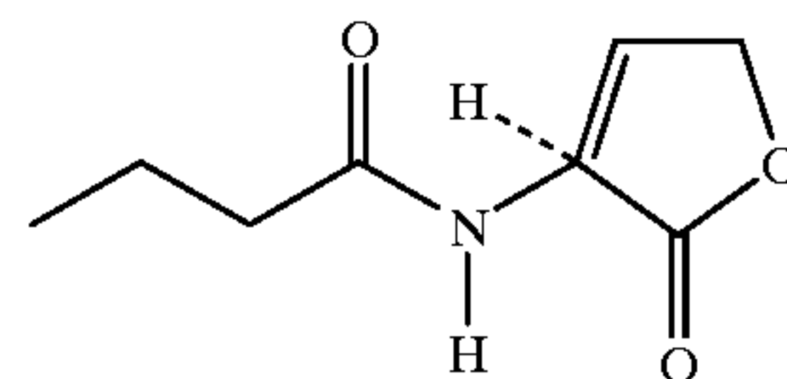
N(3-oxododecanoyl)-L-homoserine Lactone (OdDHL)
