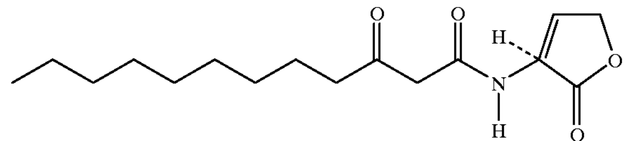
N(3-oxododecanoyl)-L-homoserine Lactone (OdDHL)
