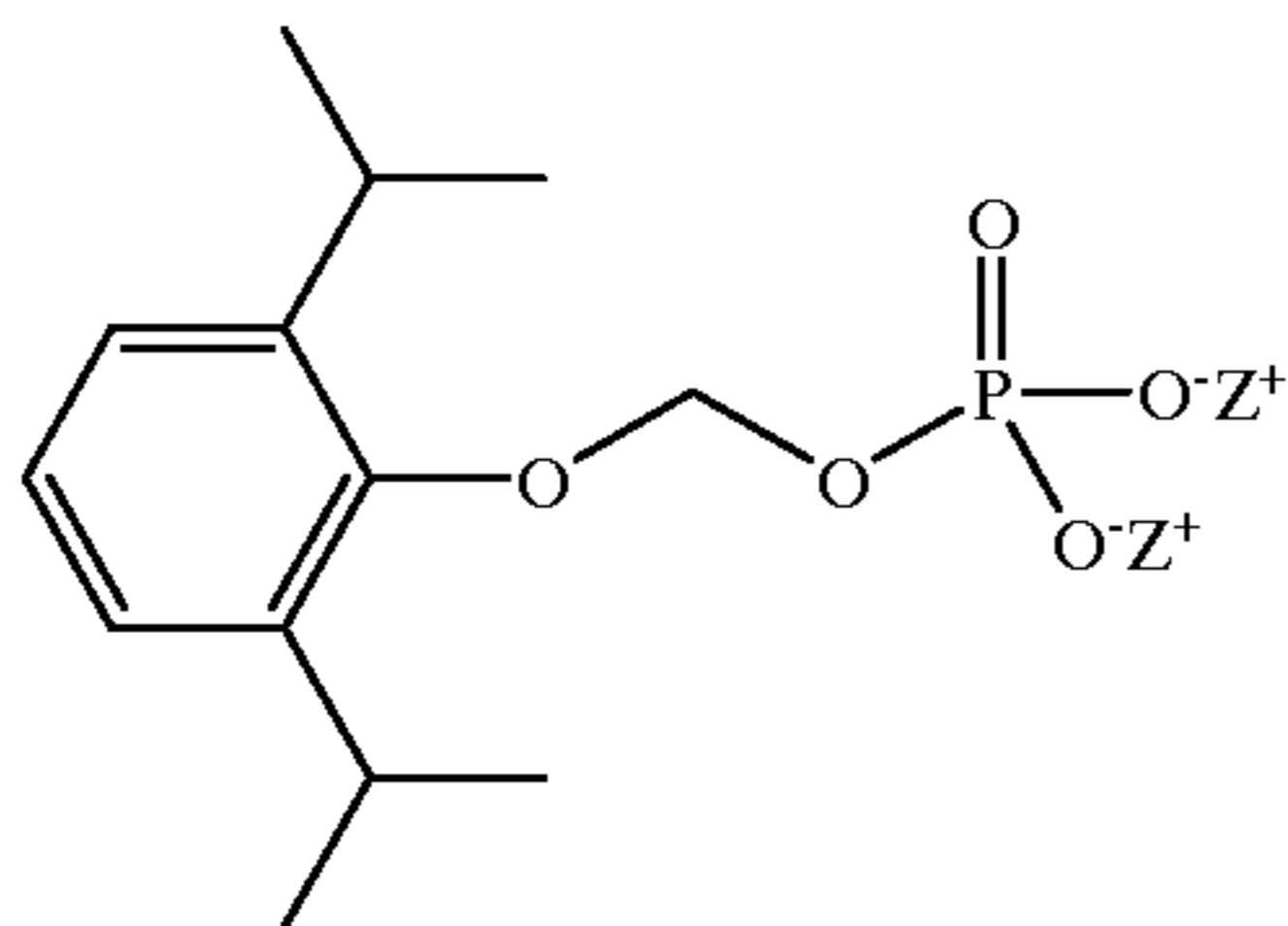
Propofol Prodrug
