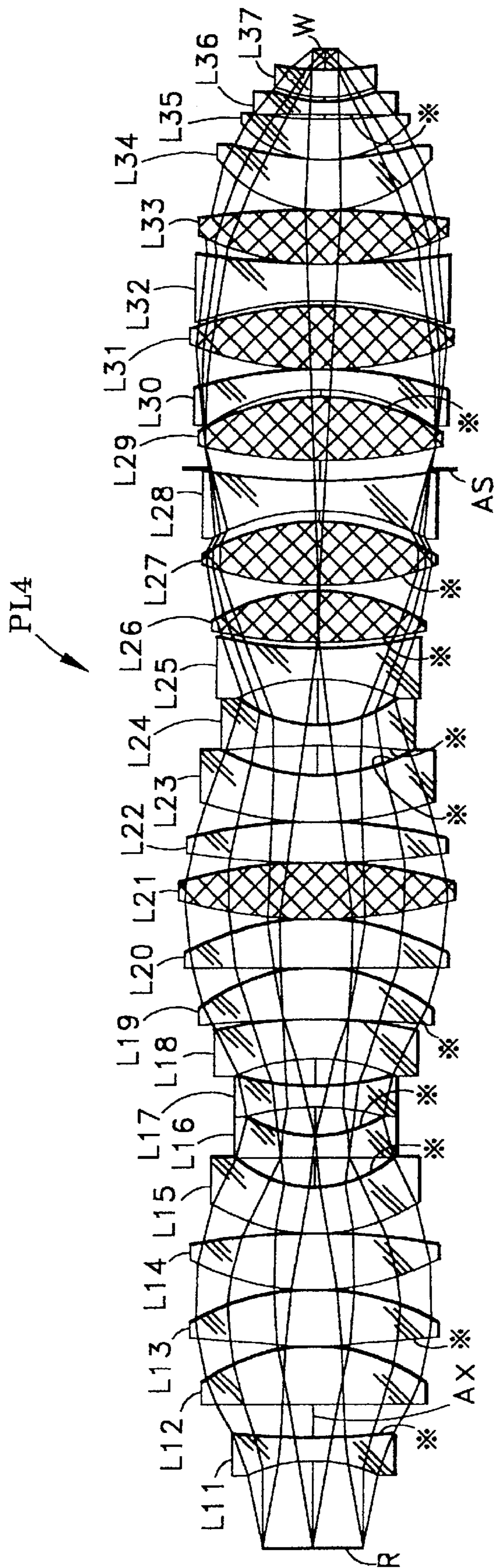
FIG. 11A
