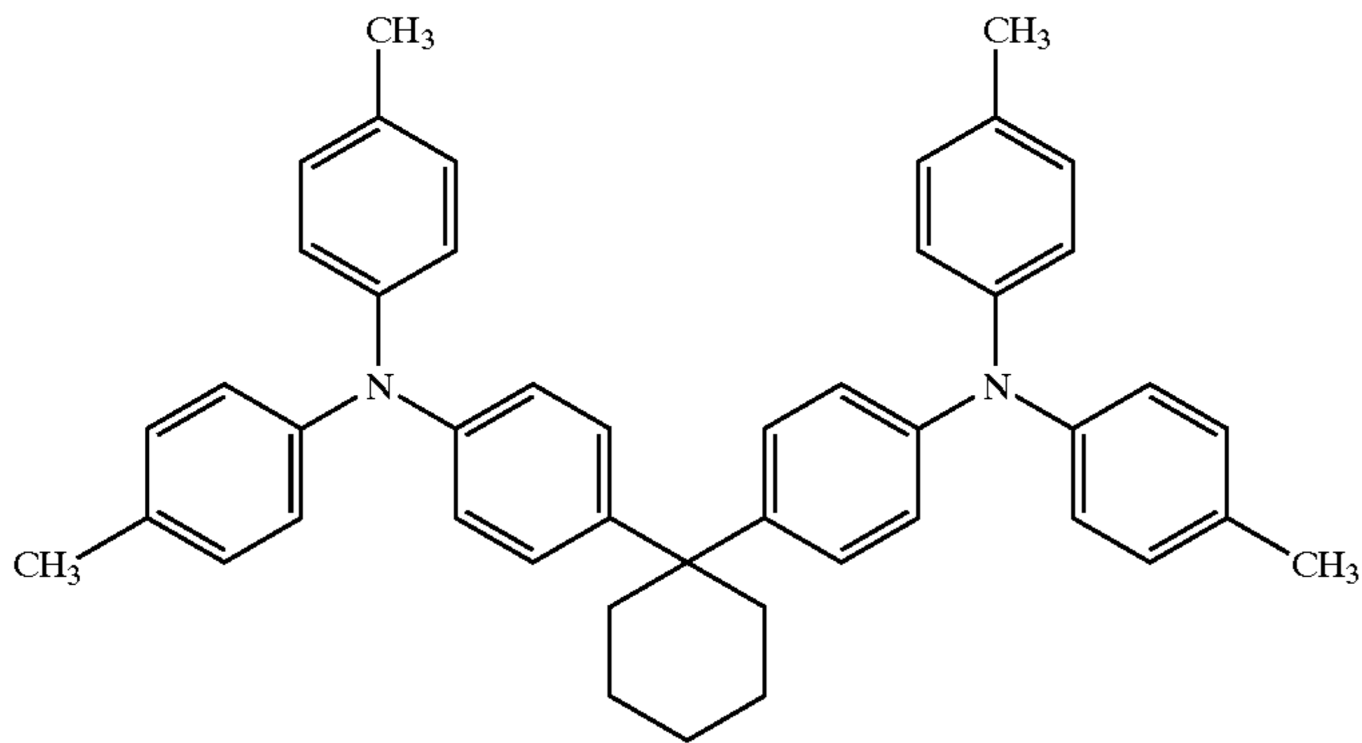
DIAMINE
