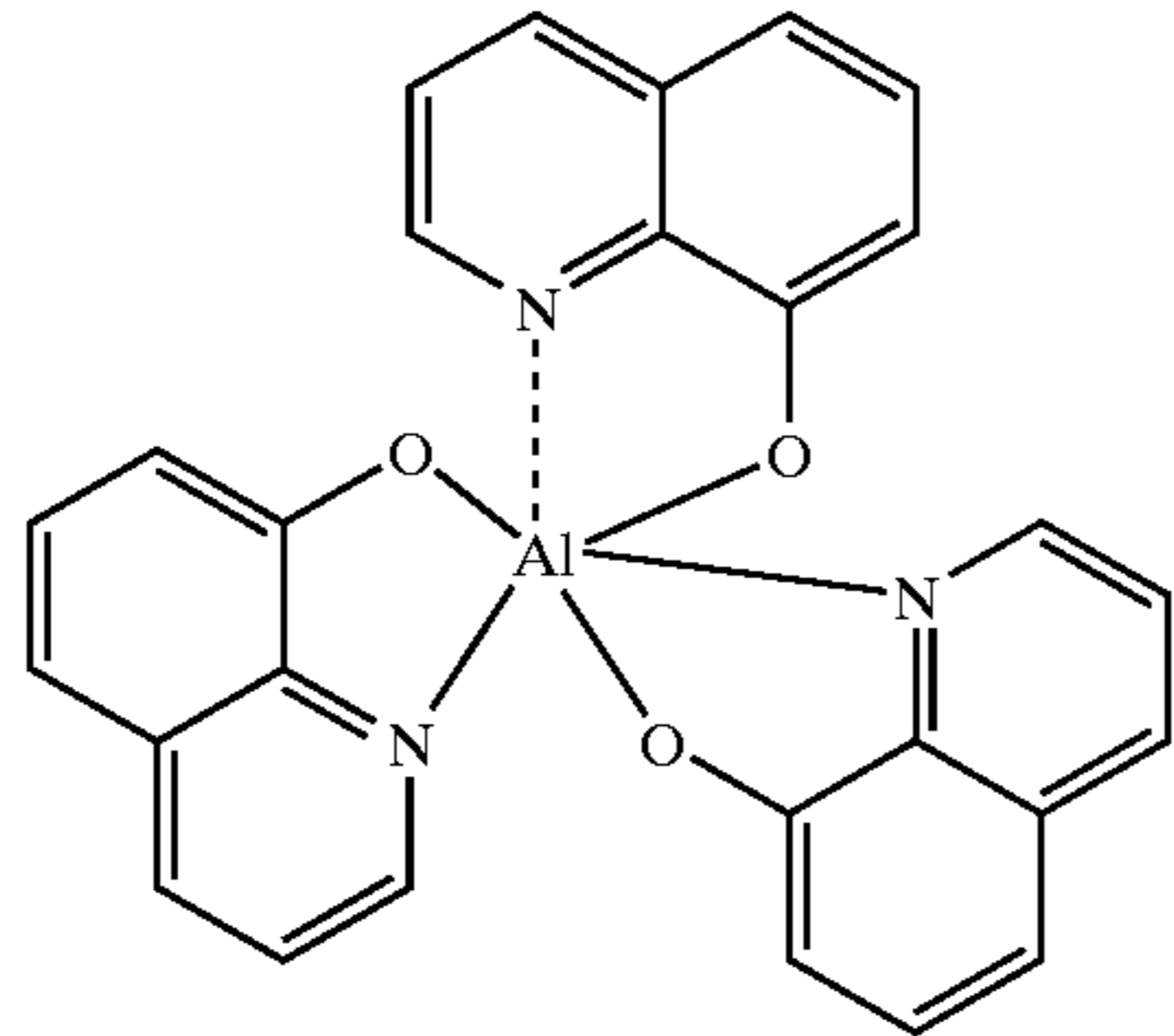
Alq 3
