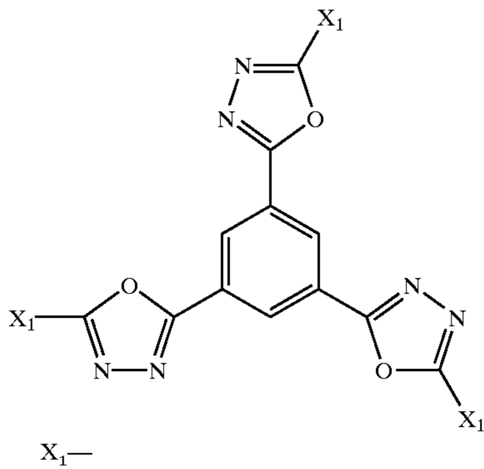
DIAMINE
