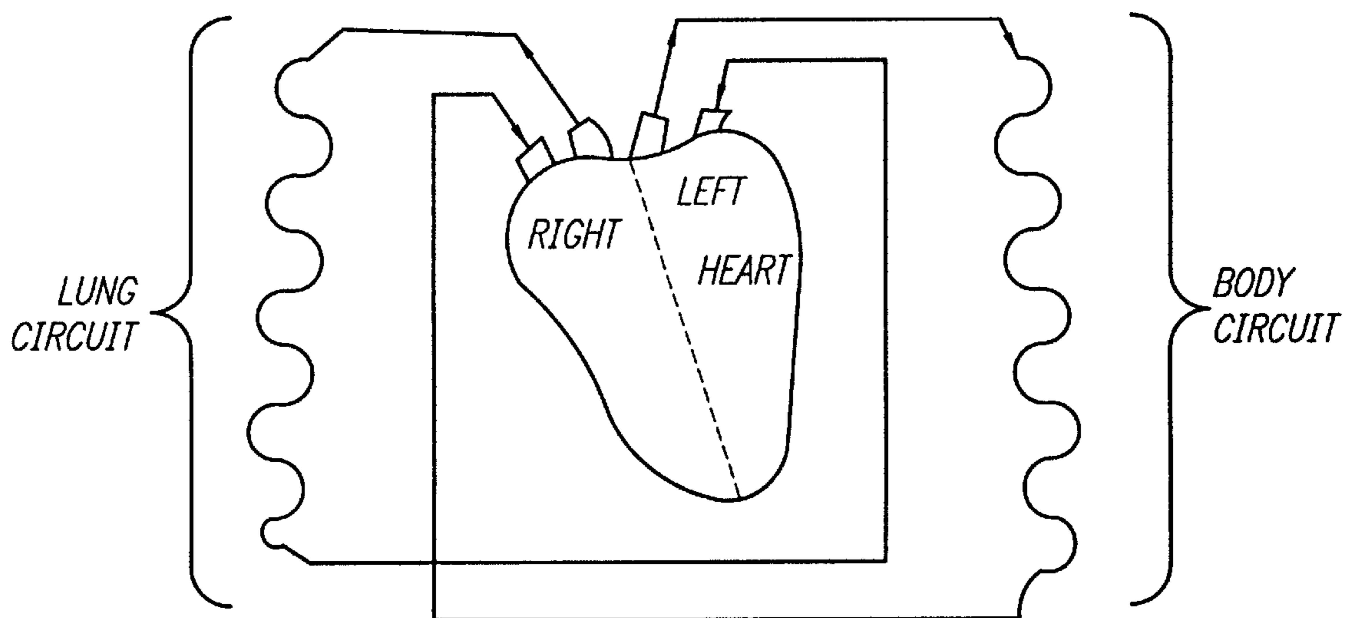
FIG. 1B
