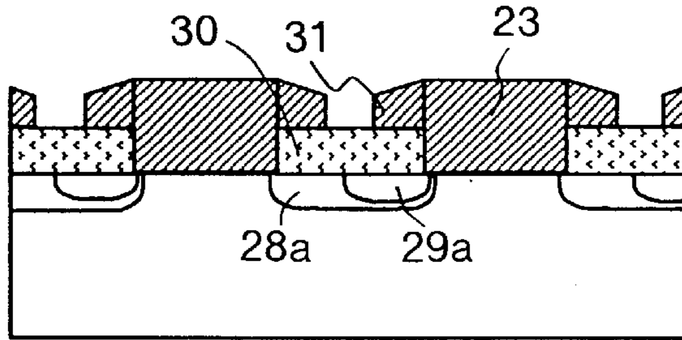
Fig. 14(f) Prior Art
