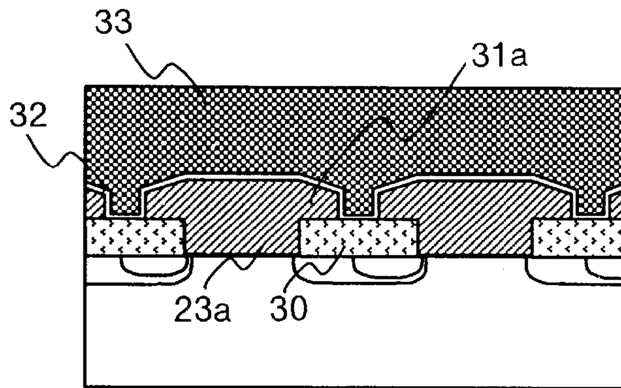
Fig. 14(g) Prior Art
