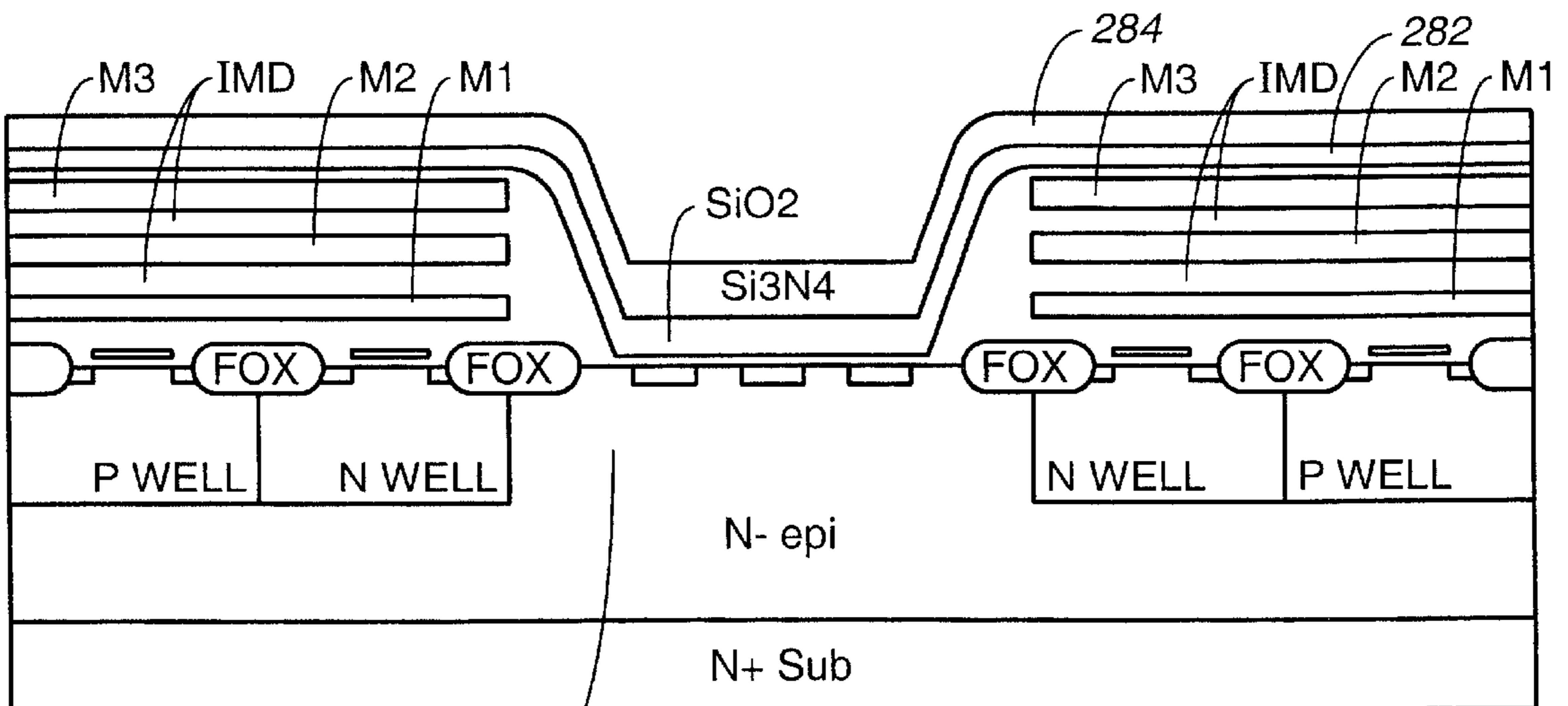
204a FIG. 26D
