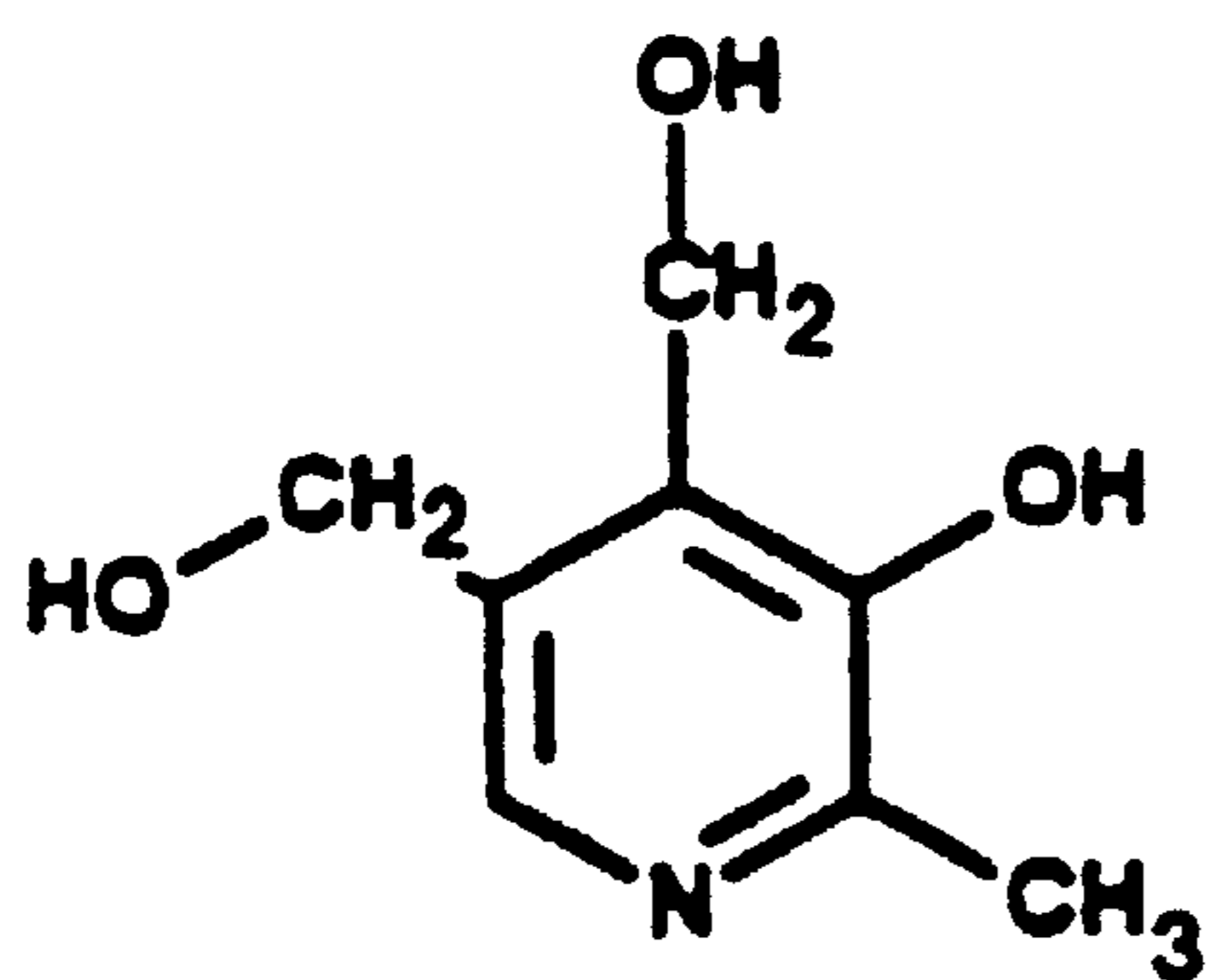
Pyridoxine
