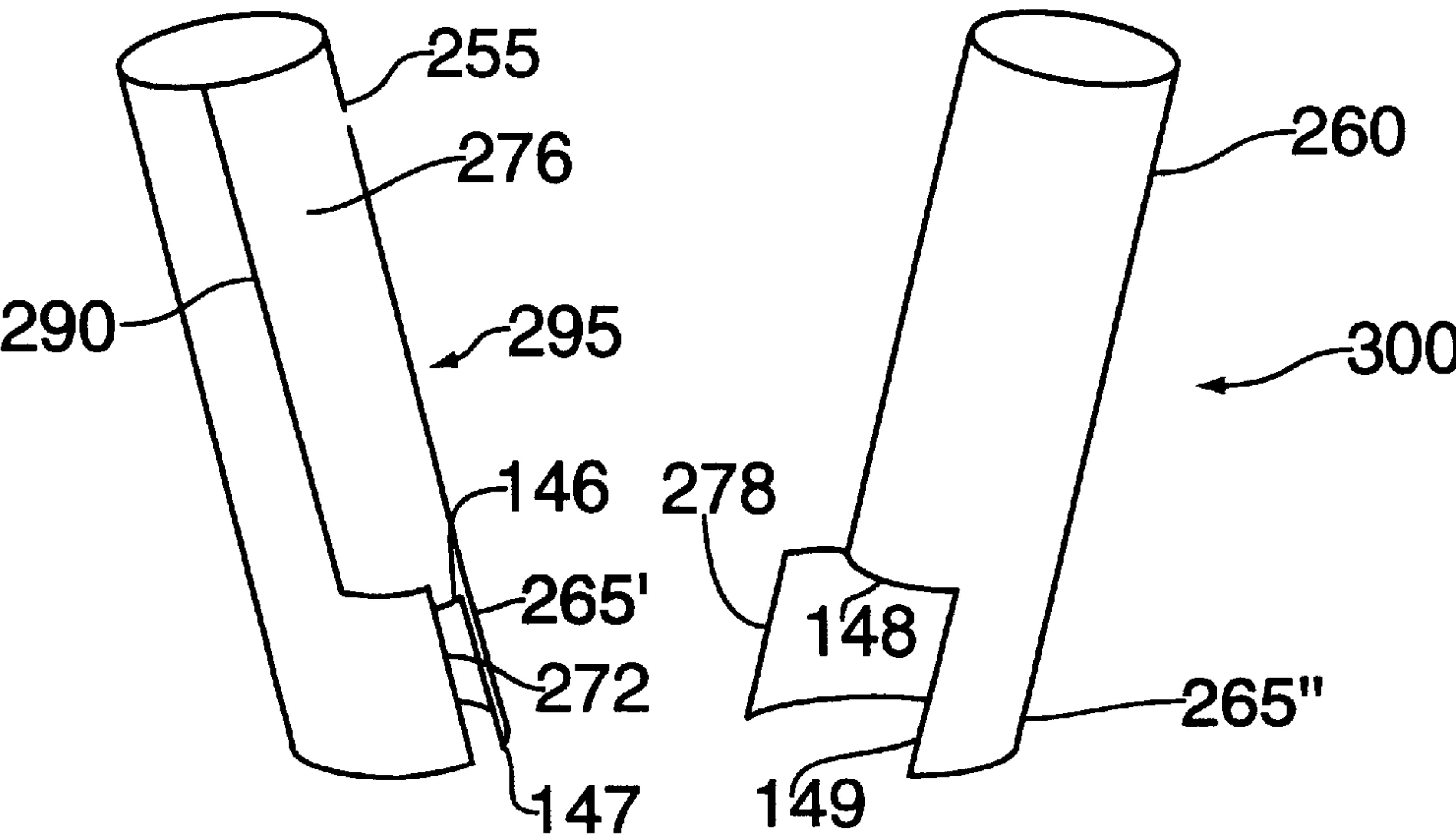
FIG. 10B
