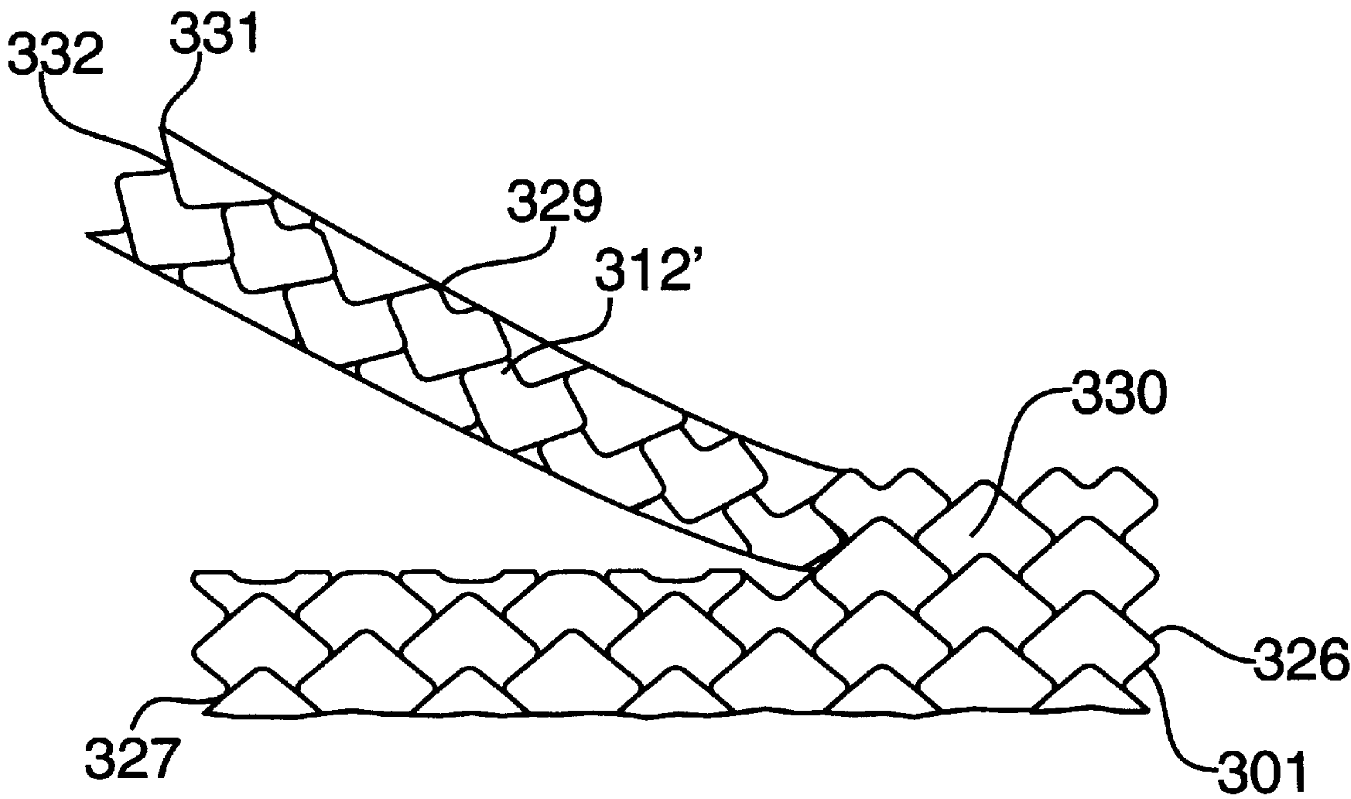
FIG. 27
