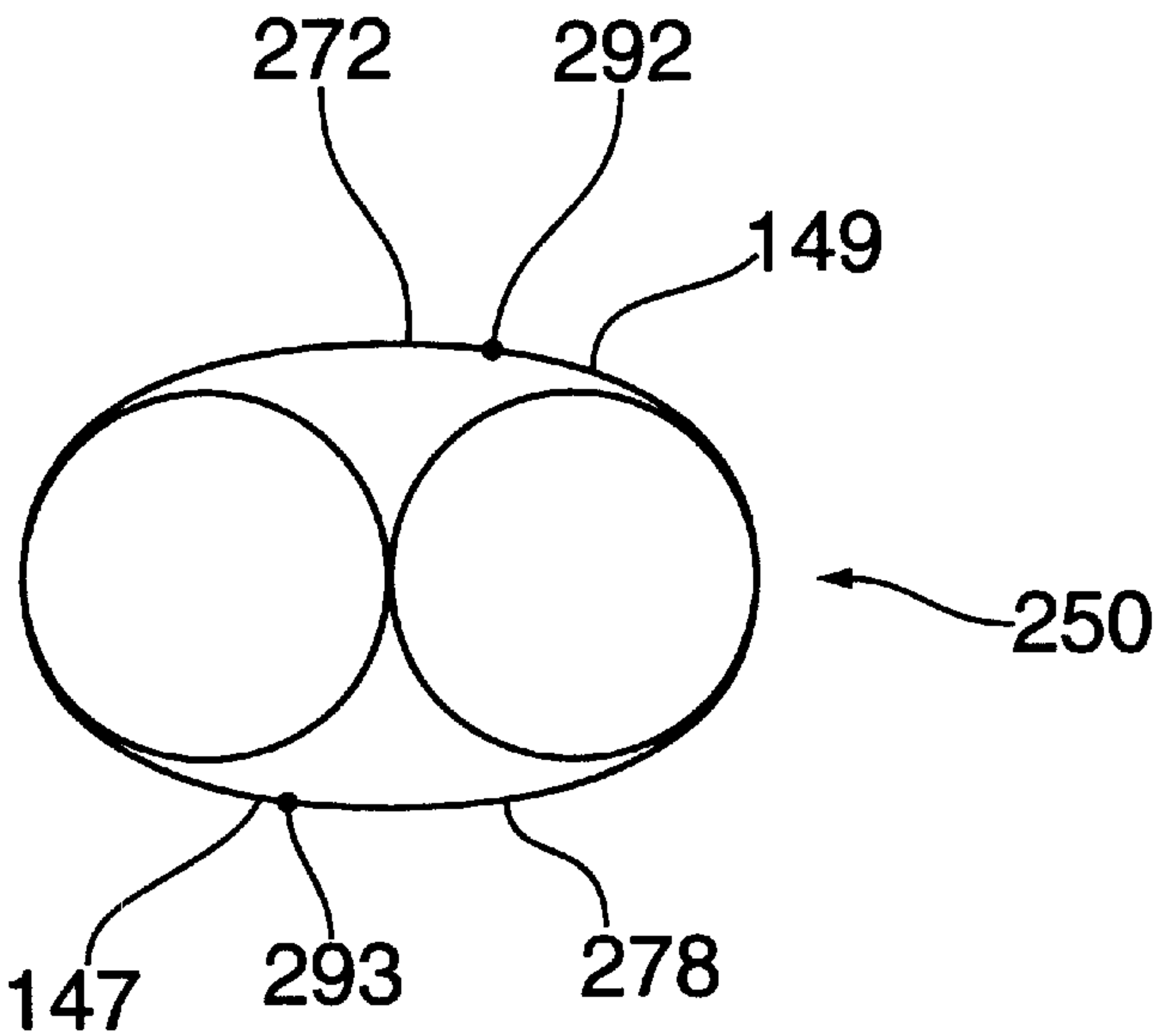
FIG. 12B
