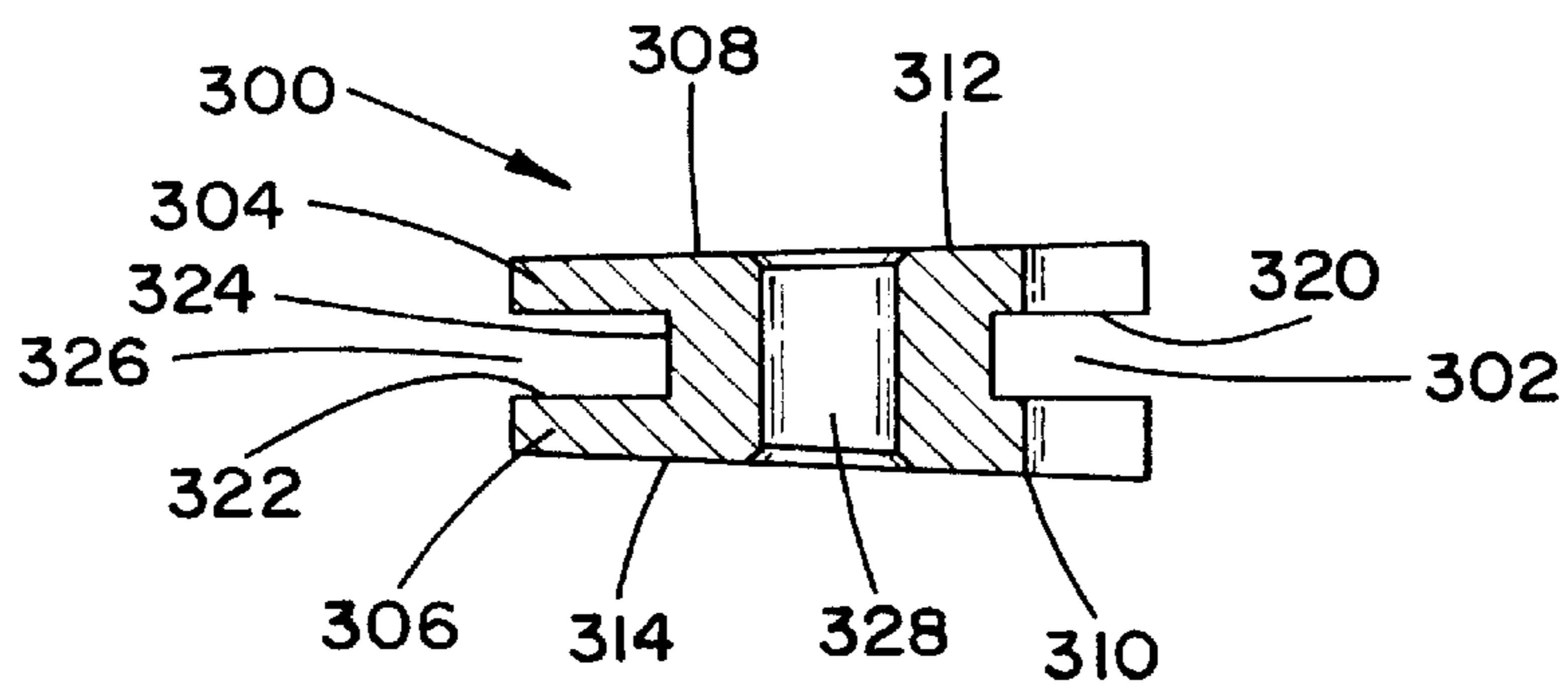
Section A-A FIG. 3c
