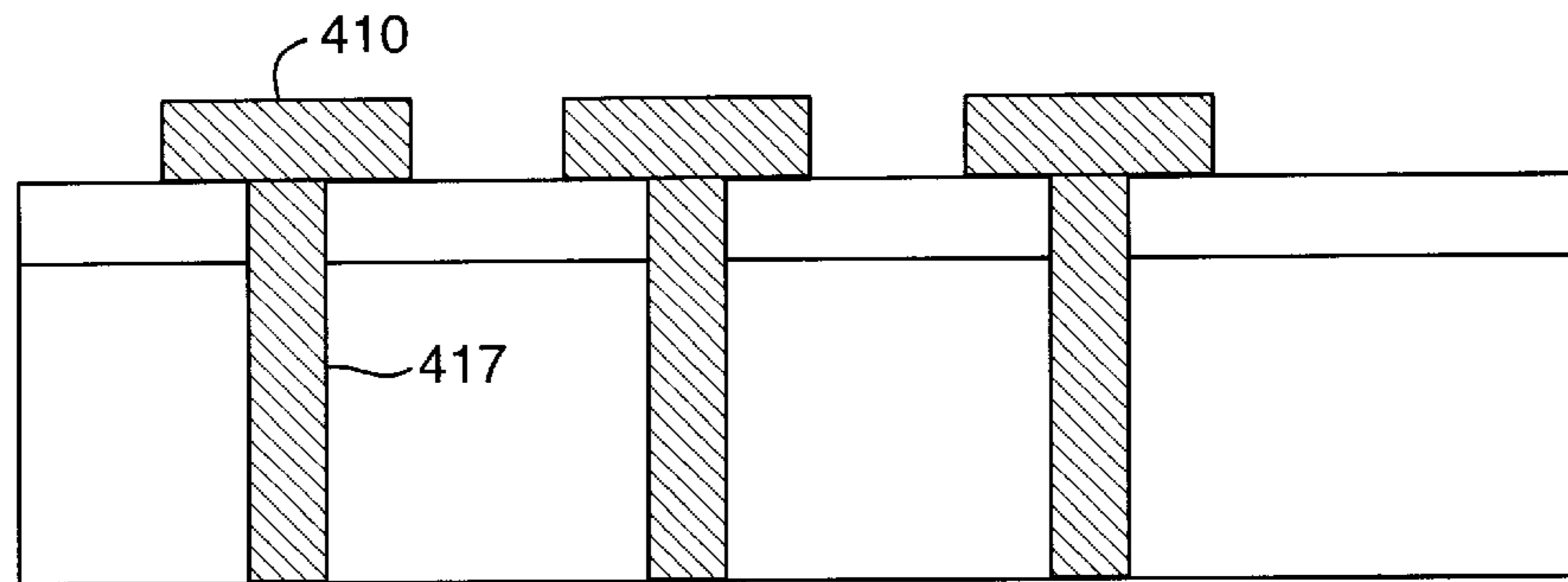
Fig. 4H
