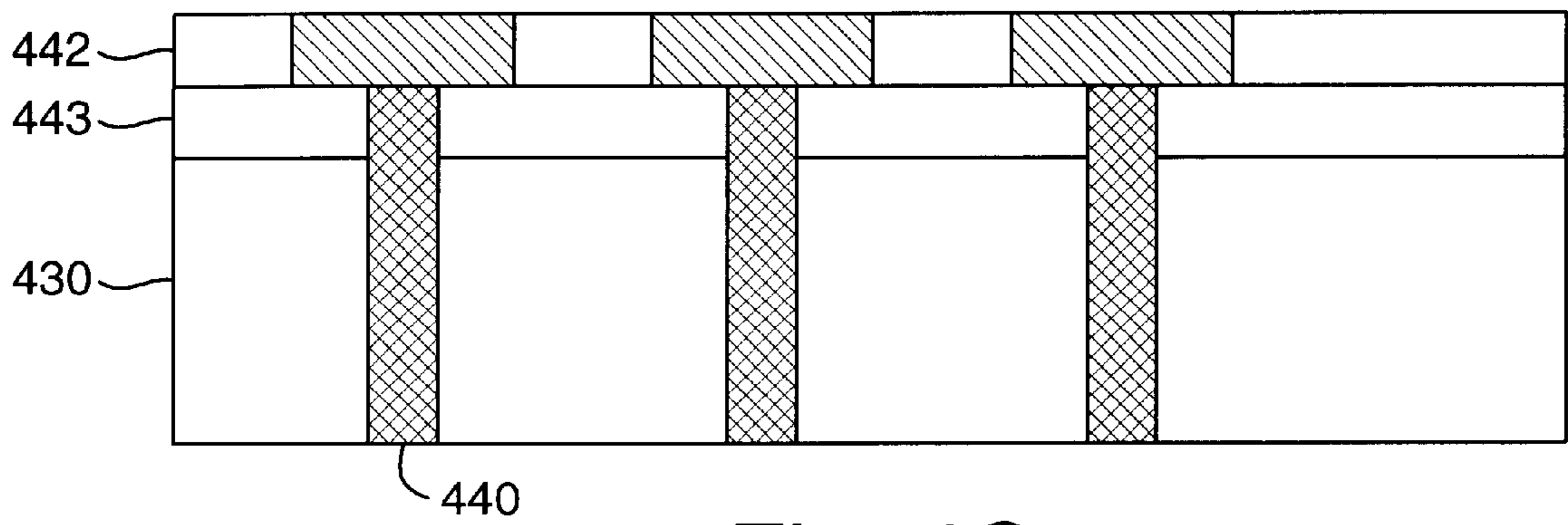
Fig. 4G
