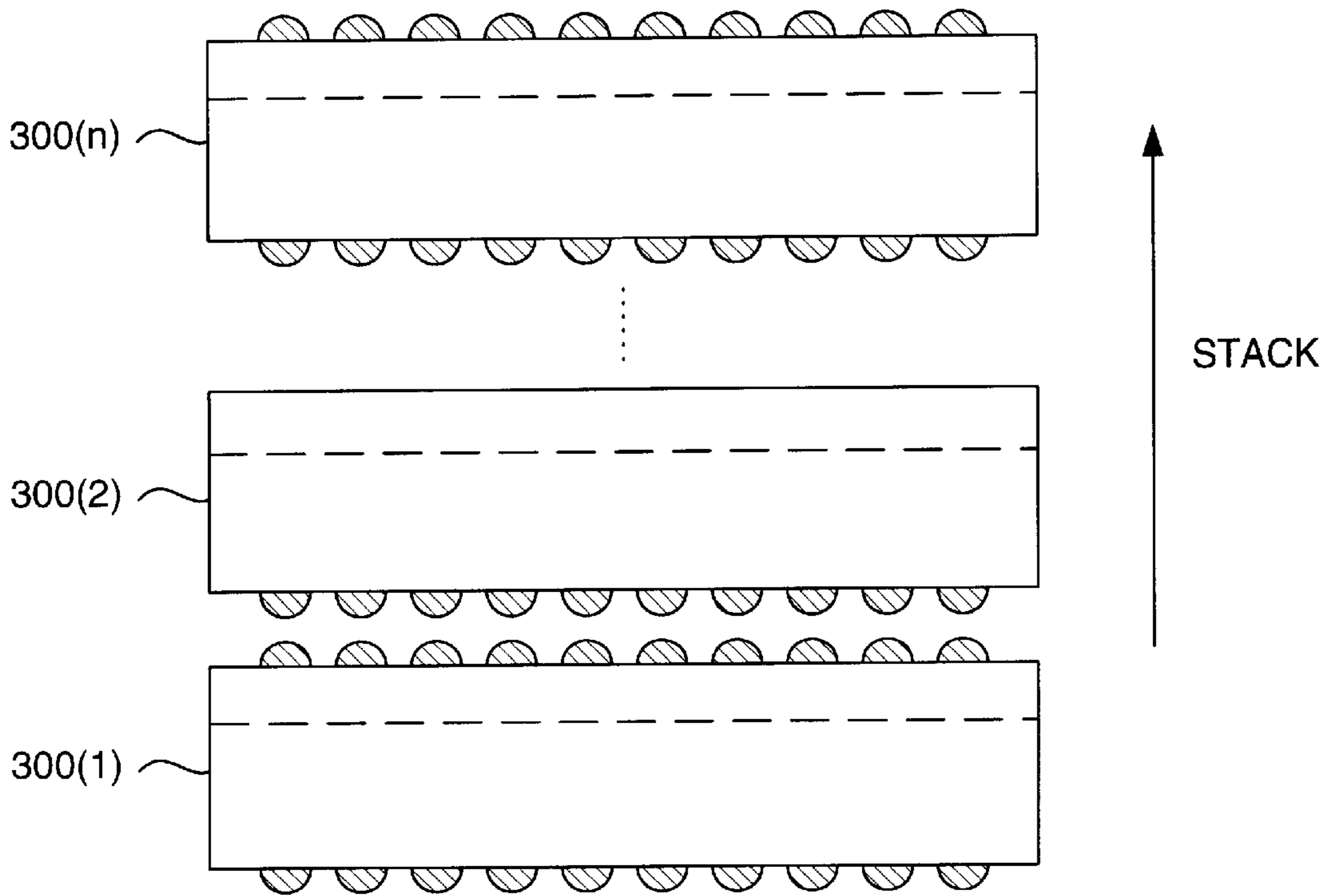
Fig. 3C
