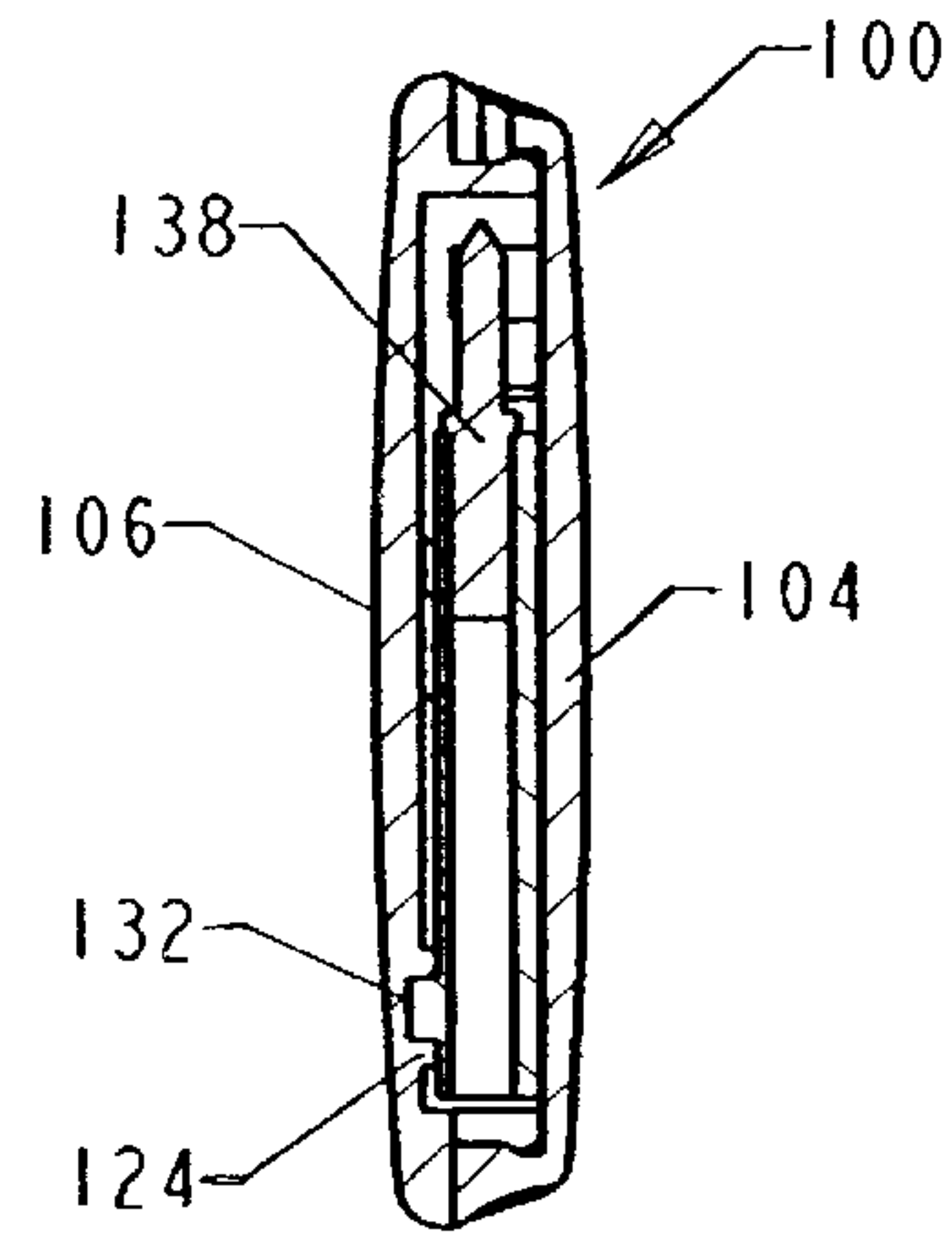
SECTION A-A
