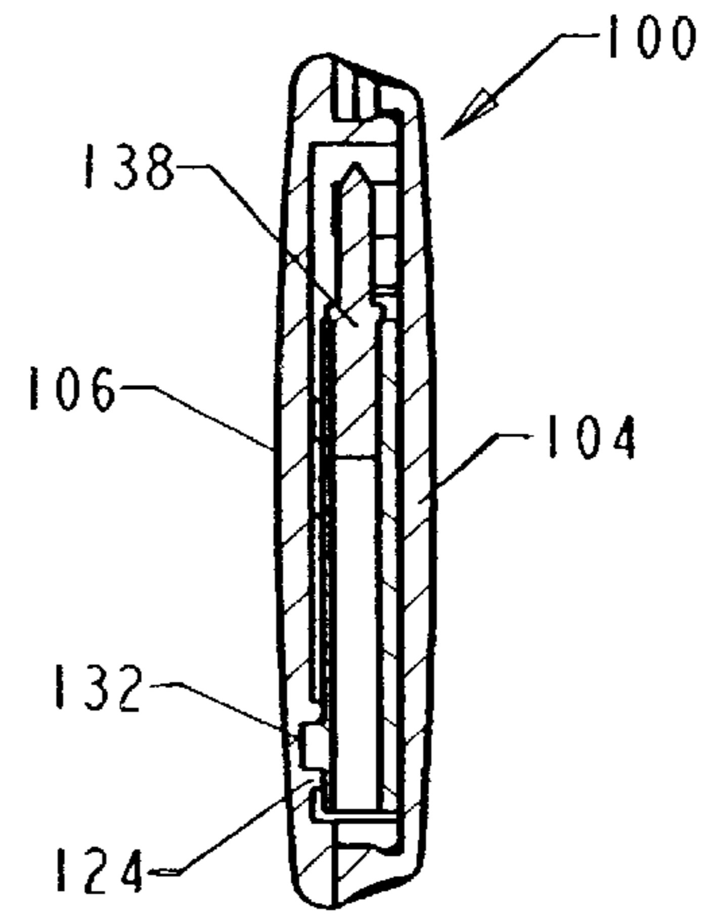
SECTION A-A
