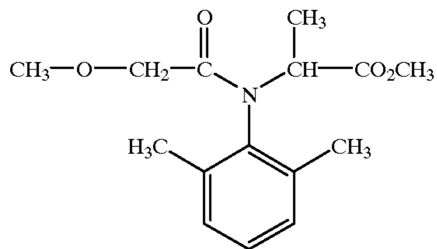
(METALAXYL)
