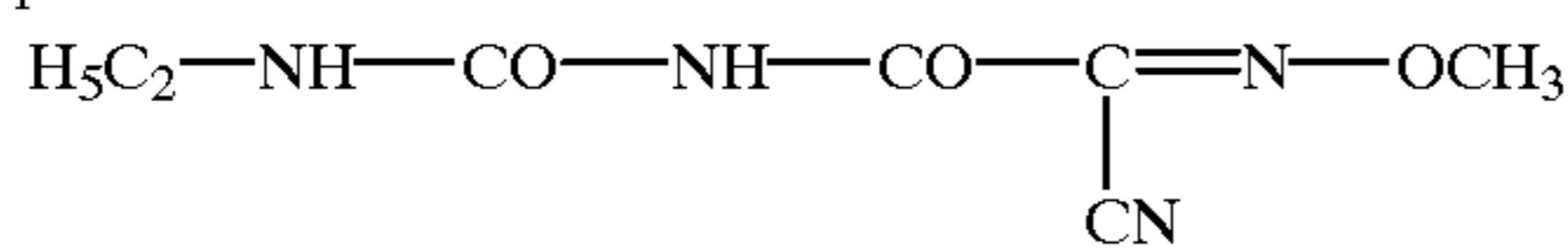
(CYMOXANILE)
