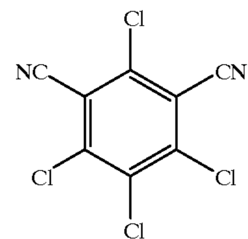
(CHLOROTHALONIL)
