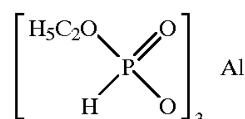
(FOSETYL AL)
