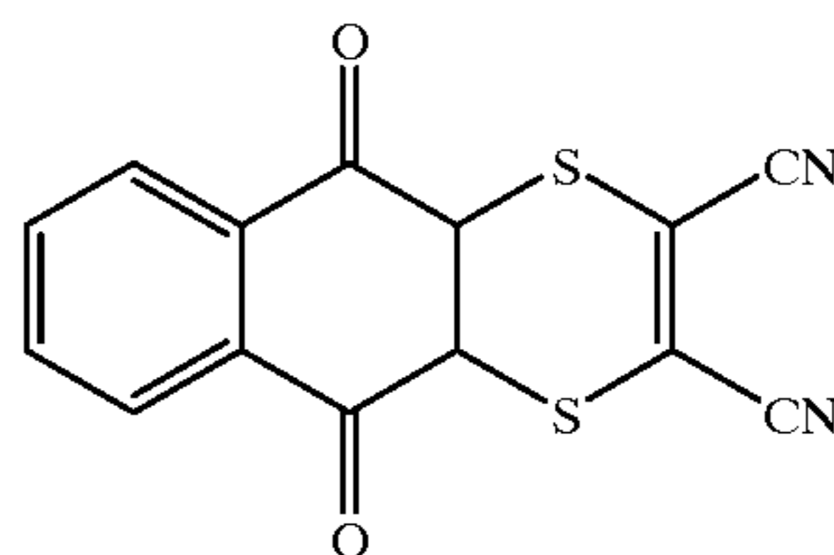
(DITHIANON)
