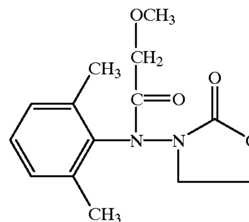
(OXADIXYL)
