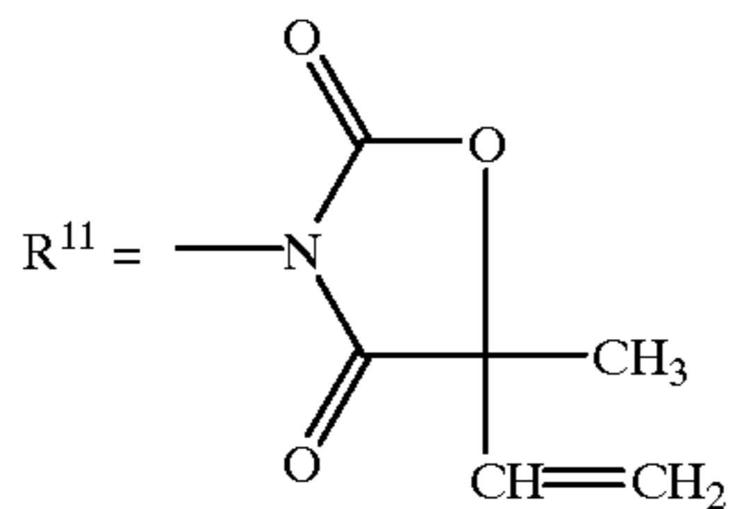
(VINCLOZOLIN)
