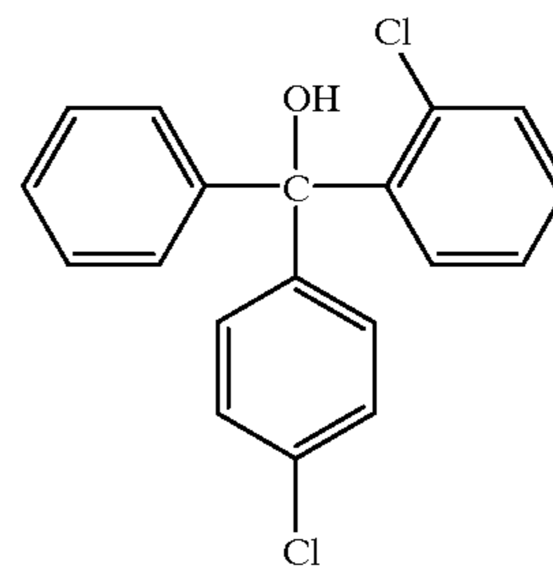
(FENARIMOL)
