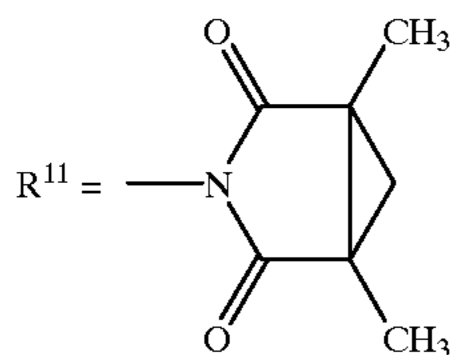
(PROCYMIDONE)
