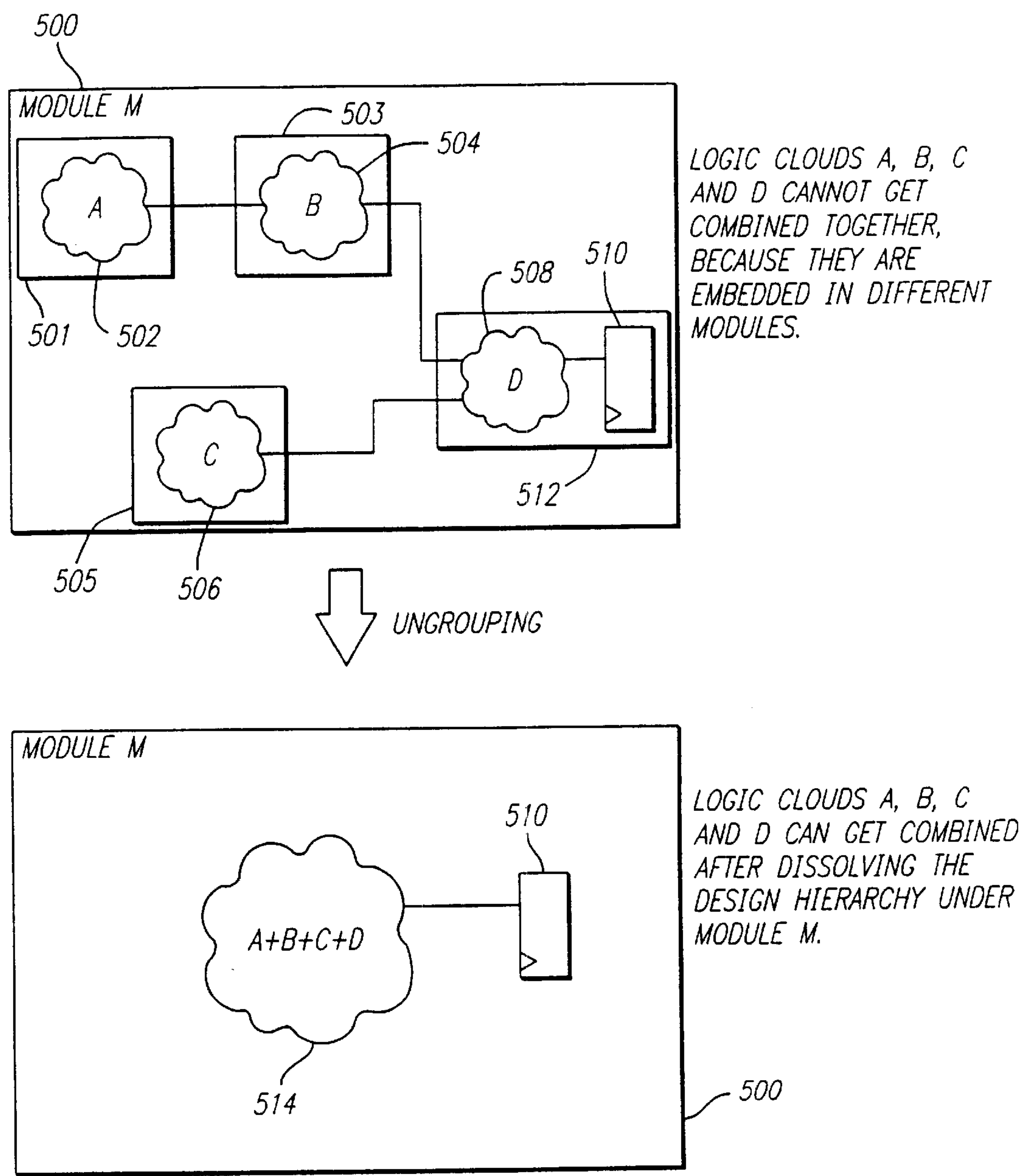
FIG. 22 HIERARCHY UNGROUPING
