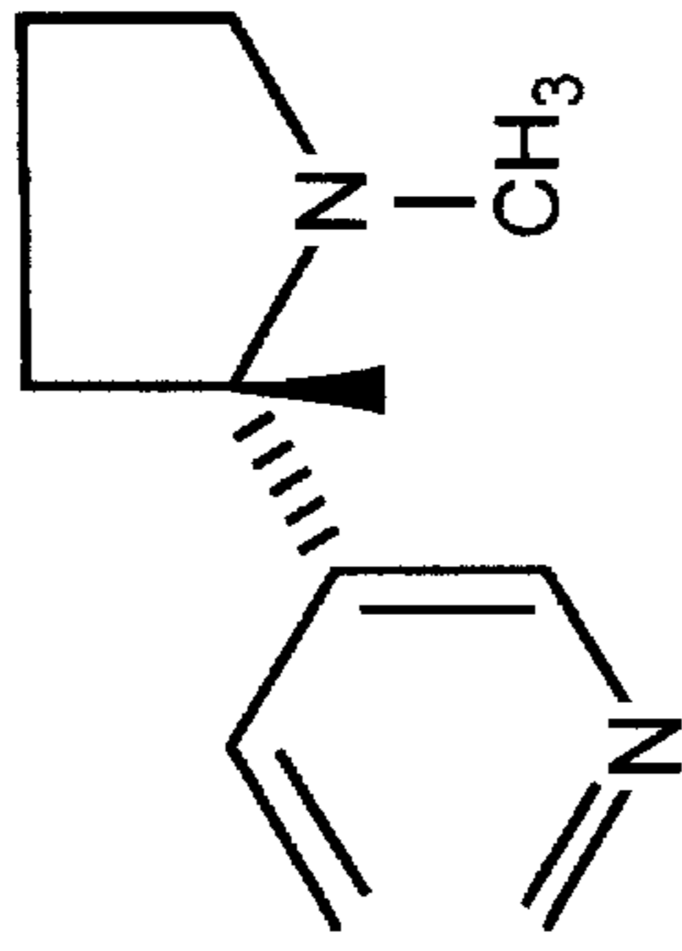
Nicotine
