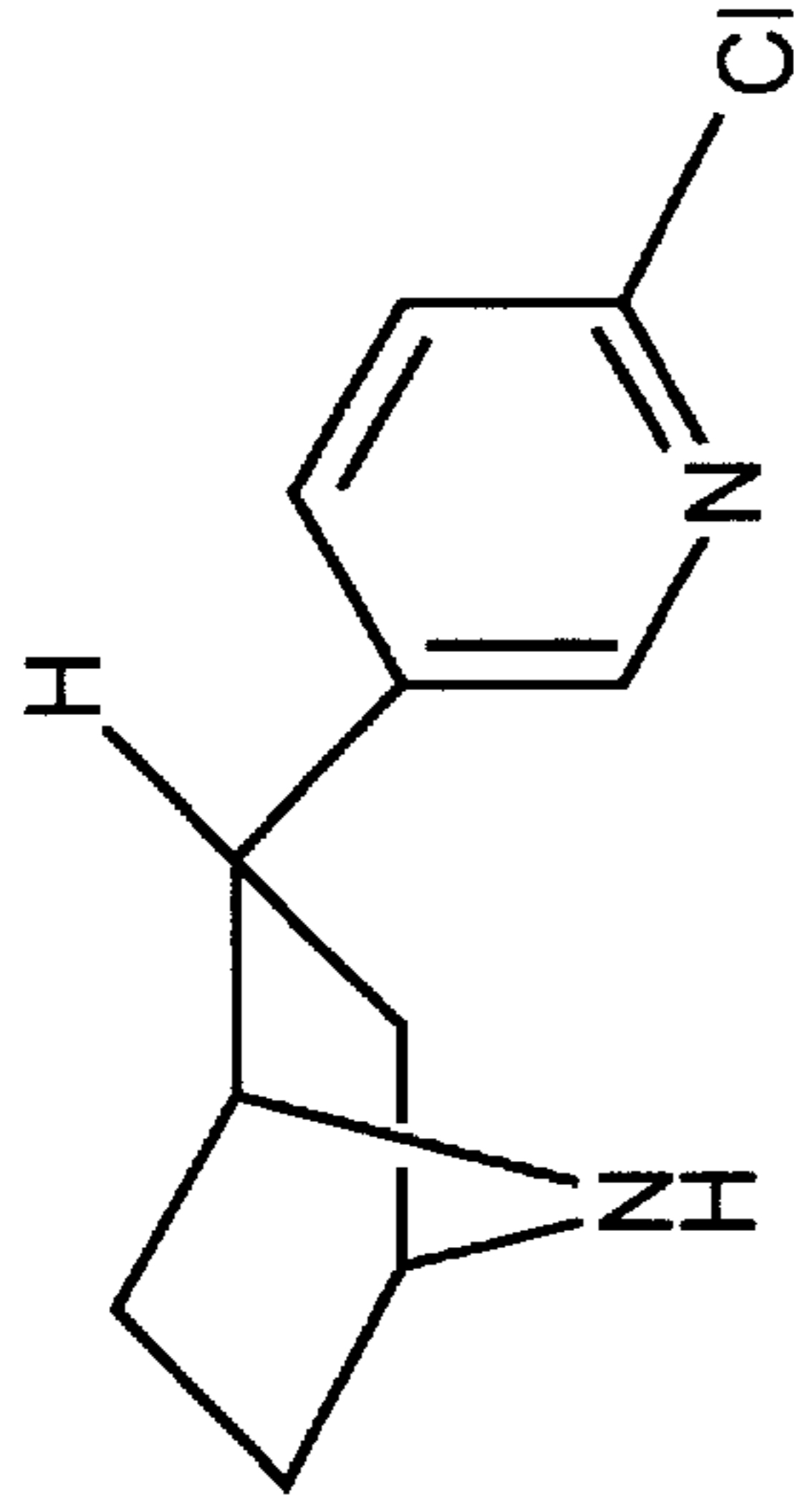
Epibatidine
