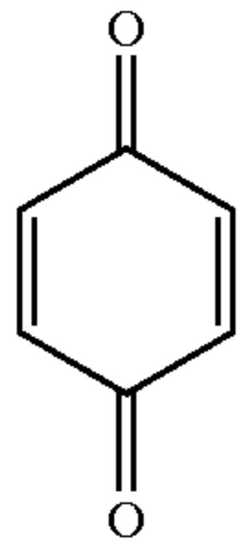
(quinone),
