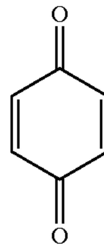
(quinone),
