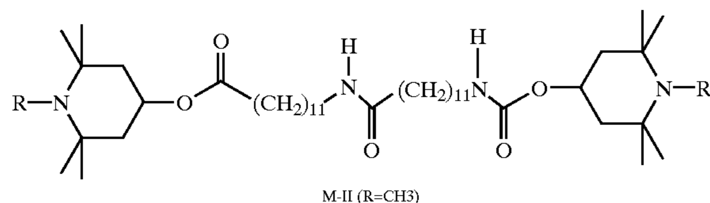
M-II (R=CH 3 )
