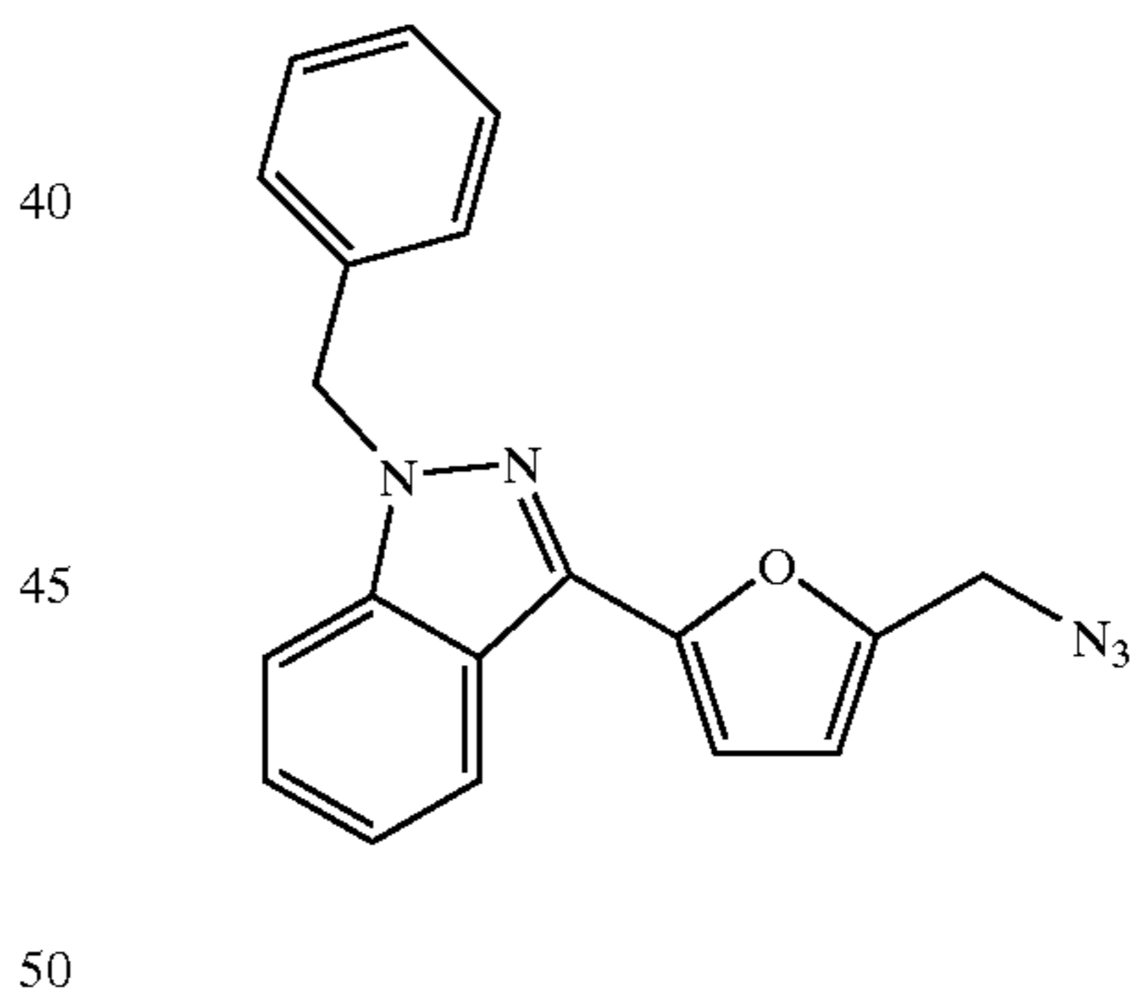
3-(5-Azidomethylfuran-2-yl)-1-benzyl-indazole
