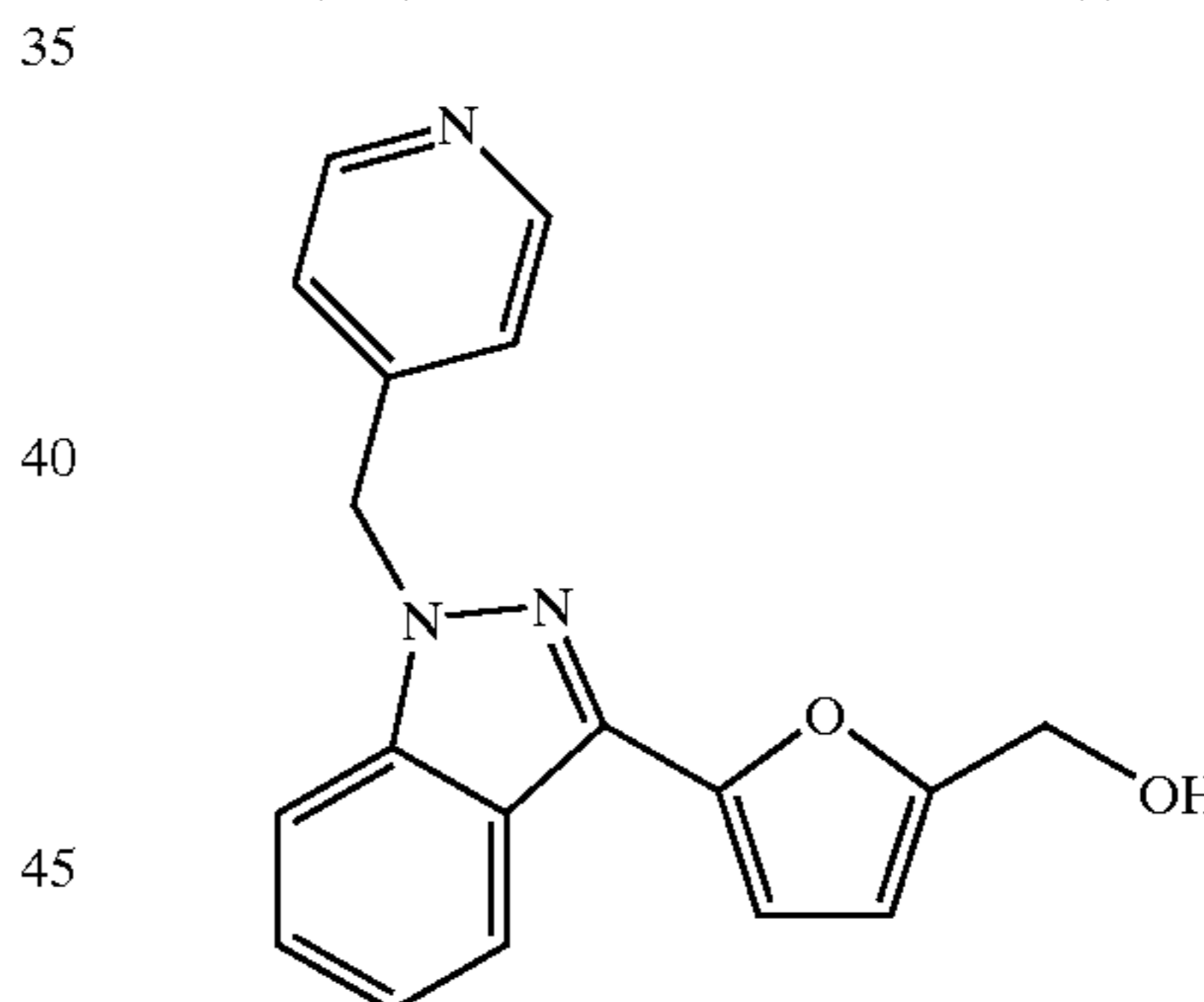
3-(2-(5-Hydroxymethylfuryl))-1-(4-picolyl)indazole
