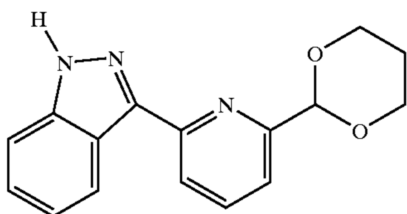
3-(6-(1,3-Dioxan-2-yl)-2-pyridyl)indazole
