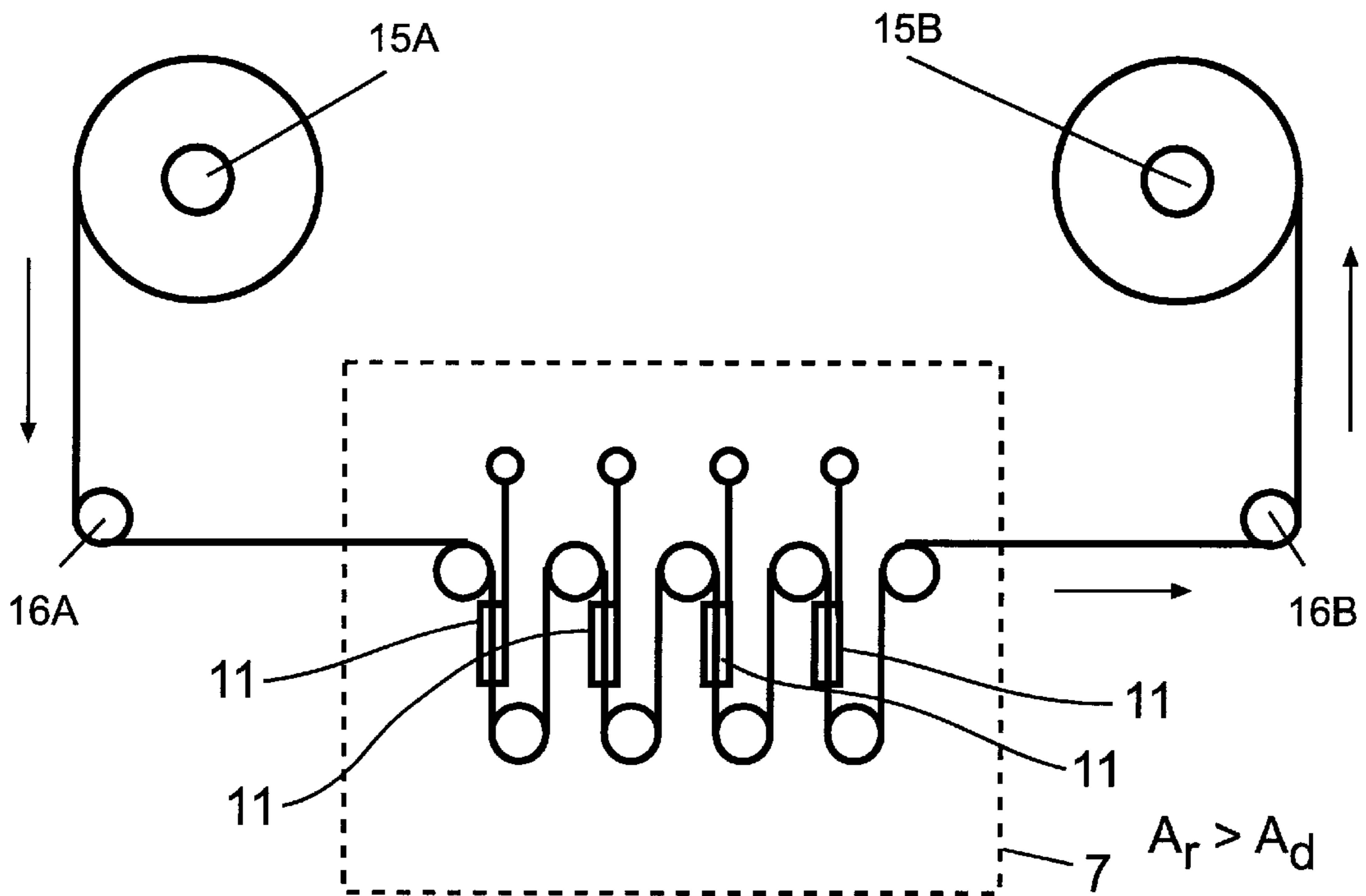
A_r > A_d FIG. 2B2
