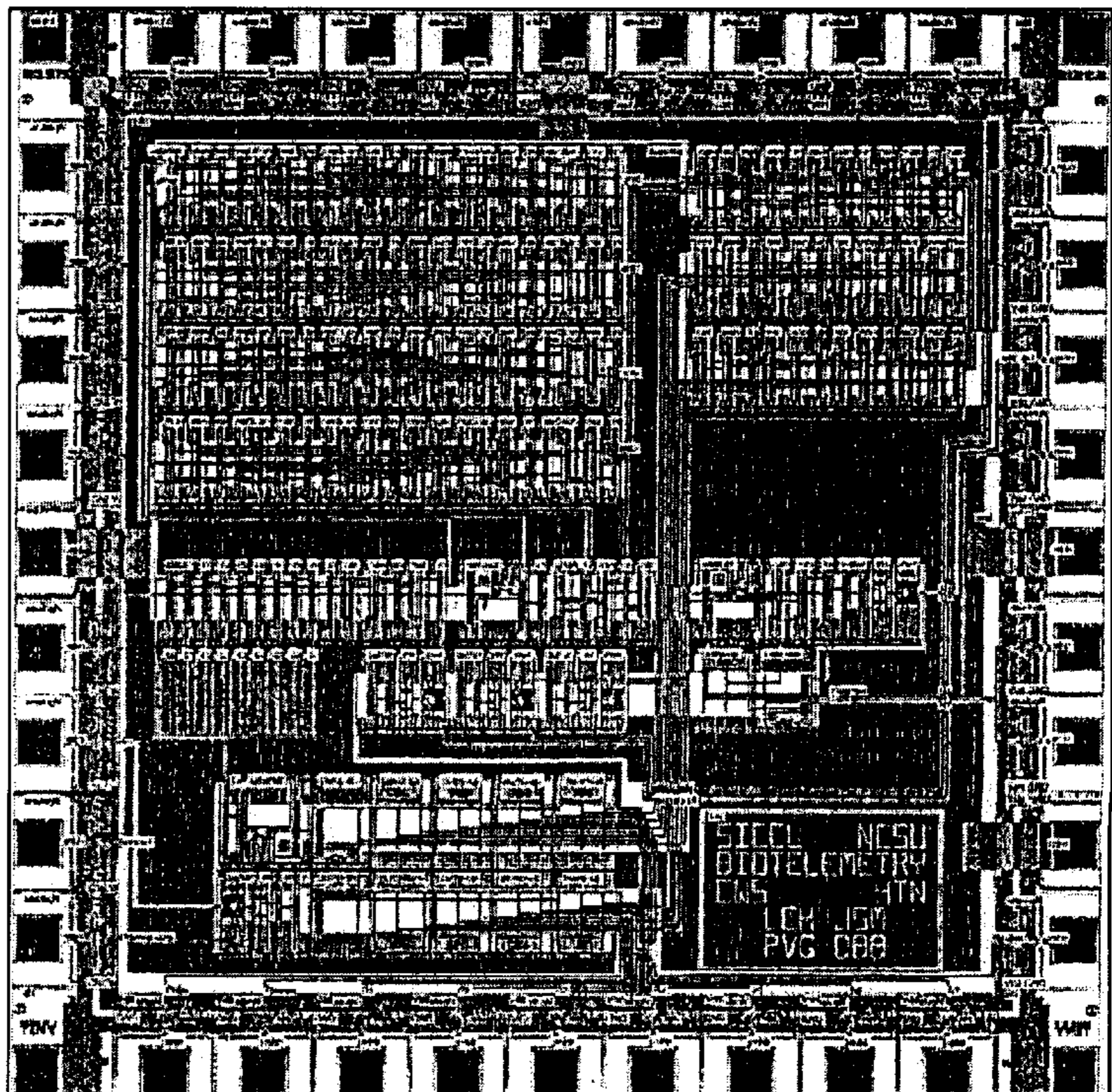
IC LAYOUT
