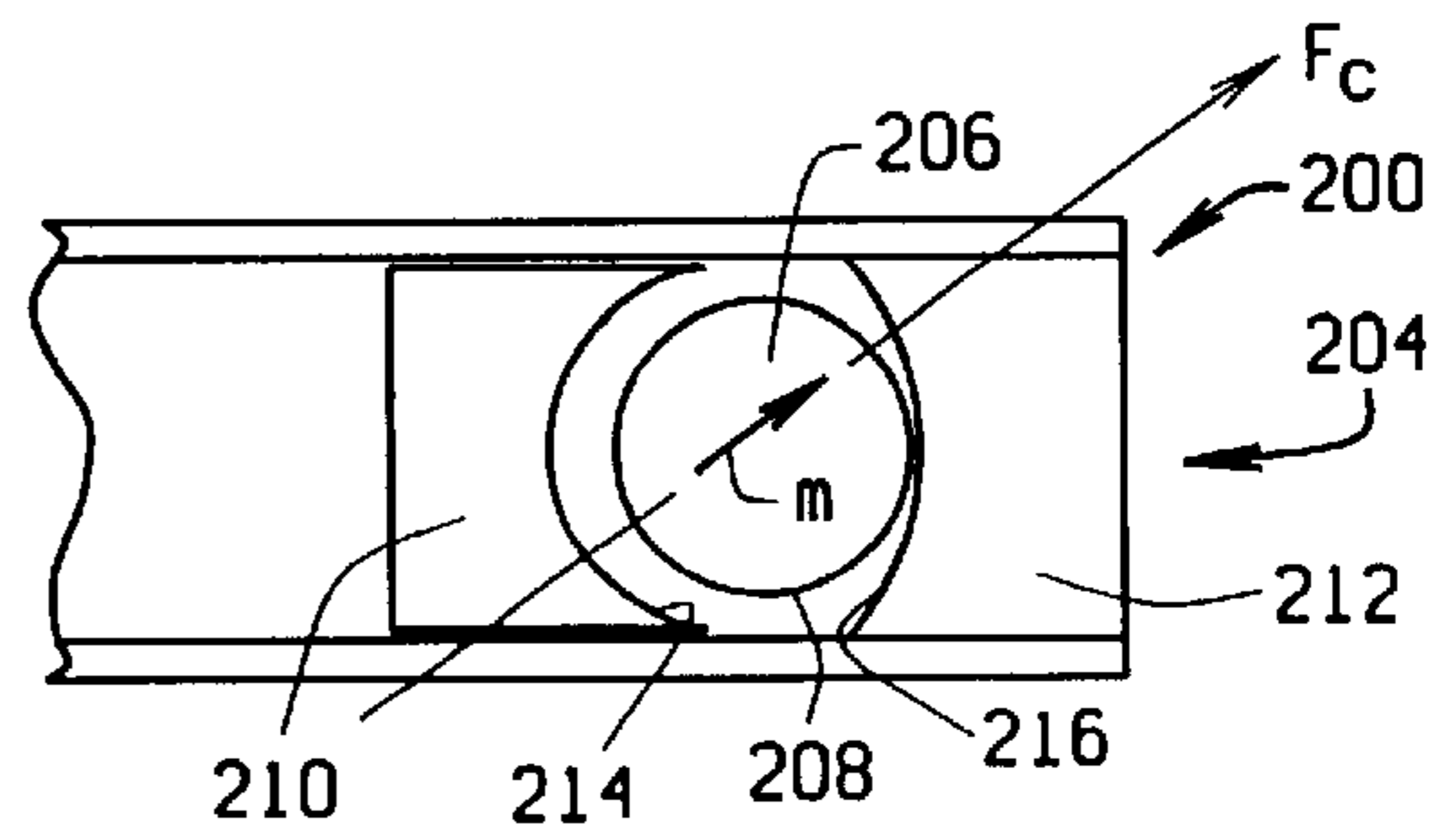
FIG. 15C
