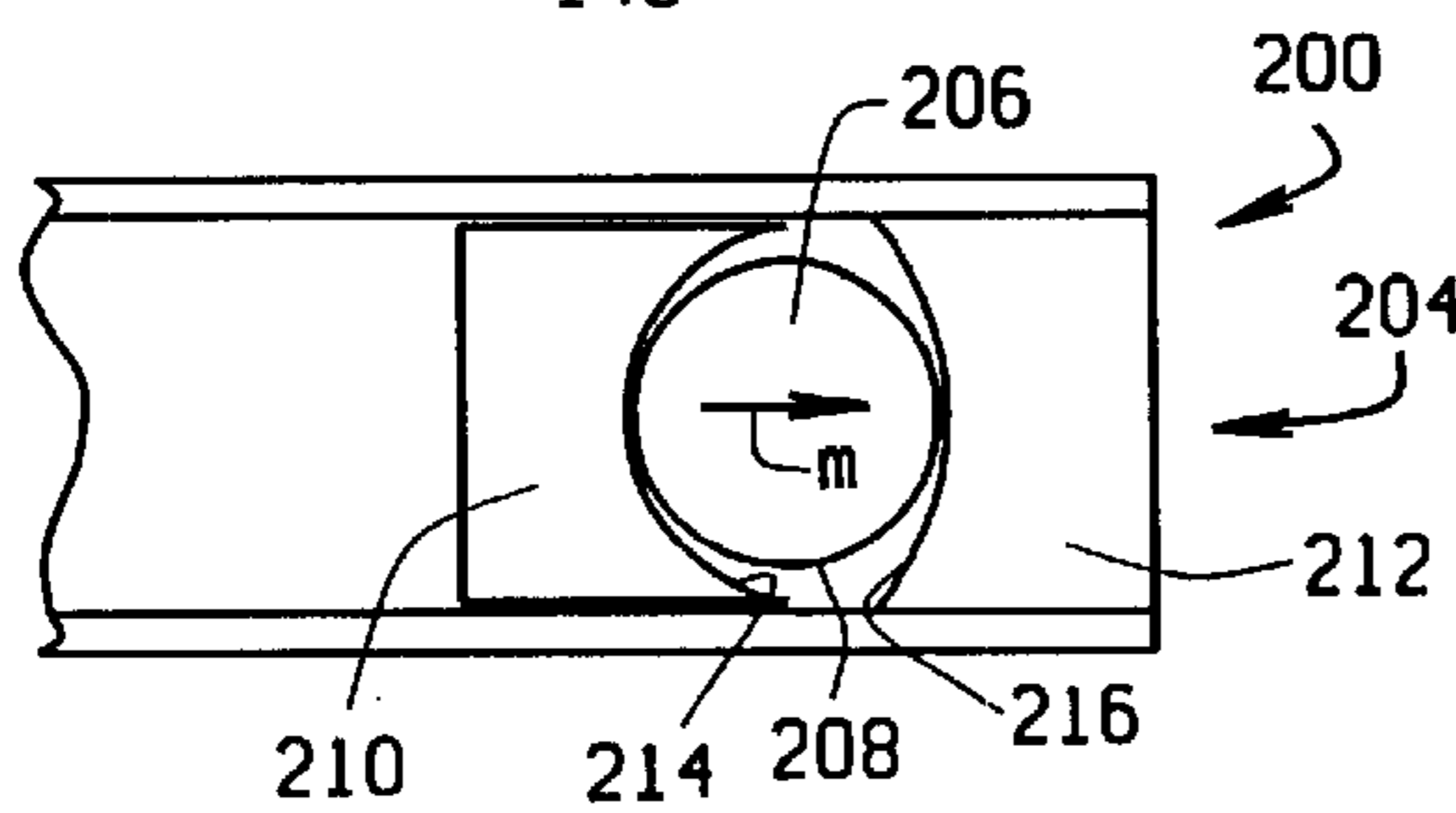
FIG. 15A
