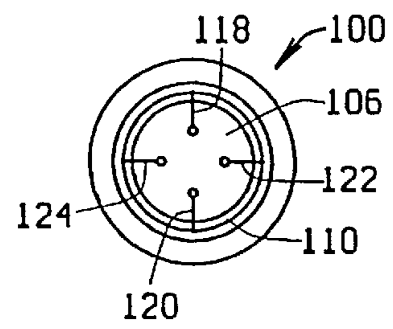
FIG. 11
