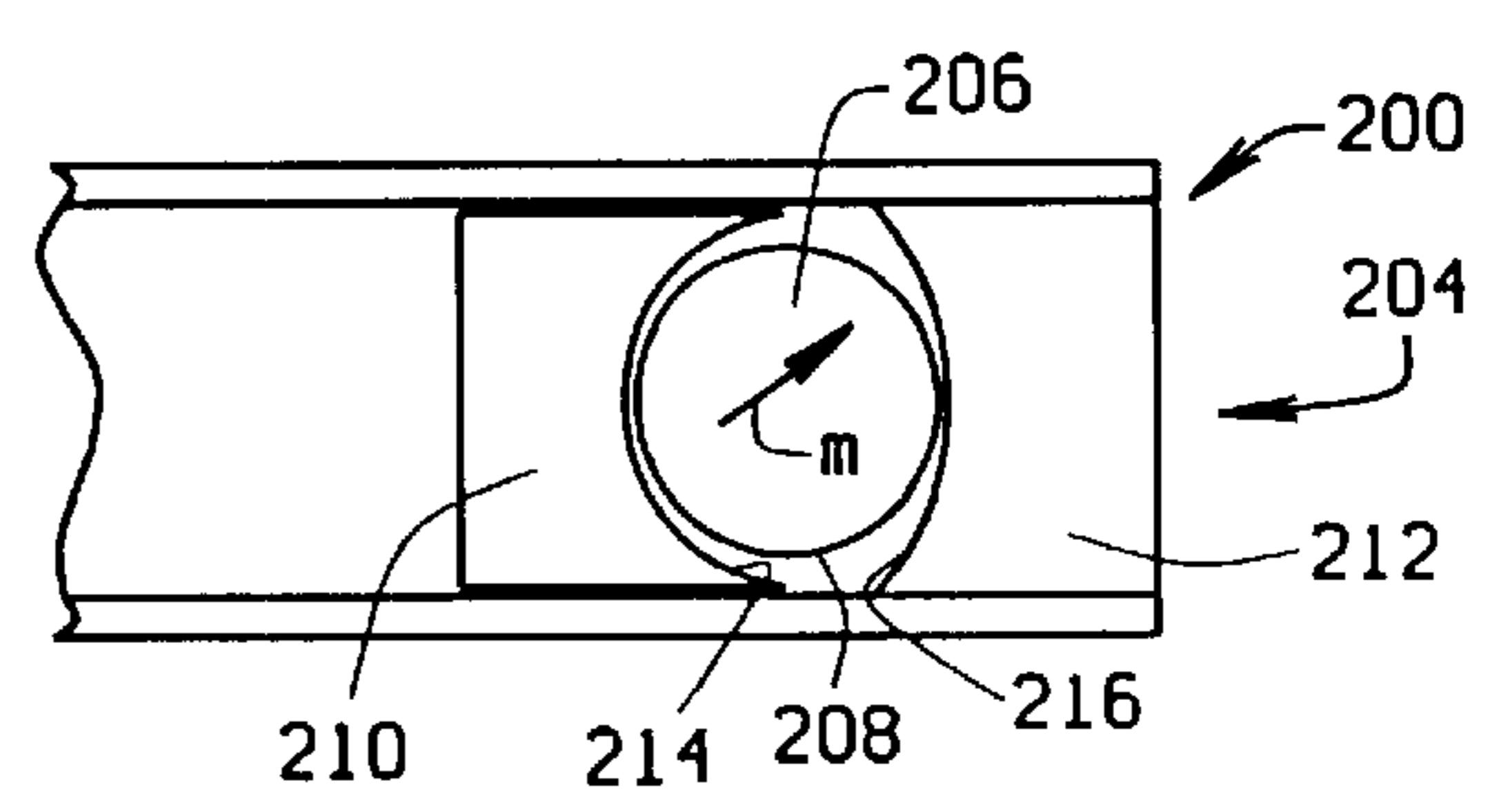
FIG. 15D
