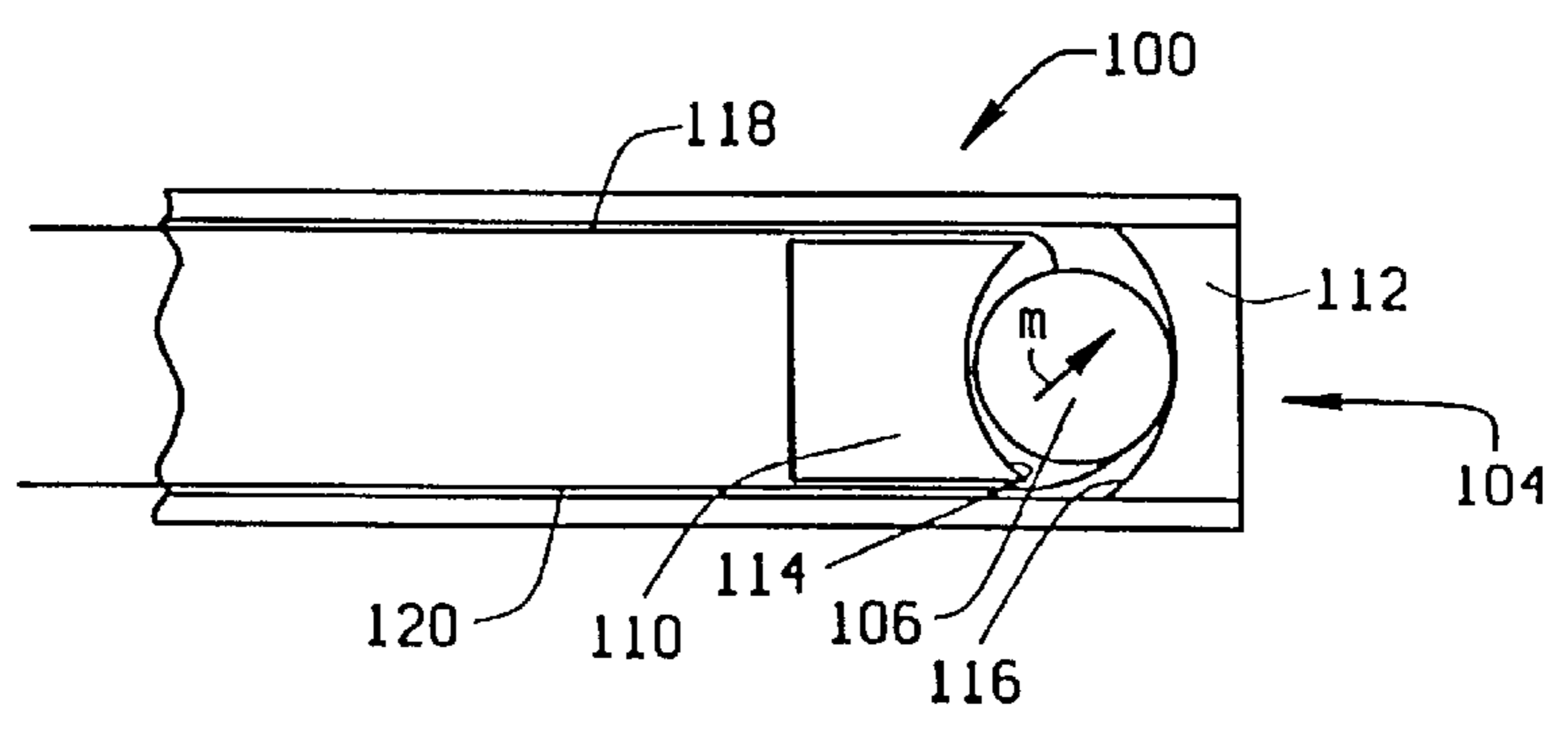
FIG. 10B
