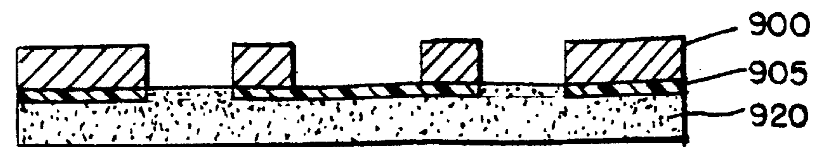
FIG. 9g
