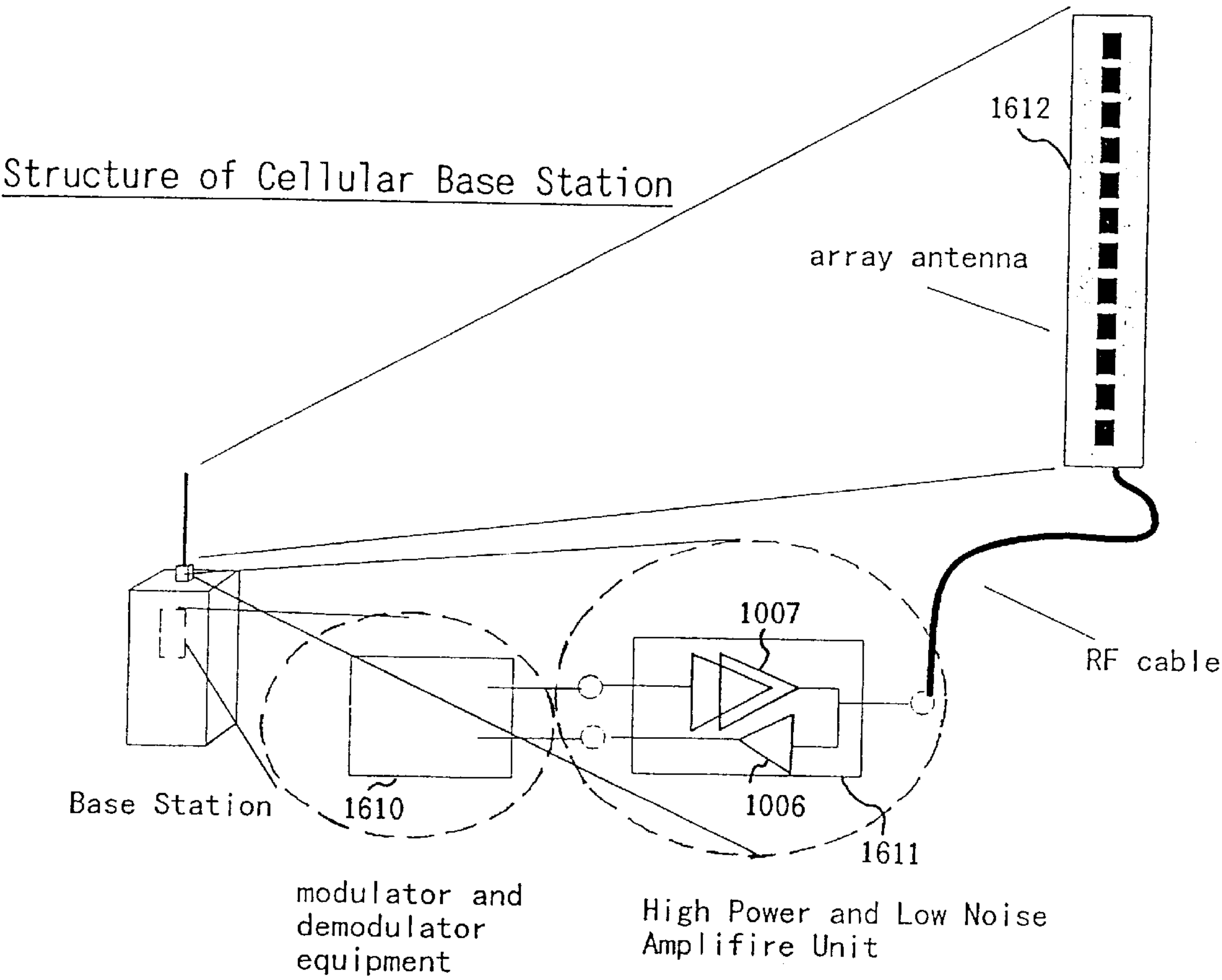
FIG. 16B
