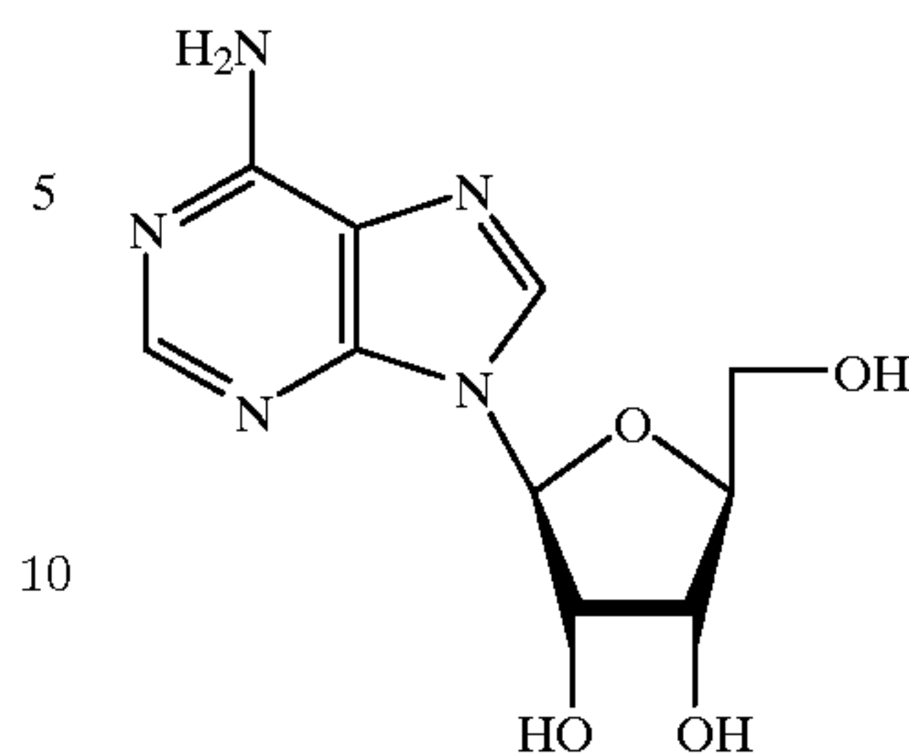
L-adenosine 145
