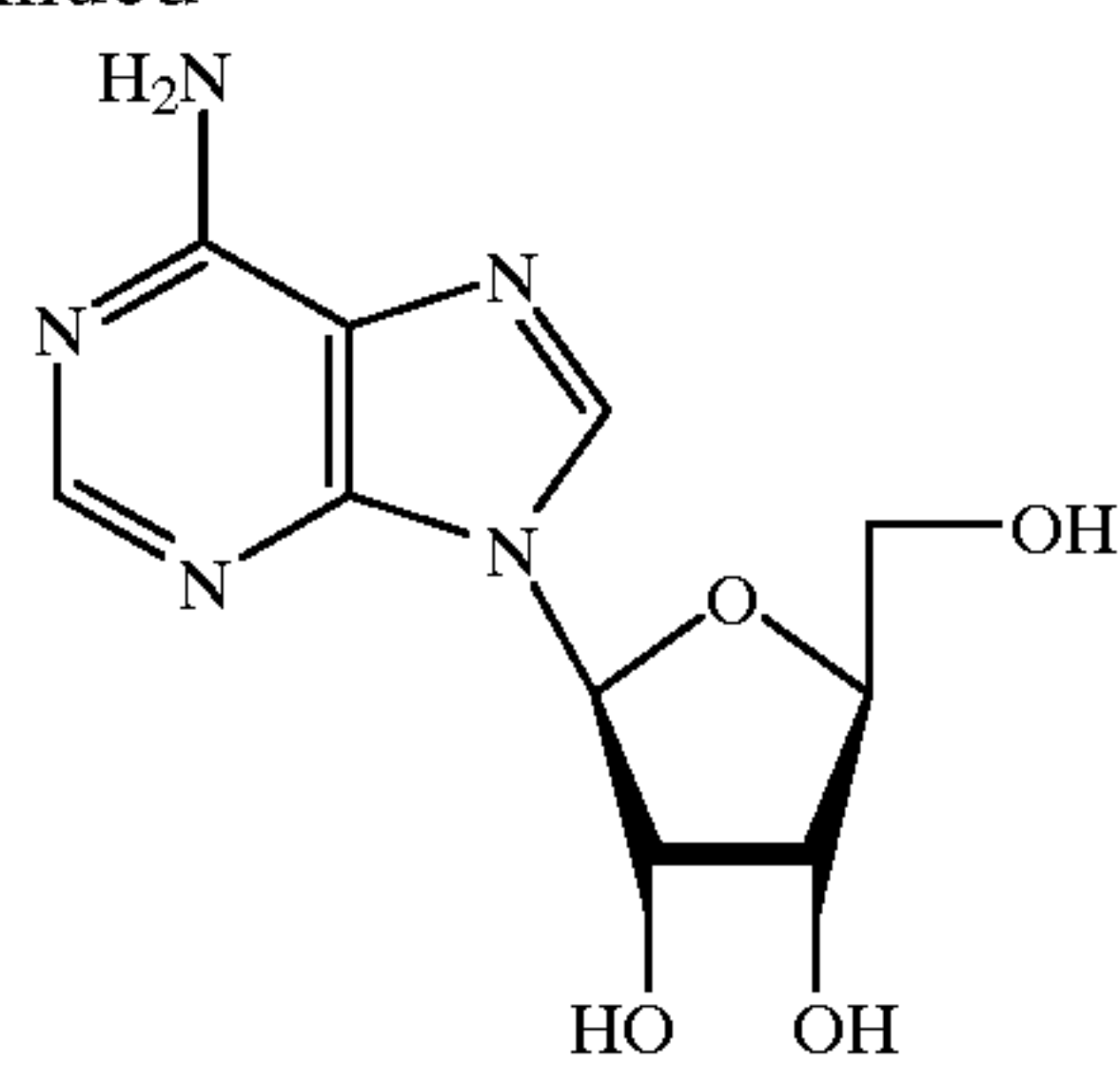
L-adenosine 145
