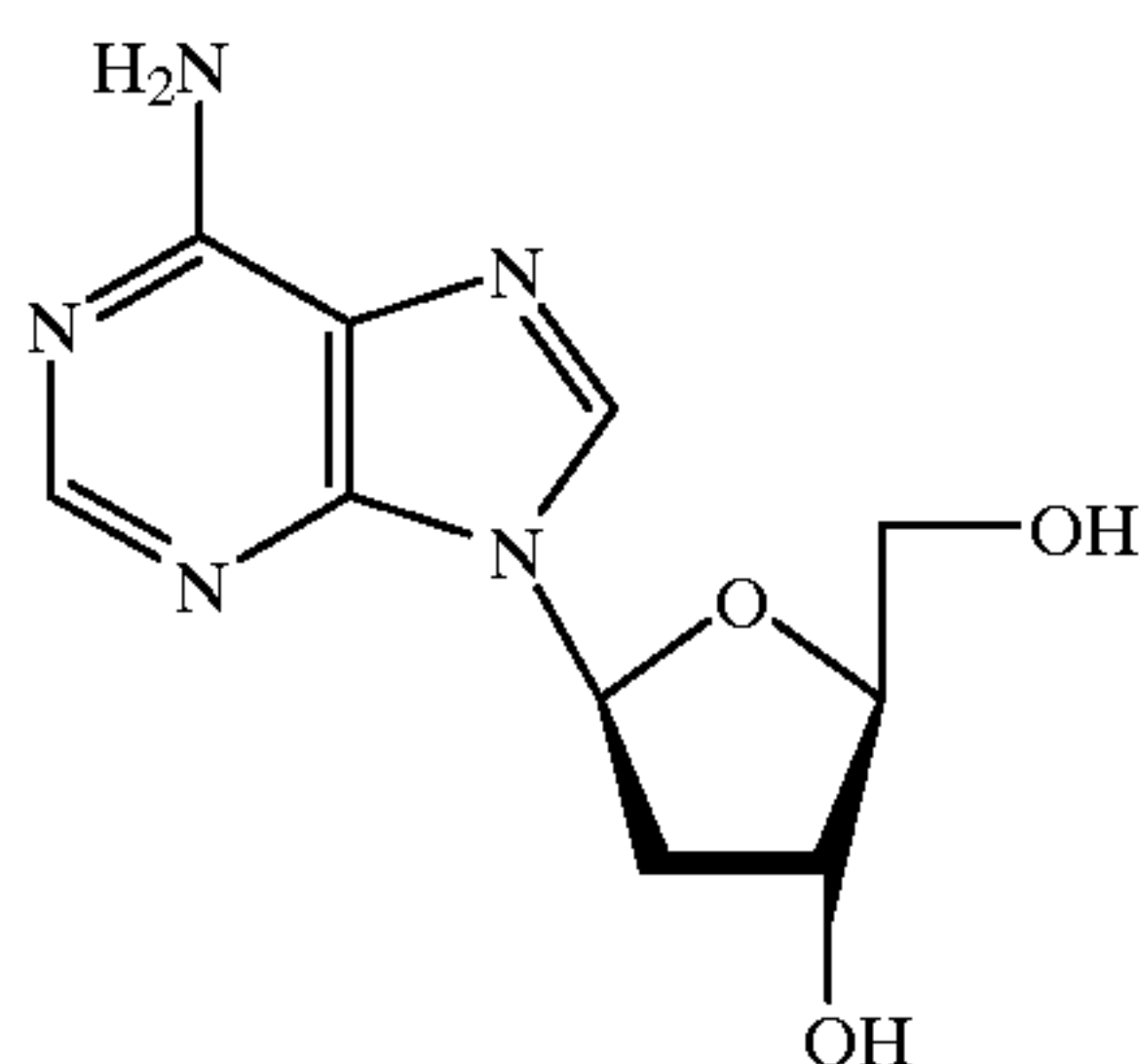
L-deoxyadenosine 149
