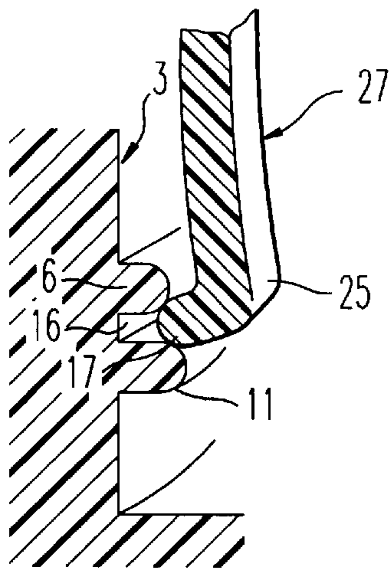
FIG. 5C
