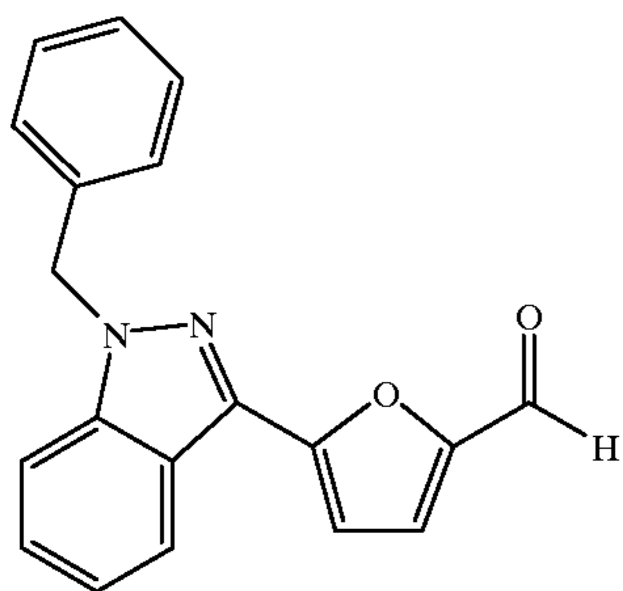
1-Benzyl-3-(5-formylfuran-2-yl)-indazole
