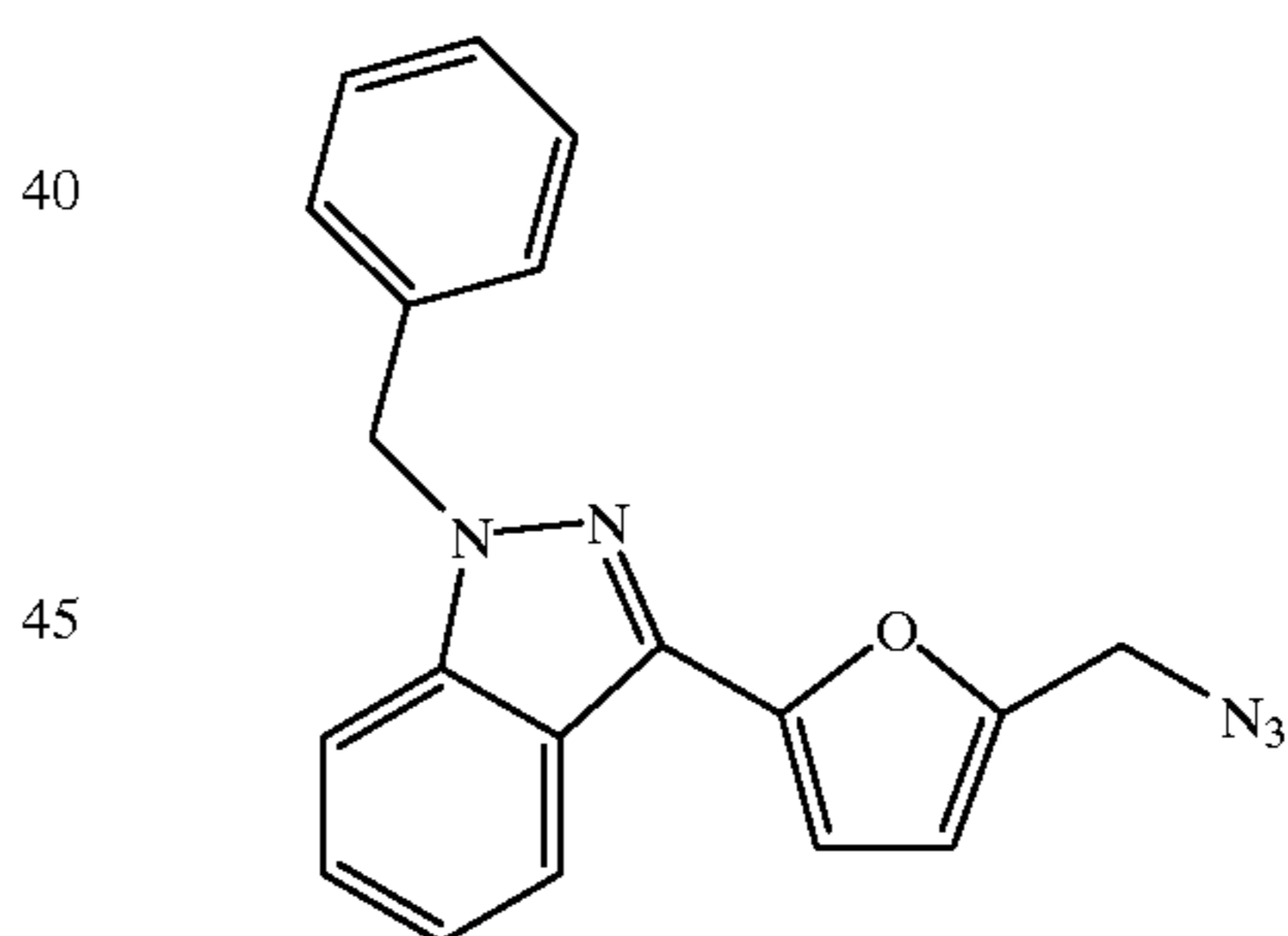
3-(5-Azidomethylfuran-2-yl)-1-benzyl-indazole
