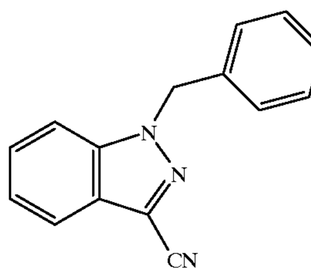
1-Benzyl-3-cyanoindazole
