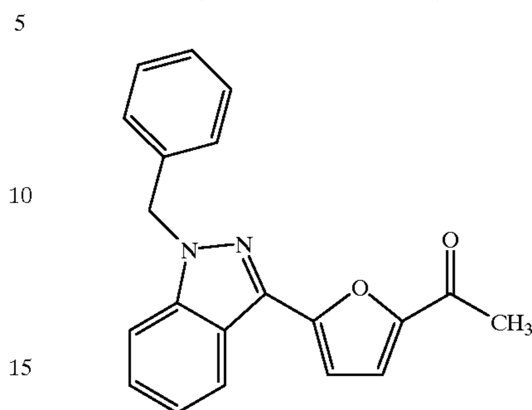
3-(5-Acetylfuran-2-yl)-1-benzyl-indazole
