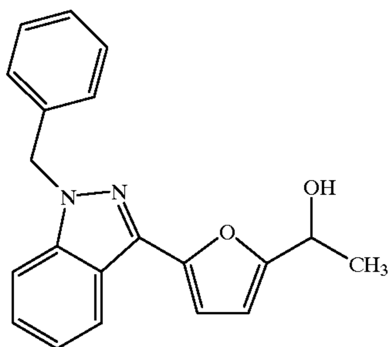
1-[5-(1-Benzylindazol-3-yl)-furan-2-yl]-ethanol
