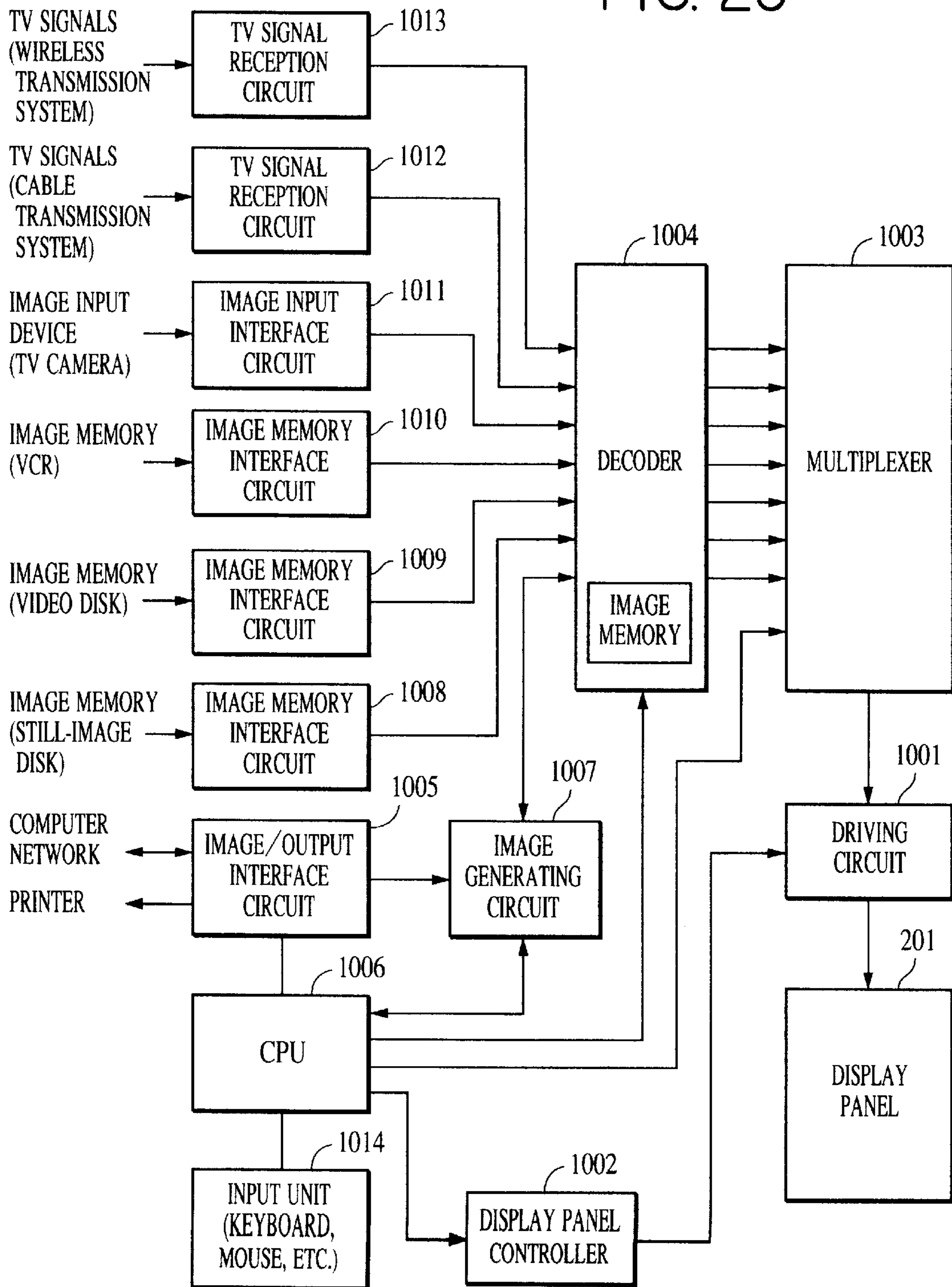
FIG. 25
