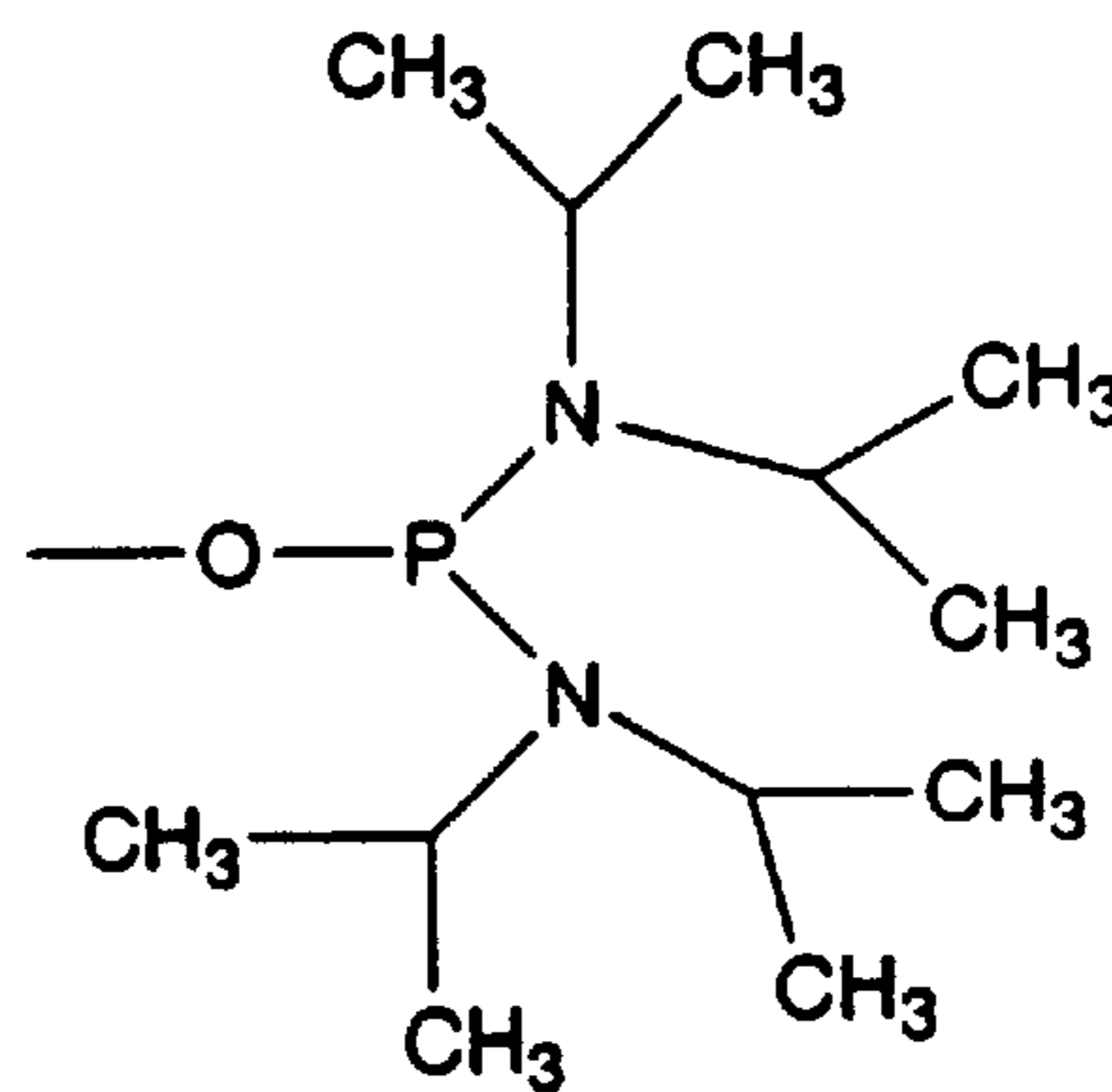
Bis(N,N-diisopropylamino)- phosphine
