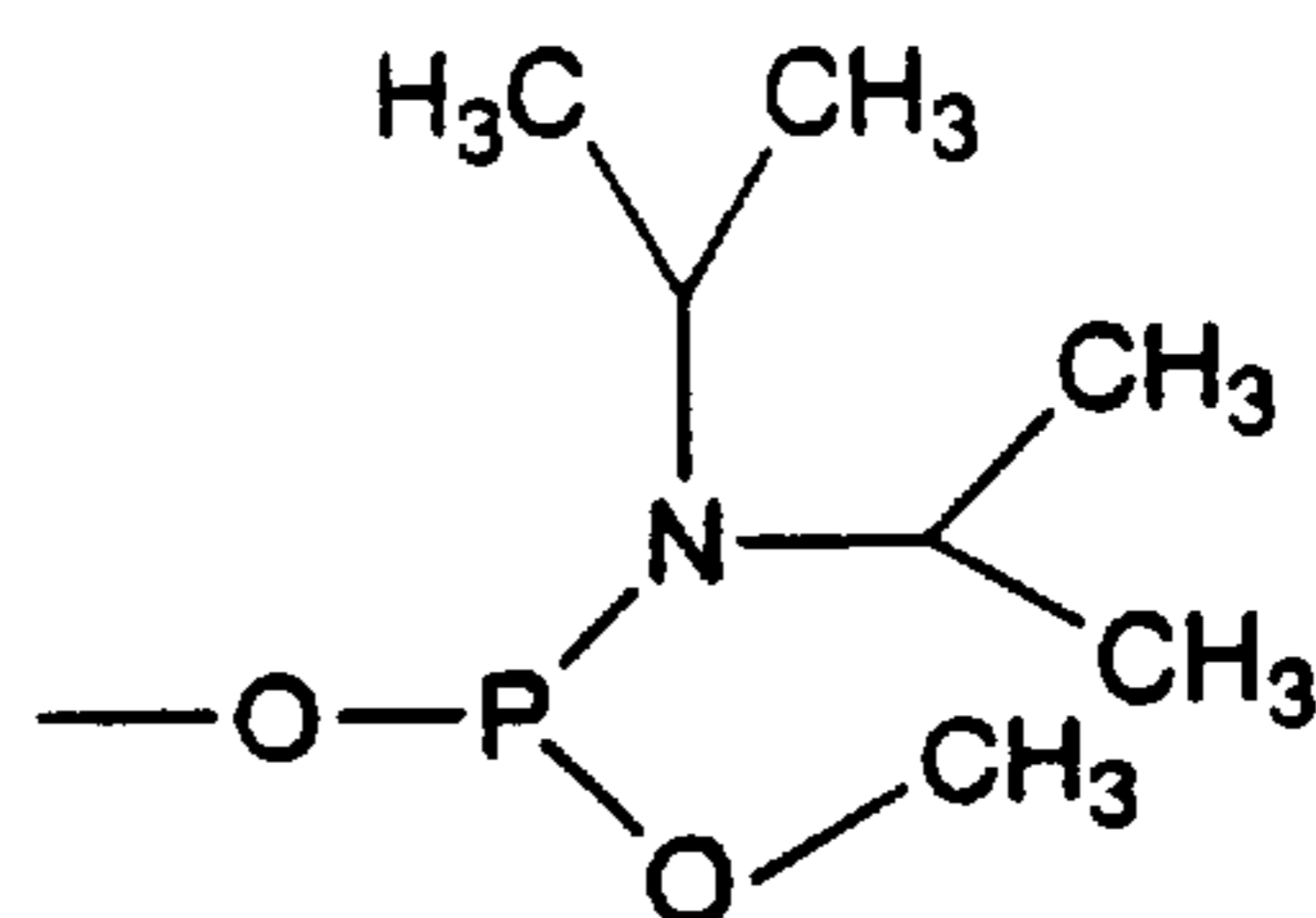
N,N-diisopropylamino-methoxyphosphine
