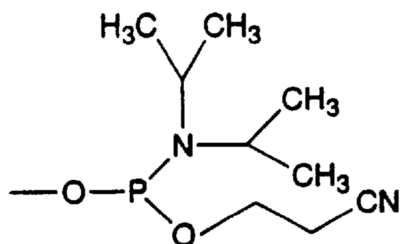
N,N-diisopropylamino-β-cyanoethoxyphosphine
