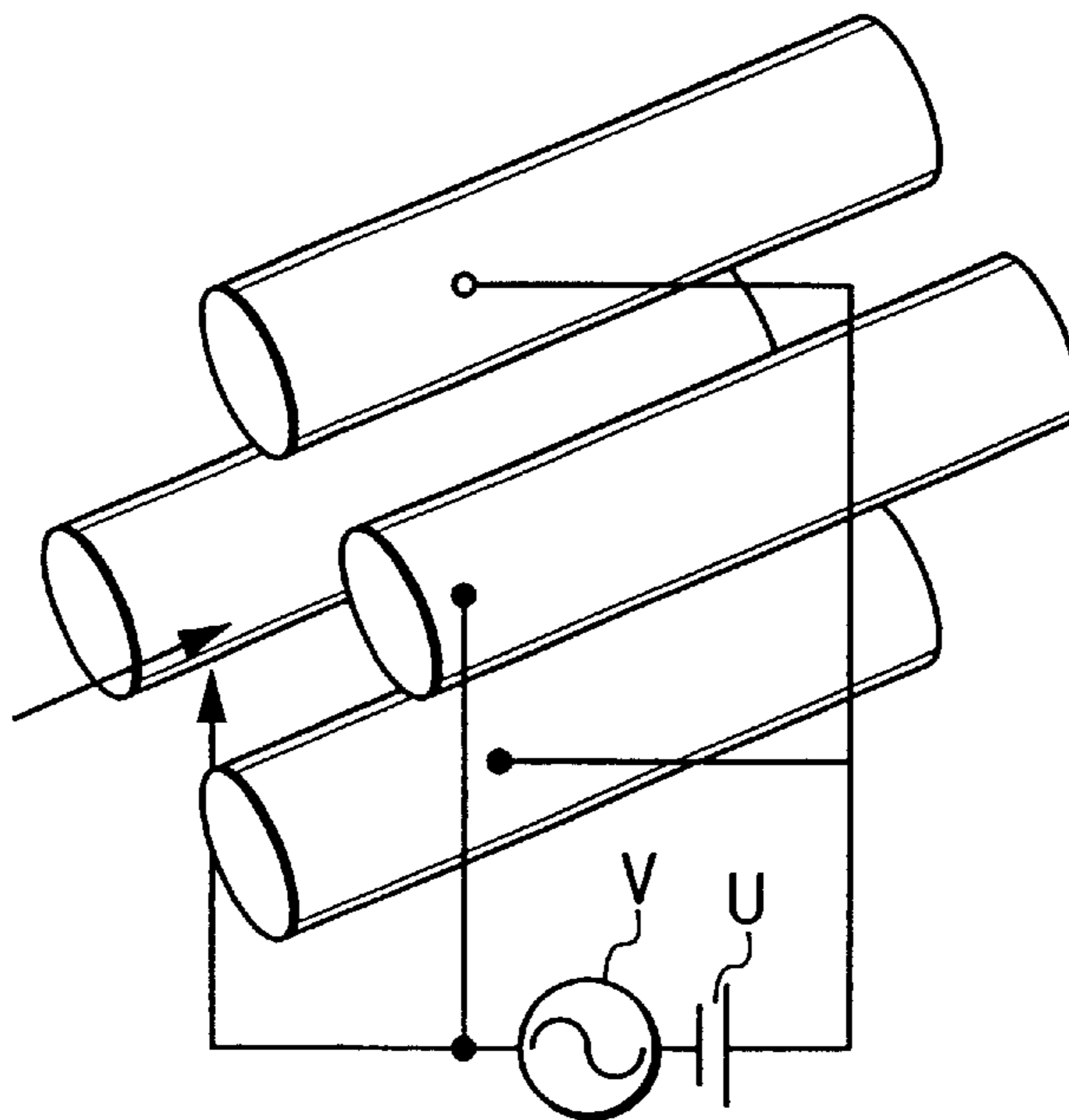
QUADRUPOLE ELECTRODE
